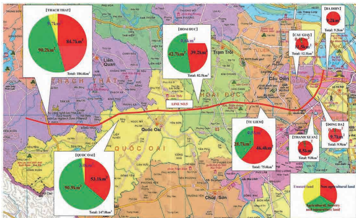
図 1.1.6 ハノイ市の土地利用状況
