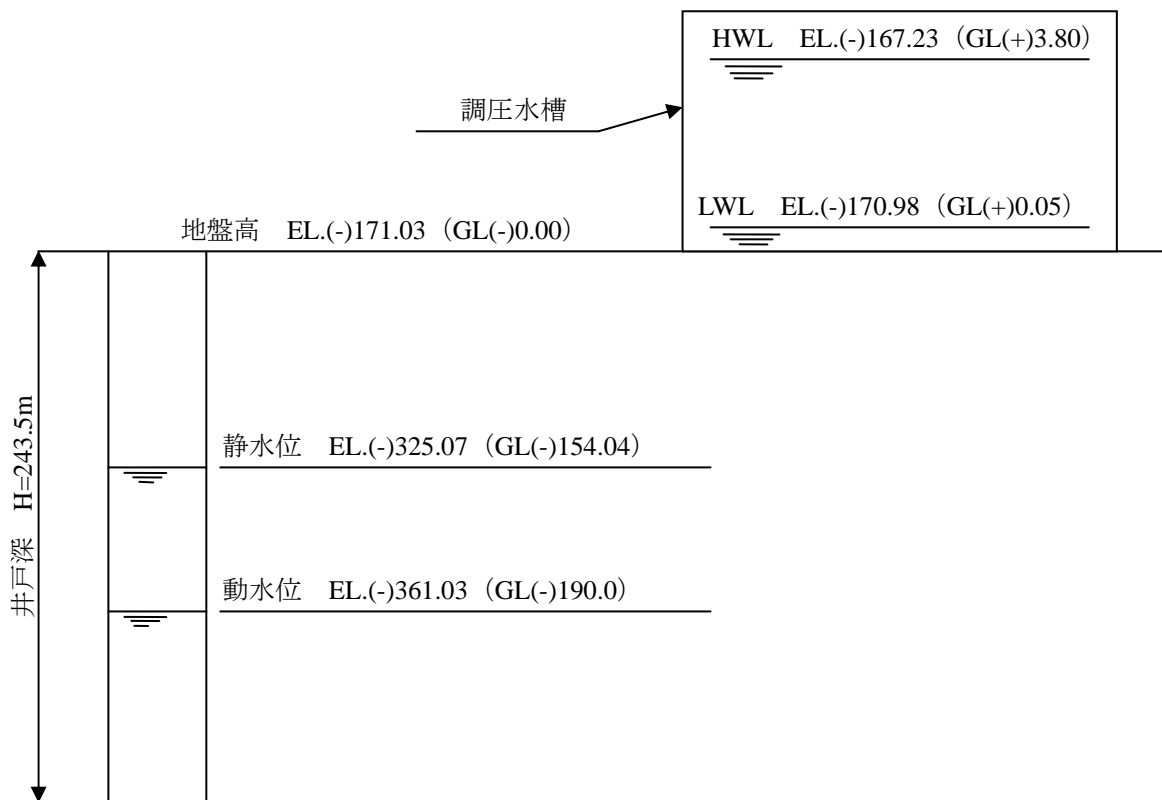
図 3-2-4 ジェリコ No. 1 井戸構造および調圧水槽水位
