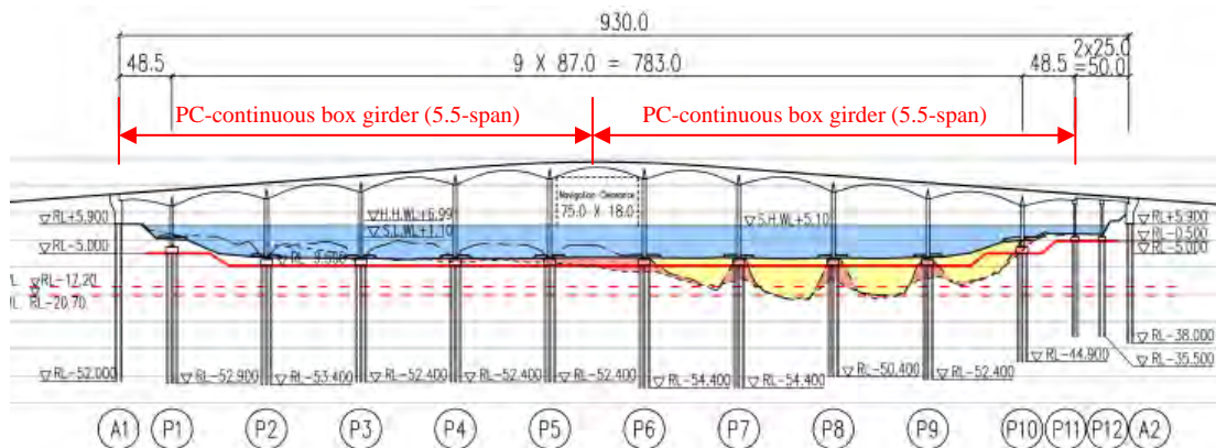
図 8.5.1 メグナ橋の連続化案
