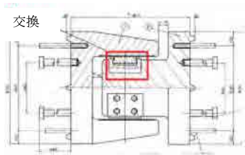
図 8.5.2 ヒンジ構造
