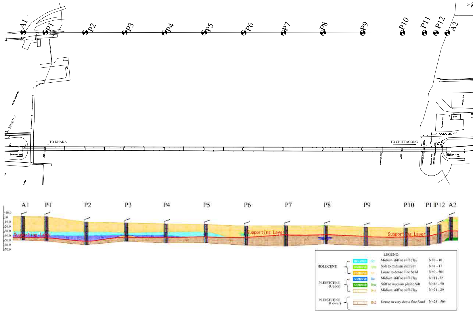
図 2.1.6 メグナ橋ボーリング調査位置および地質縦断面図
