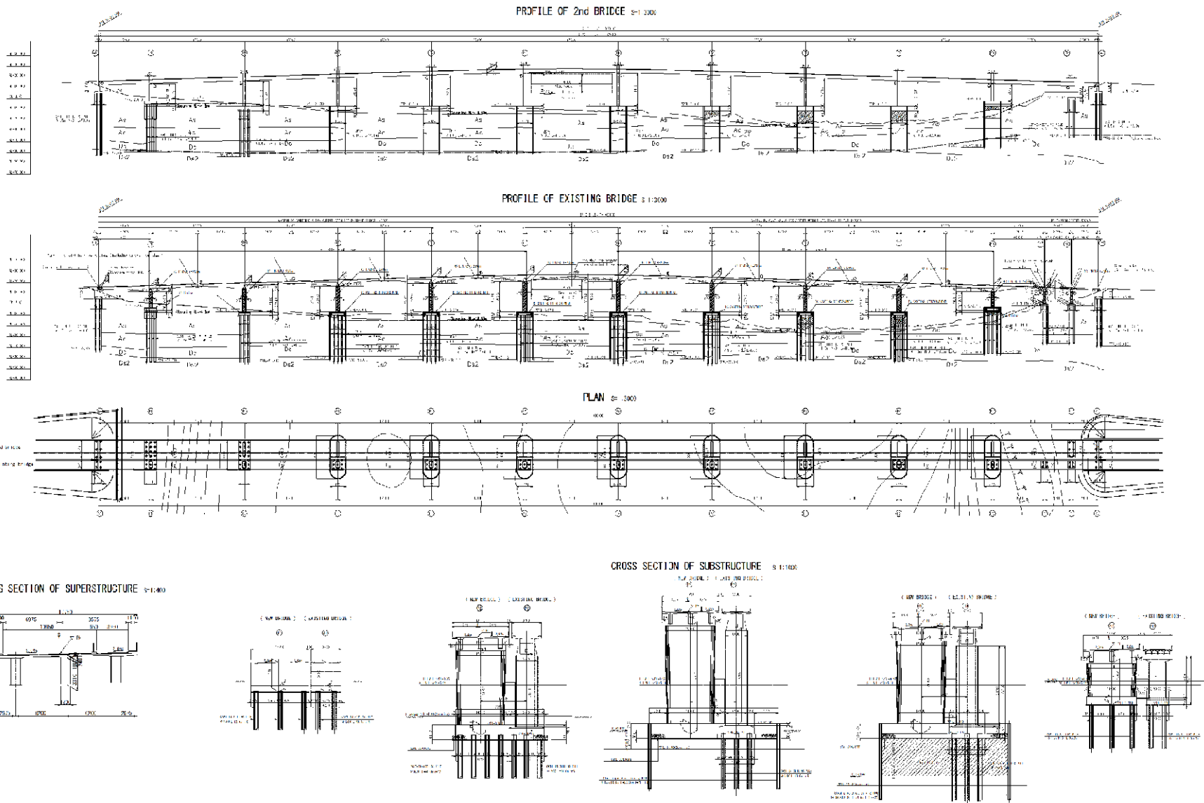
図 5.2.1 橋梁一般図 (第2メグナ橋)
