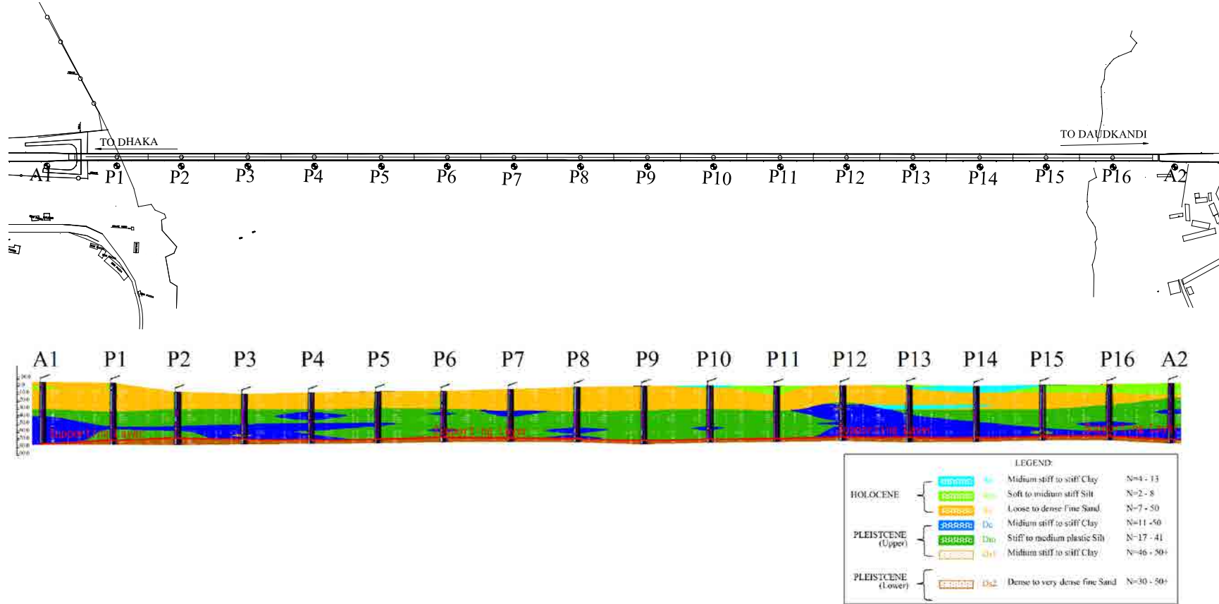
図 2.1.7 グムティ橋ボーリング調査位置および地質縦断図
