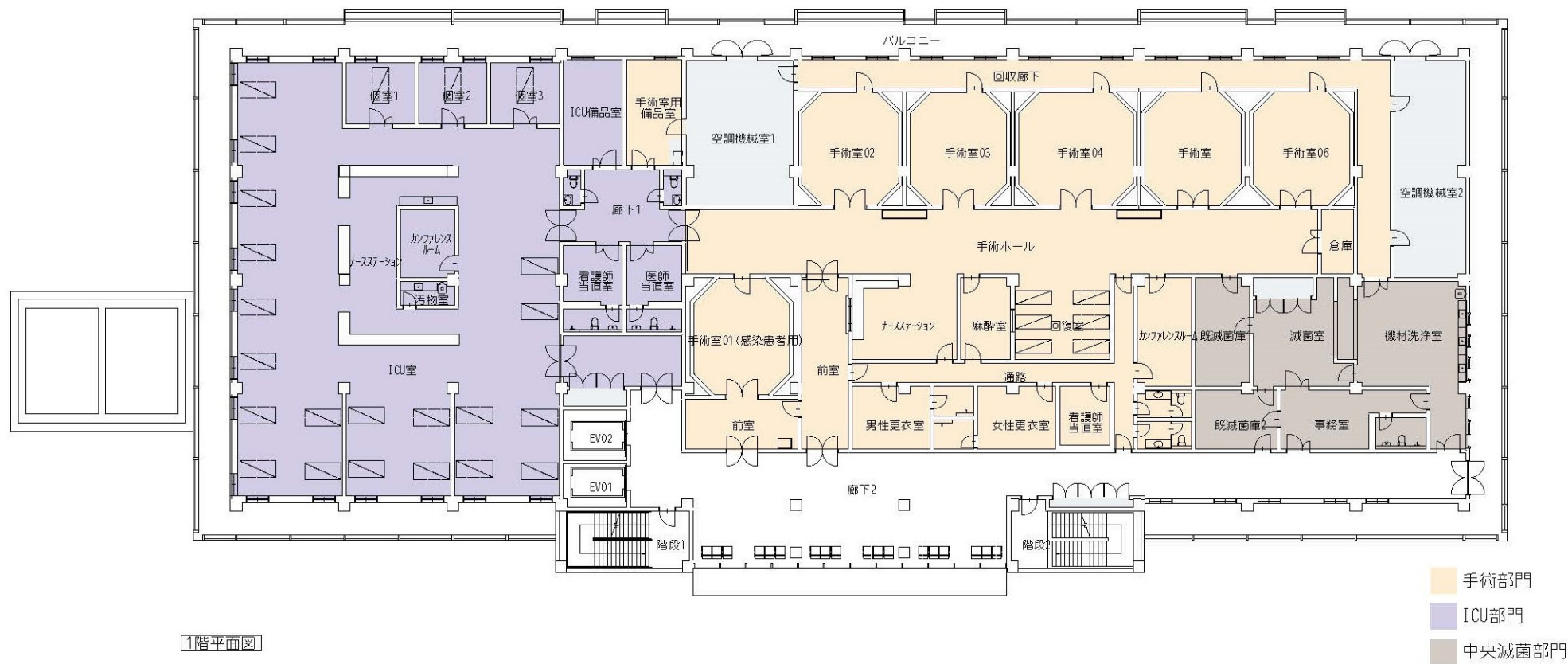
図 3-3 1 階平面図
