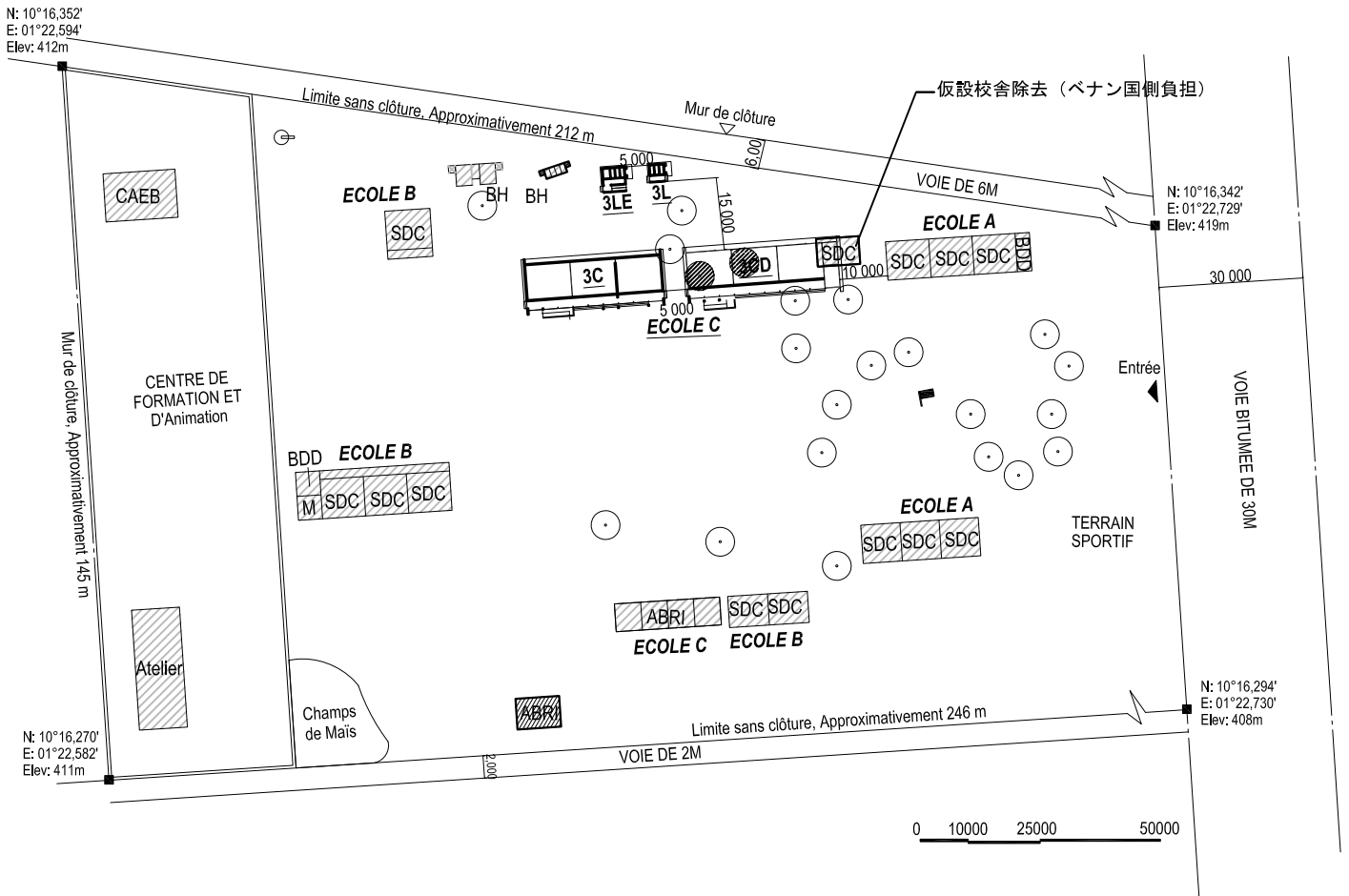
配置図 1 : 1500
