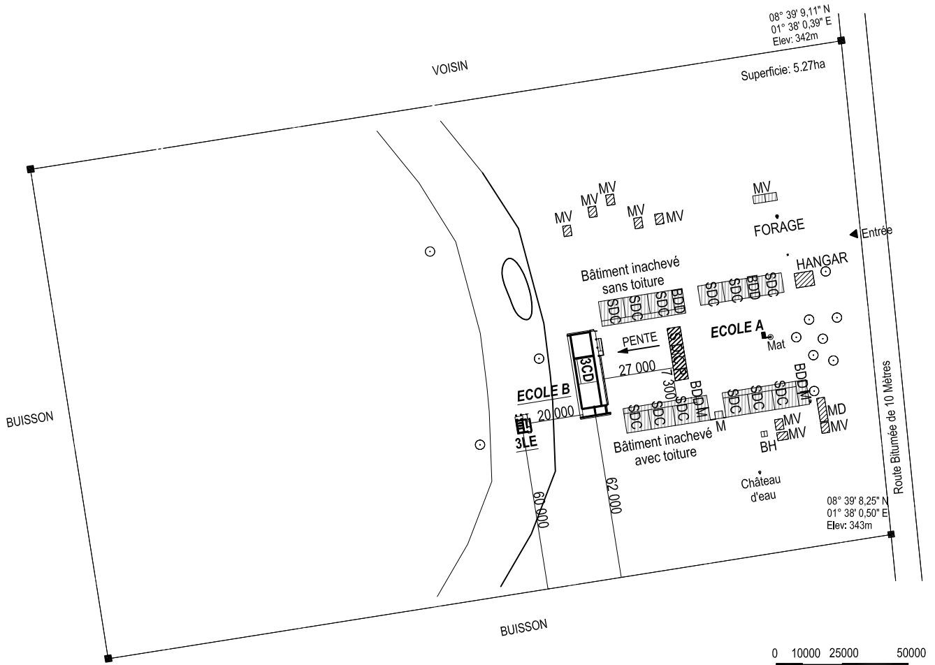
配置図 1 : 2000
