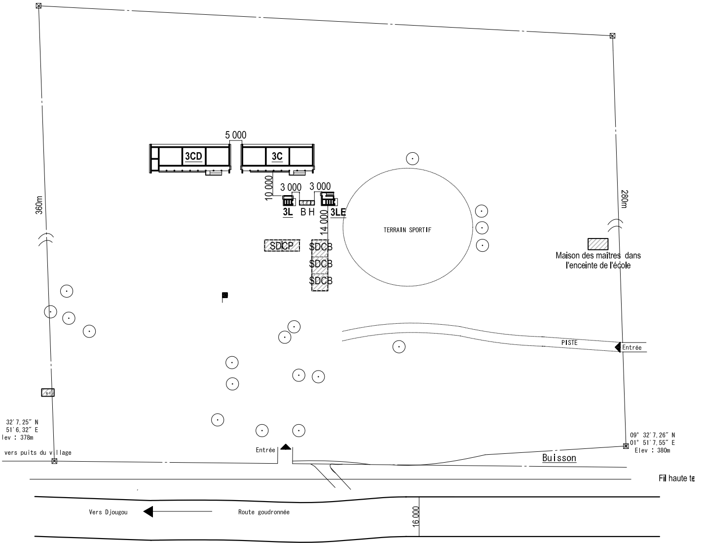
配置図 1 : 1500
