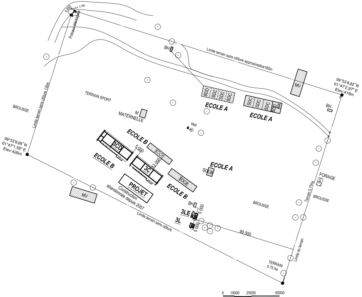
配置図 1 : 2000
