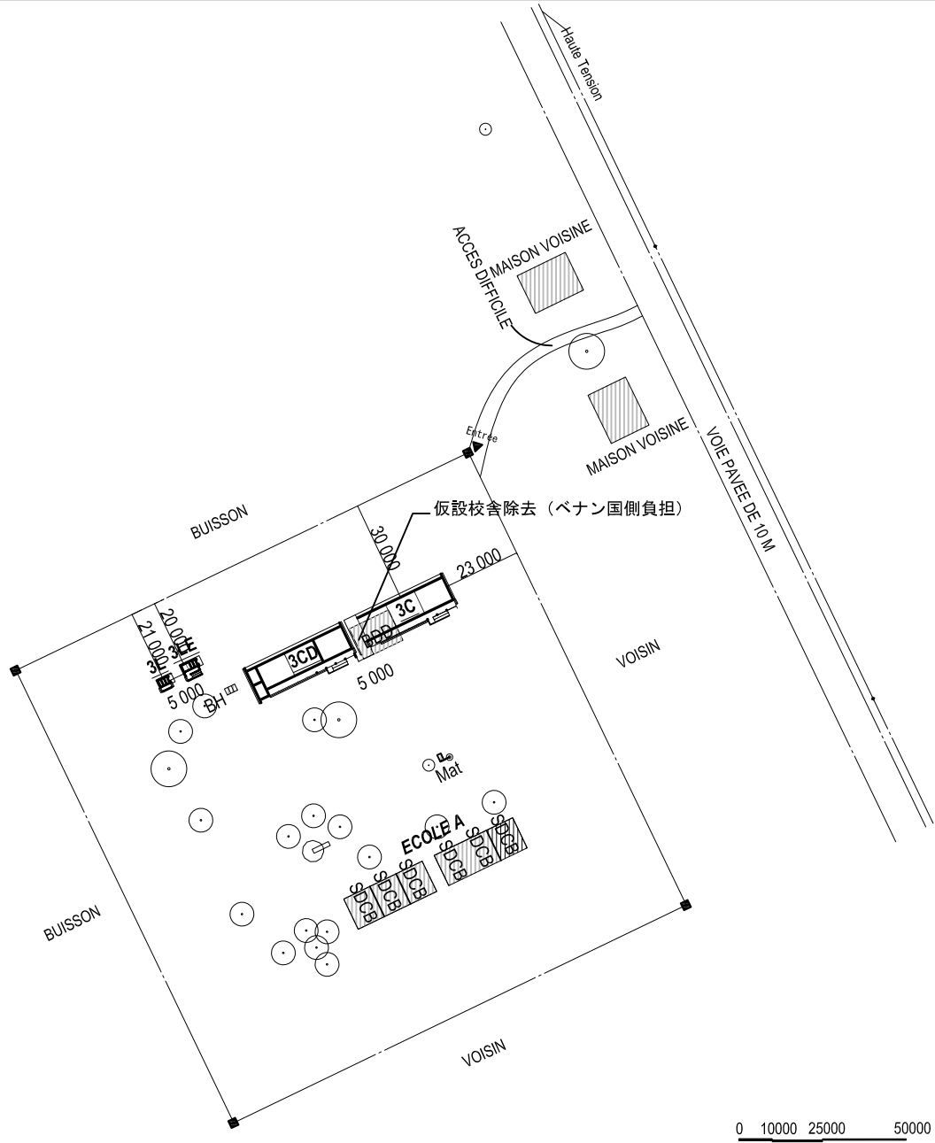
配置図 1 : 1500
