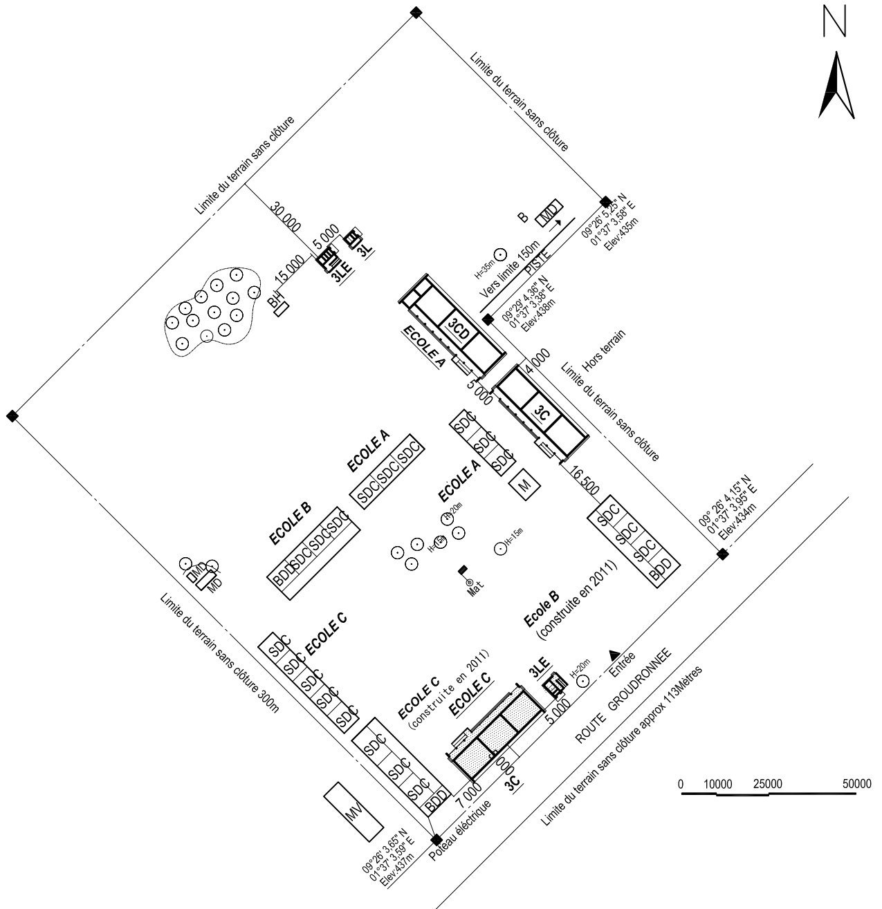
配置図 1 : 1500
