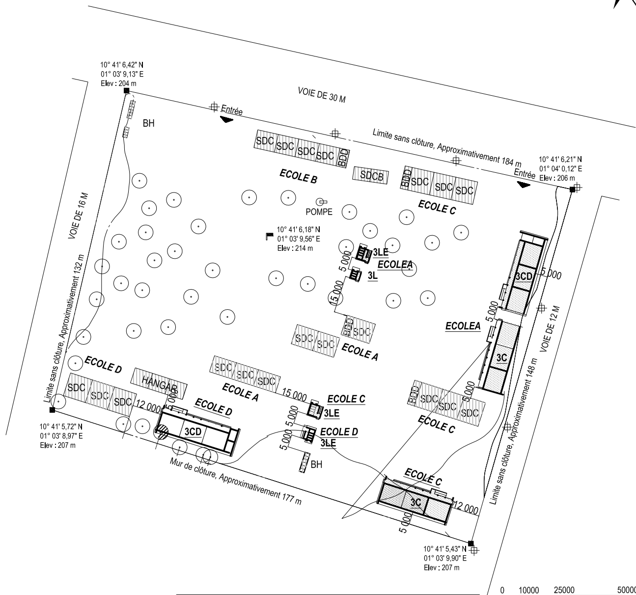
配置図
