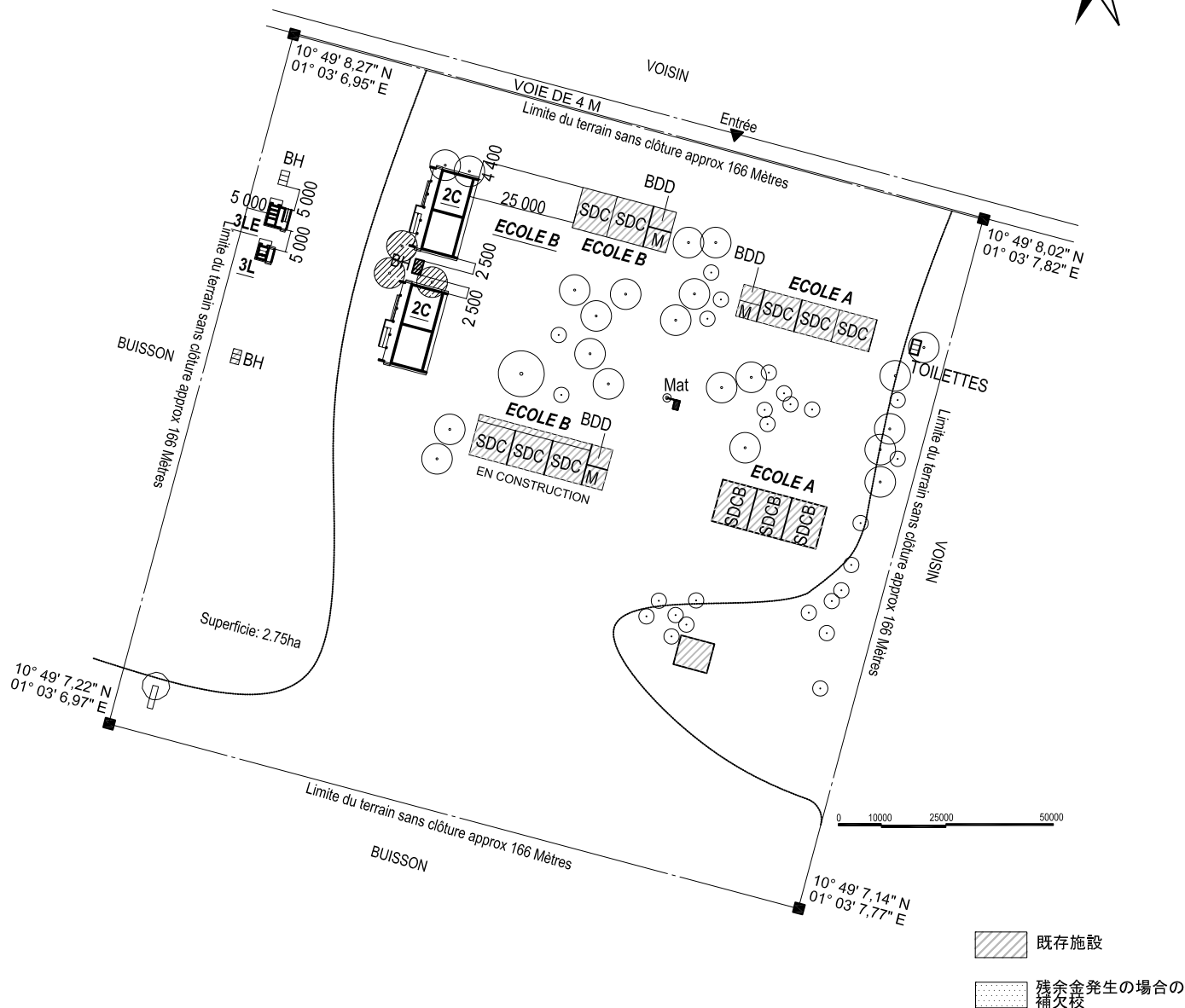
配置図
