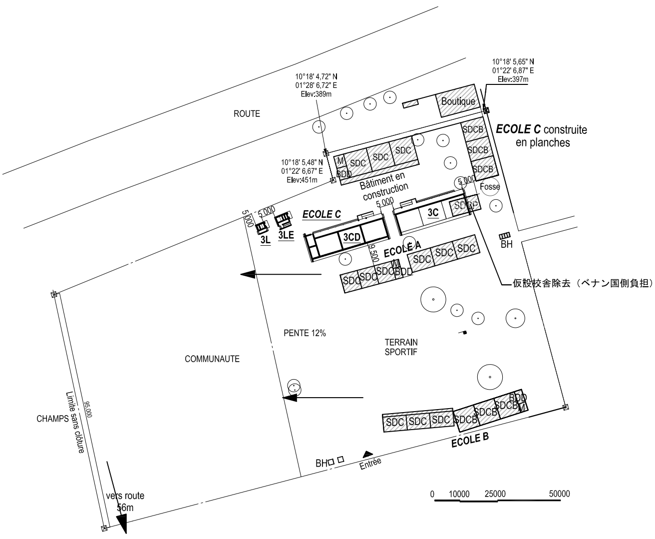
配置図 1 : 1500
