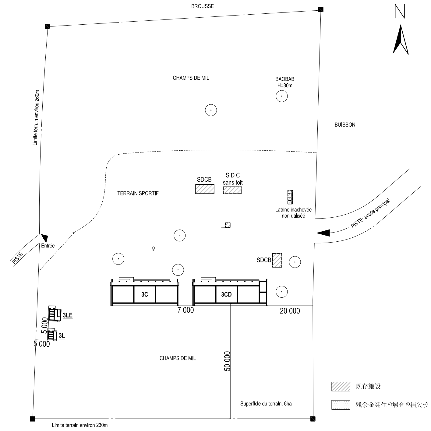
配置図 1 : 1000
