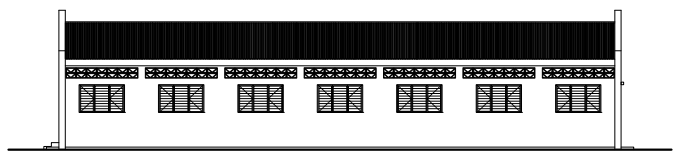
背面立面図
