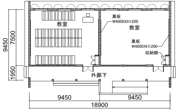
平面図
