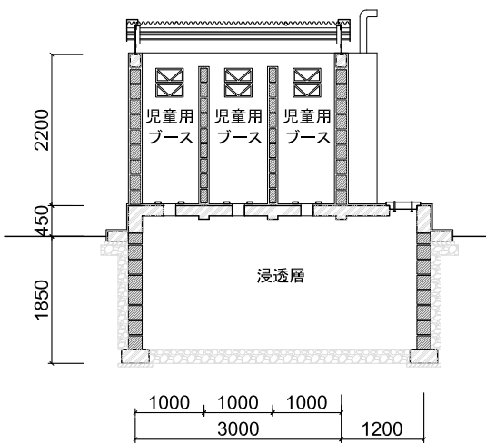
断面図
