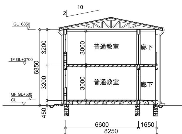
断面図
