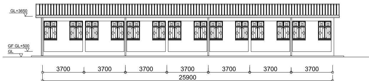
立面図
