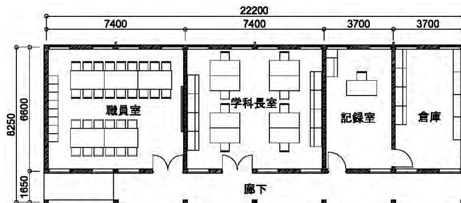
図 3-10 管理棟 B 平面図
