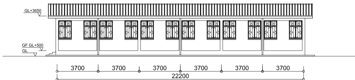
立面図
