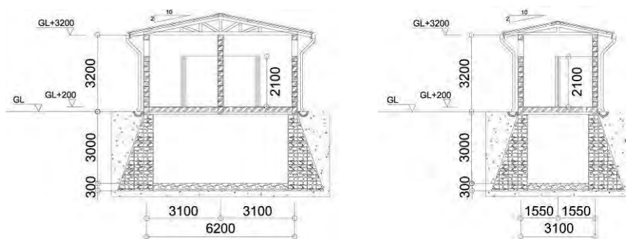
図 3-15 トイレ棟断面図
