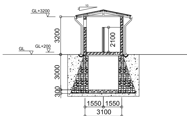
断面図
