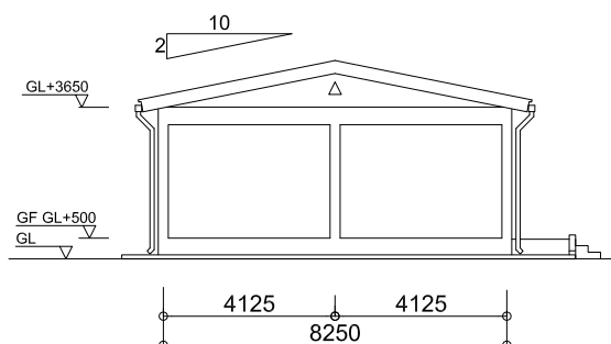
立面図（妻側）
