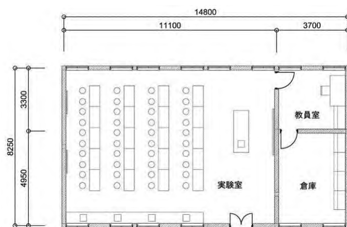
図 3-6 実験室（生物）平面図
