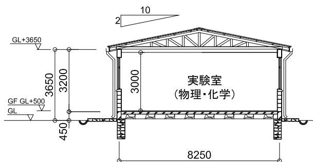
断面図
