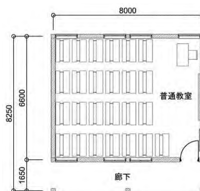
図 3-2 普通教室（初等学校）平面図
