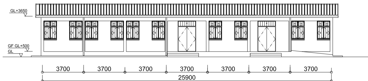
立面図 (入口側)
