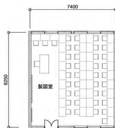
図 3-7 製図室平面図
