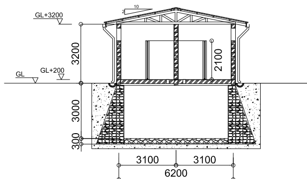
断面図
