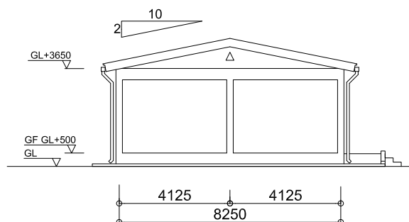
立面図（妻側）
