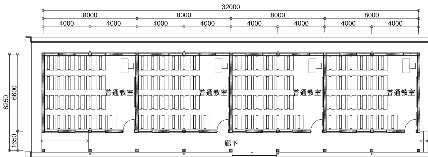
平面図
