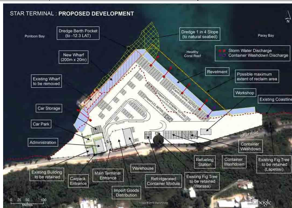
図 4.2-1 新埠頭の施設計画（排水位置）
