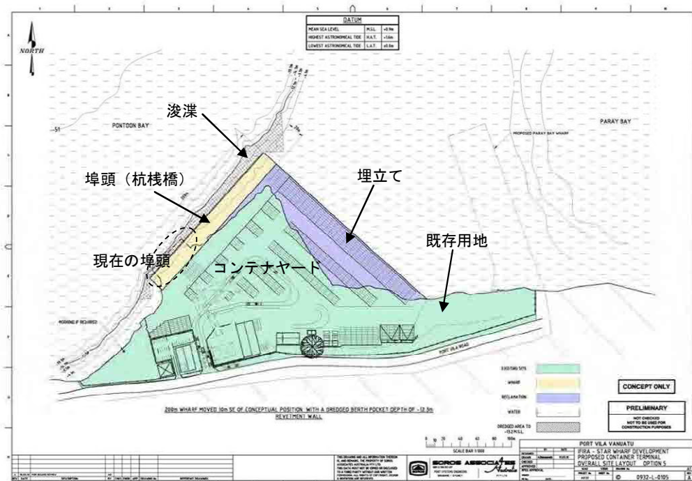
事業計画図（スター埠頭）
