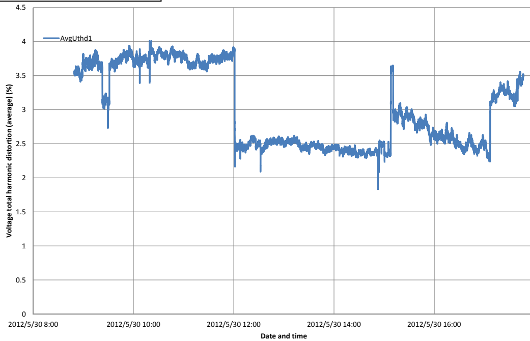
⑦ 総合高調波電圧歪率
