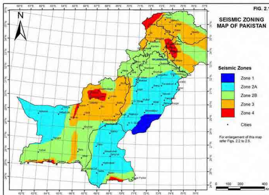
図 3-6：パキスタン国における地震ゾーニング図
