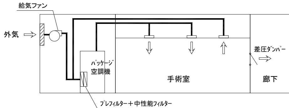
図 3-9 : 手術室空調換気概念図
