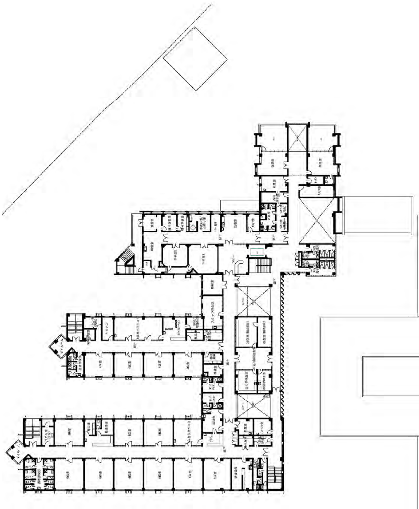
図 3-13 : 平面図 2 階
