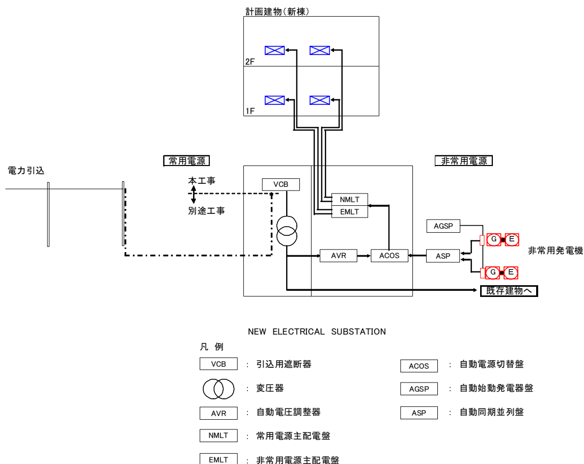
図 3-7 : 電力系統図
