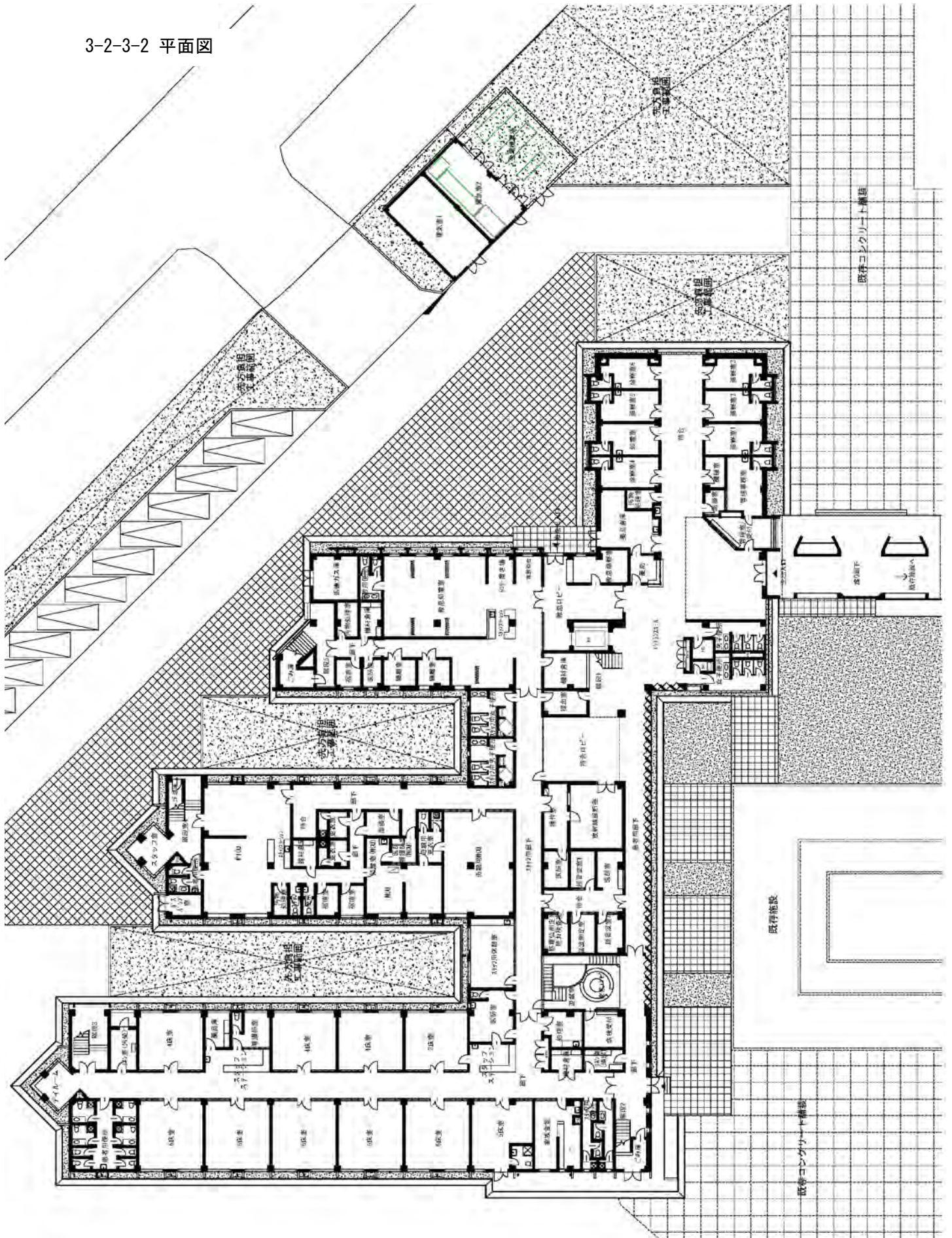
図 3-12 : 平面図 1 階
