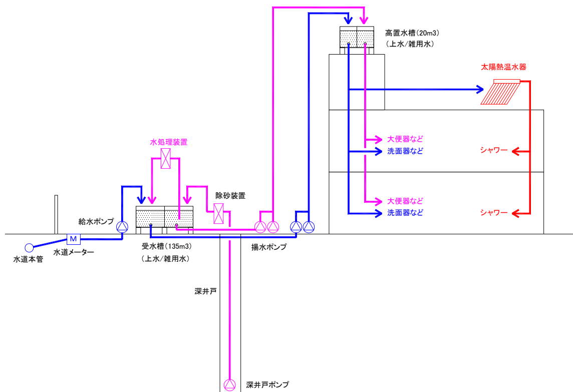
図 3-10 : 給水・給湯設備フロー図
