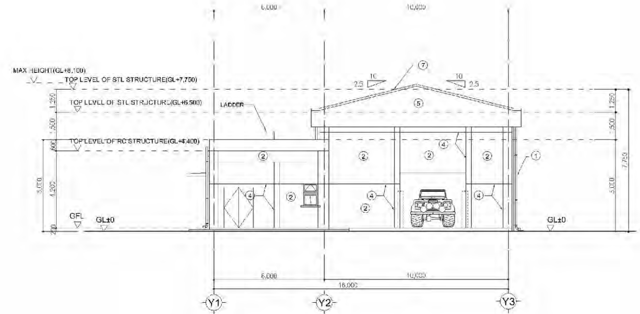
西侧立面图
