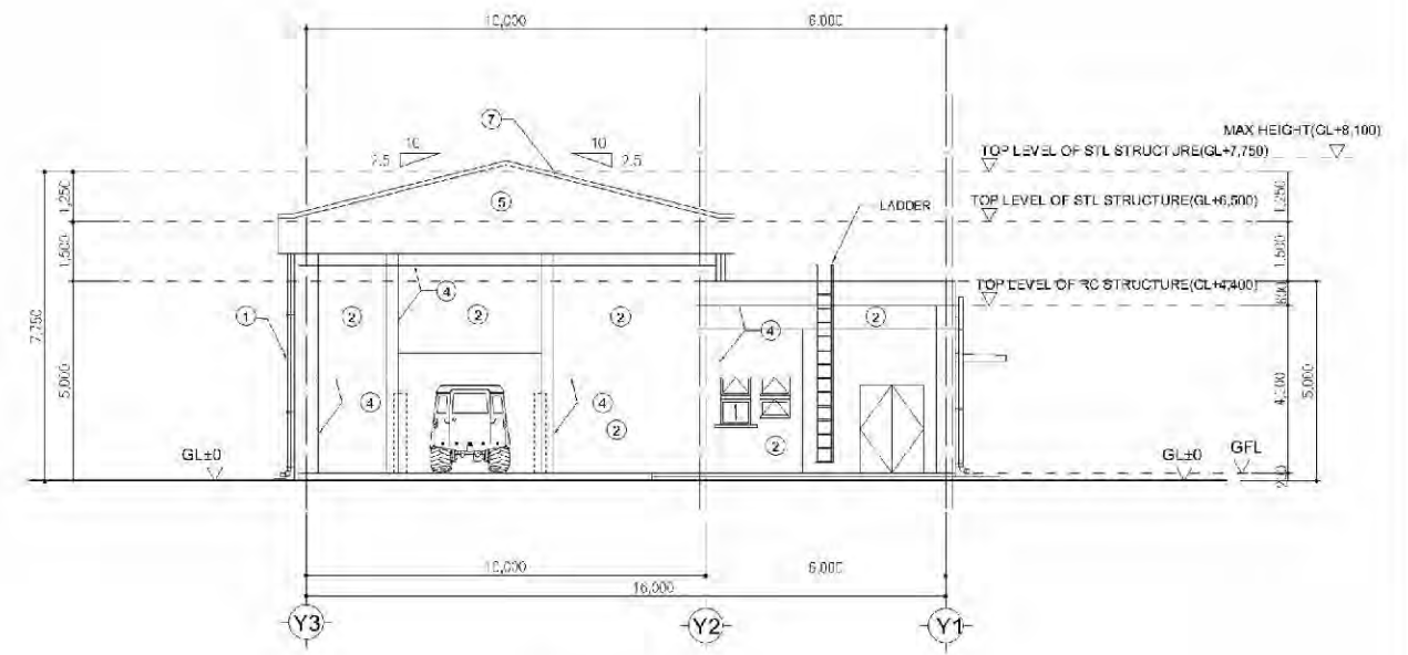
东侧立面图
