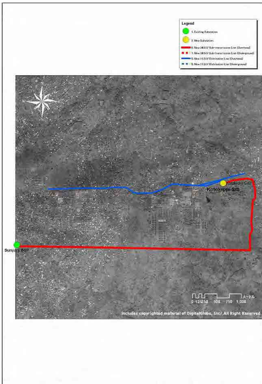
図 3-2-3.19 スンヤニ地区 配電ルート図
