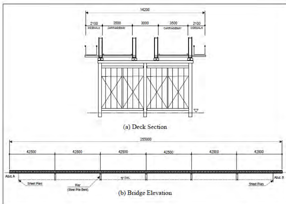
図 2-2-2 ジュバ橋の概略構造図
