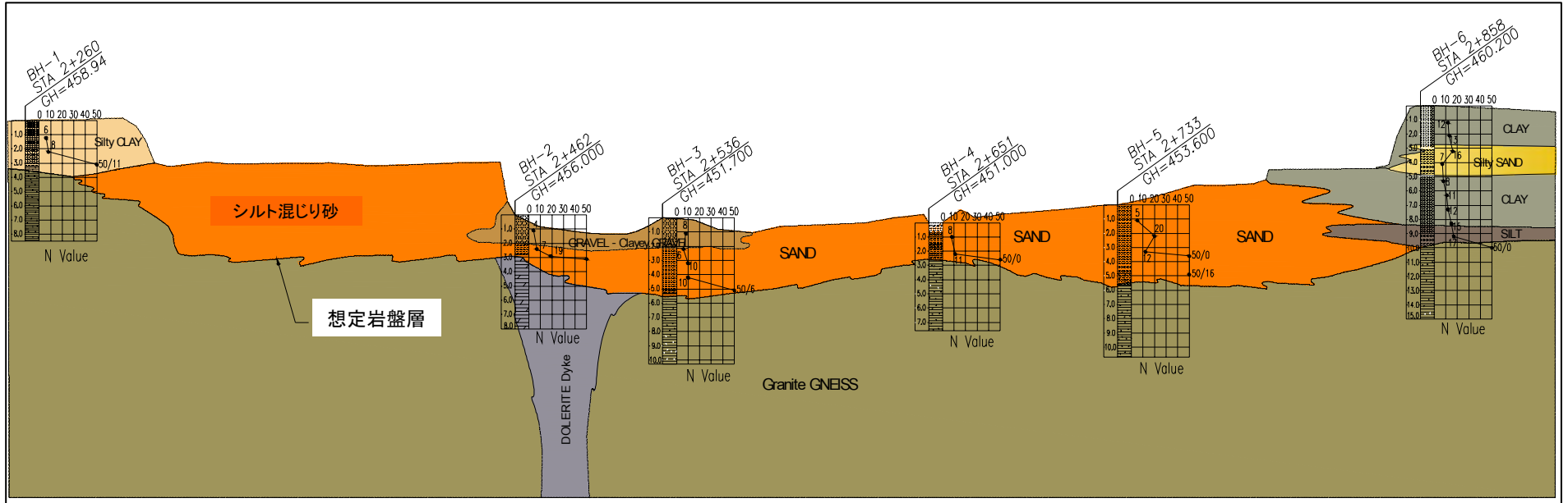
図 2-2-8 地質縦断面図
