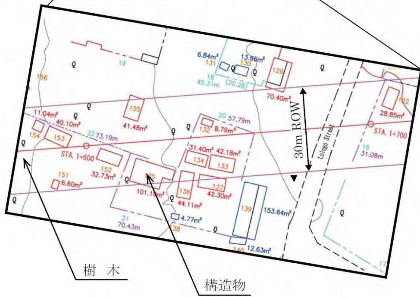
図 2-2-7 測量実施範囲および構造物・樹木調査位置
