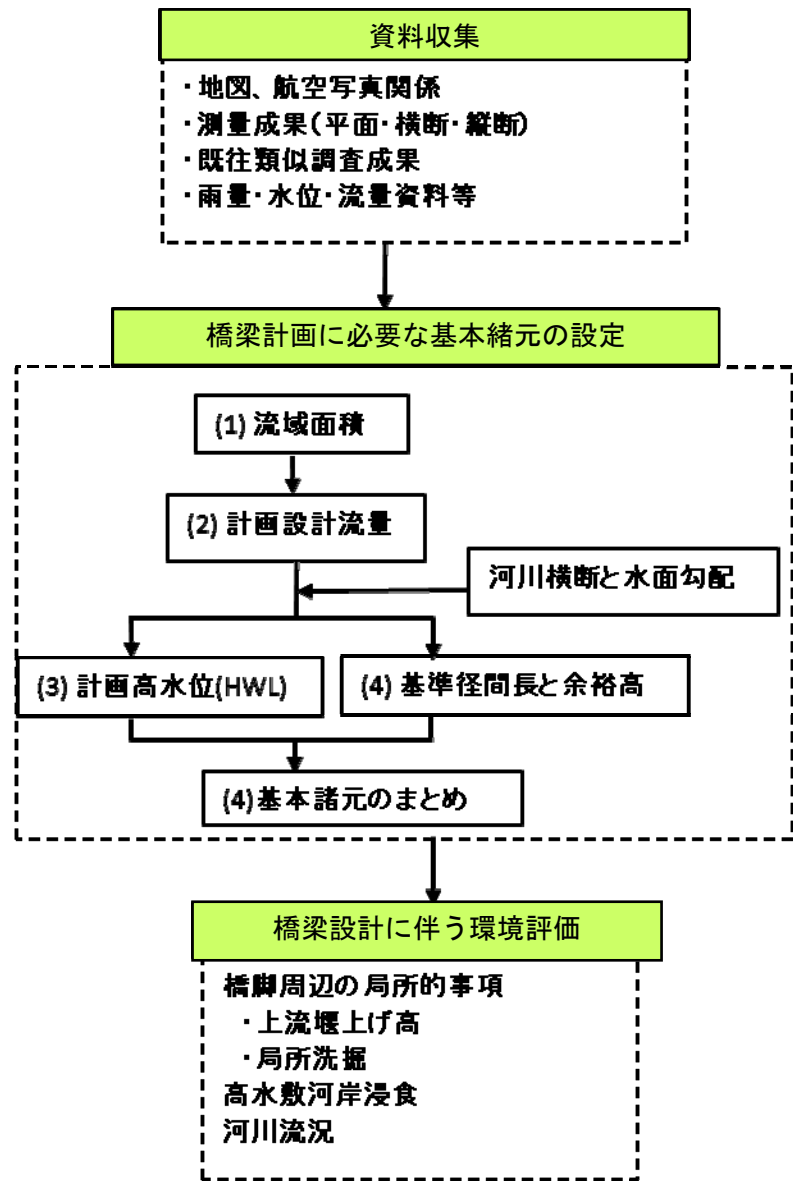
図 2-2-9 調査フロー
