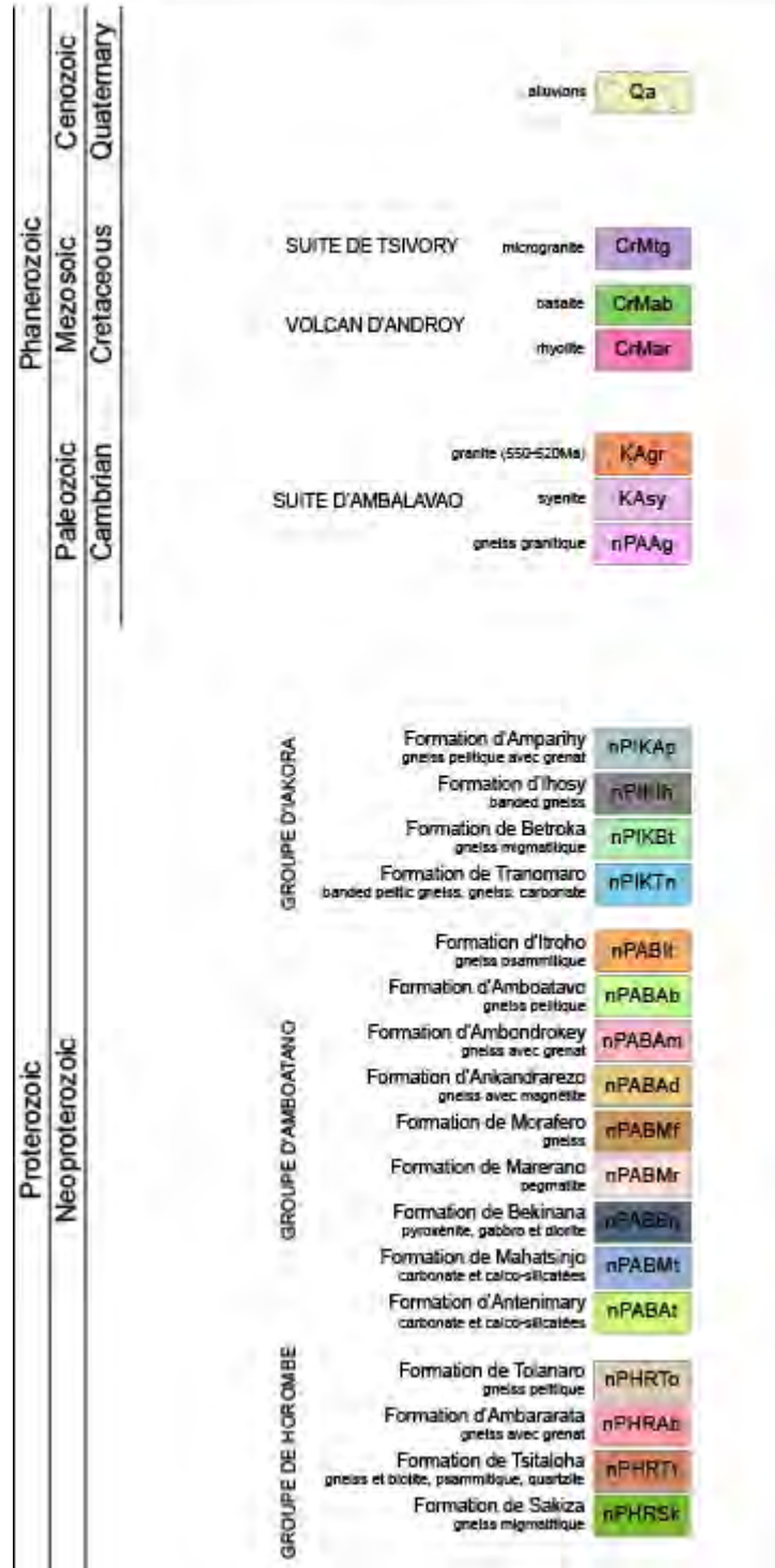
图 10 K59 地区 地質凡例
