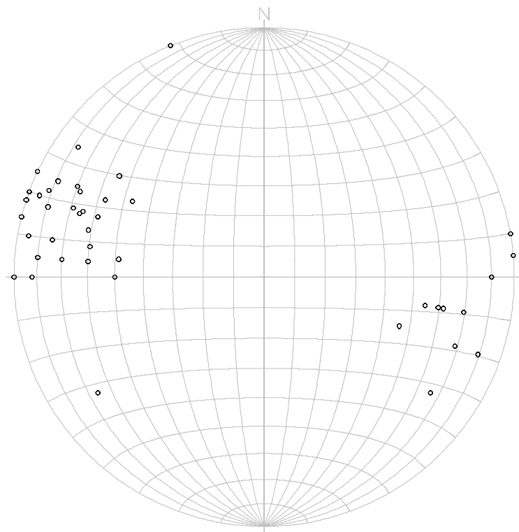
図 12 K58 地区 サブドメイン III 走向傾斜シュミットネット下半球投影図
