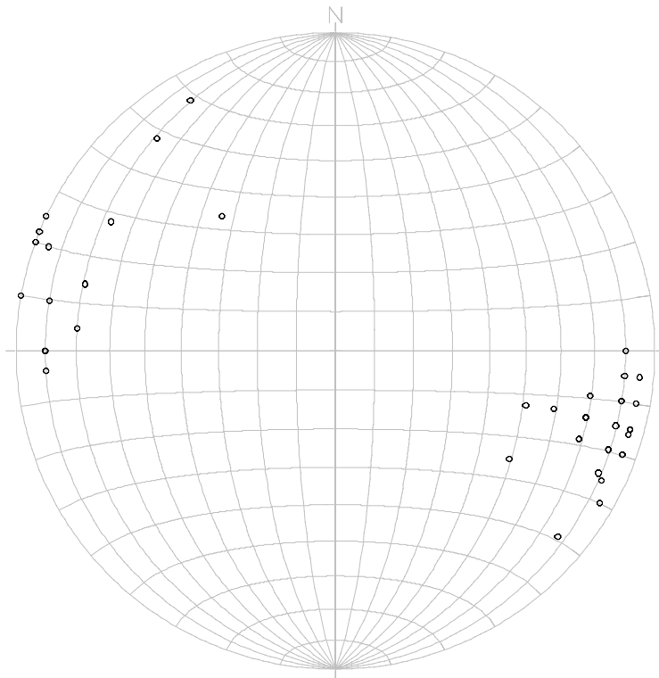
図 12 J60 地区 サブドメイン IV 走向傾斜シュミットネット下半球投影図
