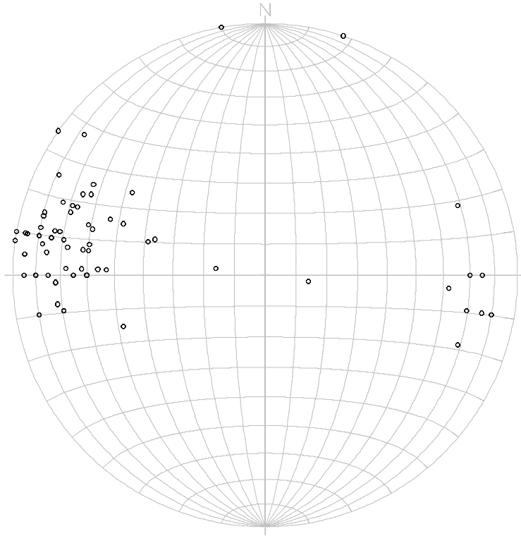
図 11 J60 地区 サブドメイン III 走向傾斜シュミットネット下半球投影図
