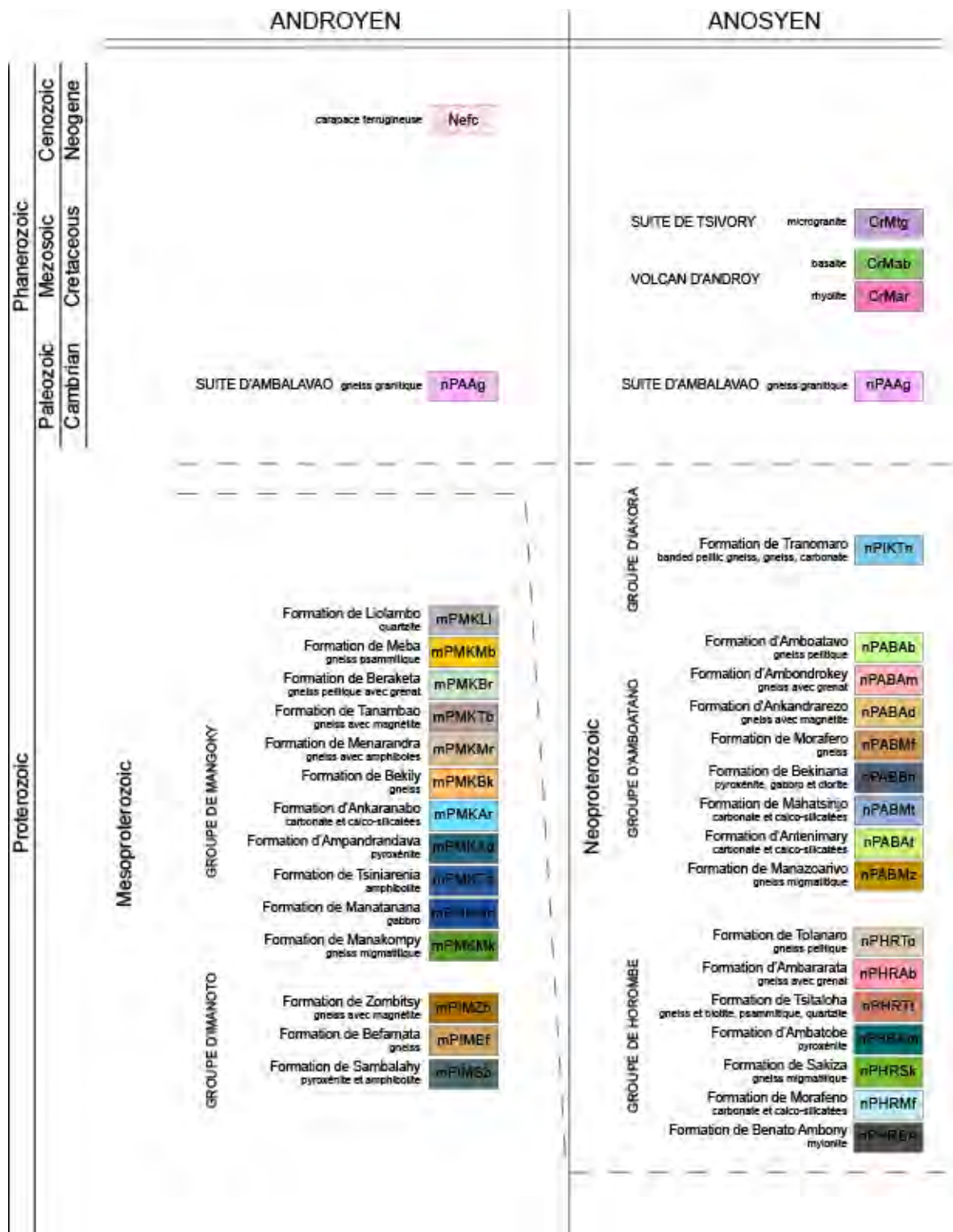
图 10 J60 地区 地質凡例
