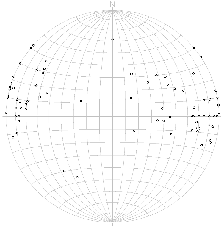
図 11 K58 地区 サブドメイン I 走向傾斜シュミットネット下半球投影図
