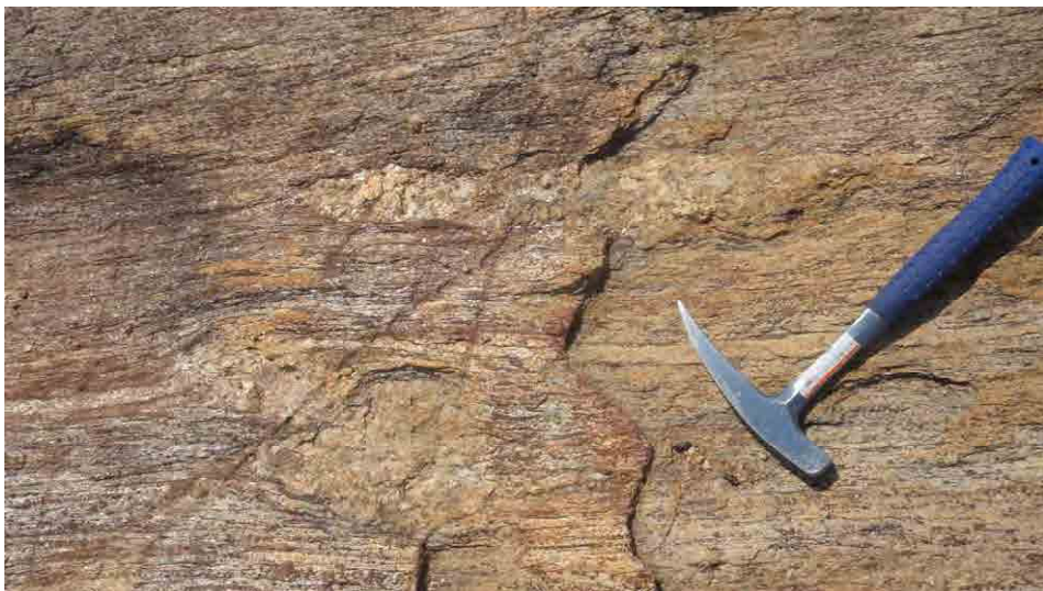
写真7 粗粒部分を含む泥質片麻岩
