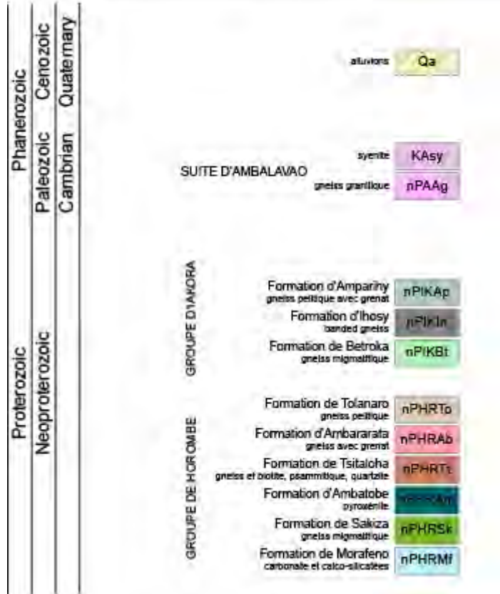
图 10 K58 地区 地質凡例
