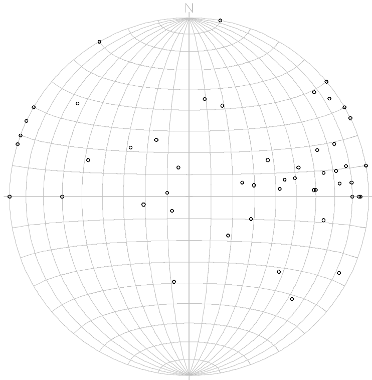
図 11 K59 地区 サブドメイン I 走向傾斜シュミットネット下半球投影図
