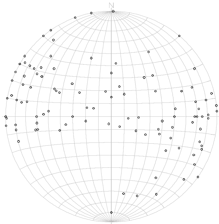
図 12 K59 地区 サブドメイン II 走向傾斜シュミットネット下半球投影図
