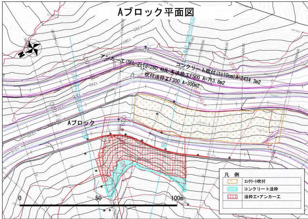
図 3.2.10 A ブロック アンカー工案平面図
