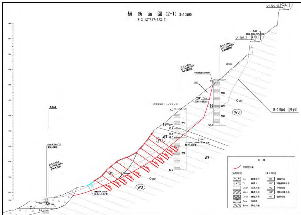
図 3.2.15 B ブロック アンカー工案断面図
