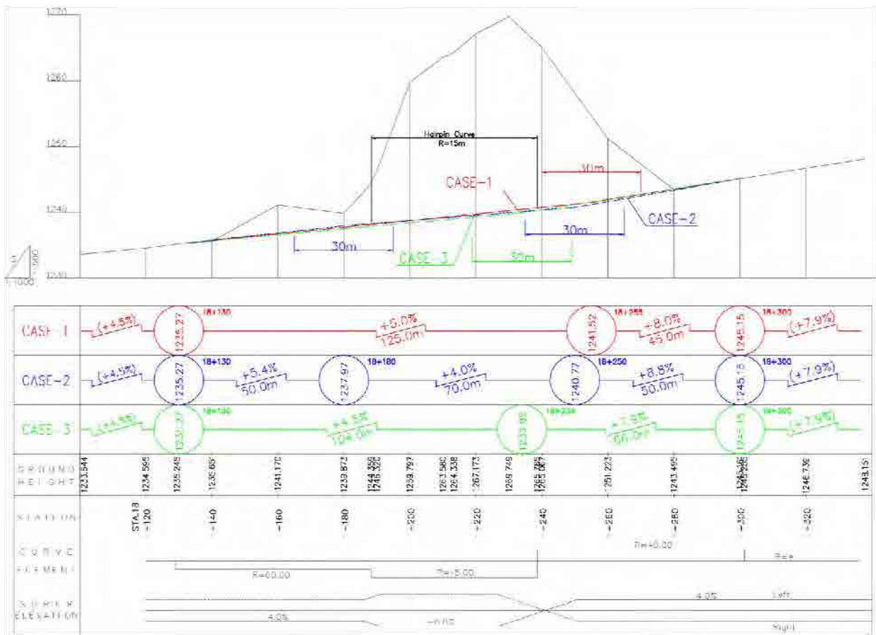
図 3.2.36 縦断検討図
