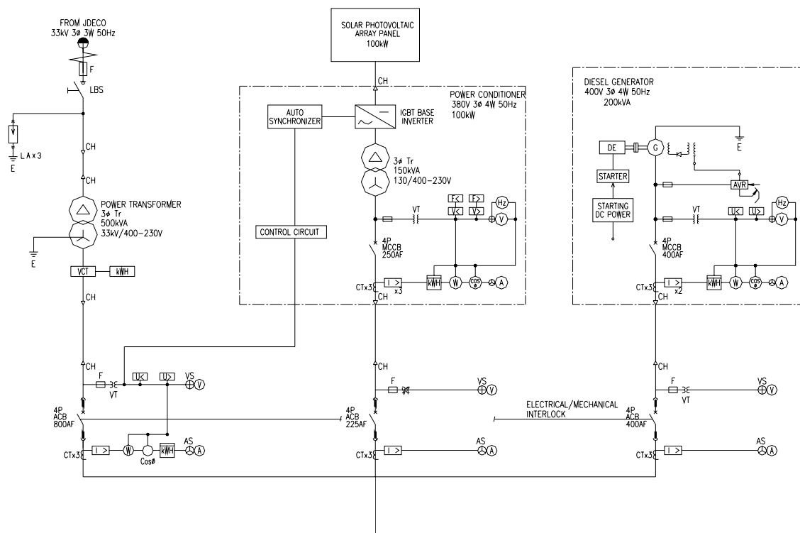
図 3-4 電気単線結線図
