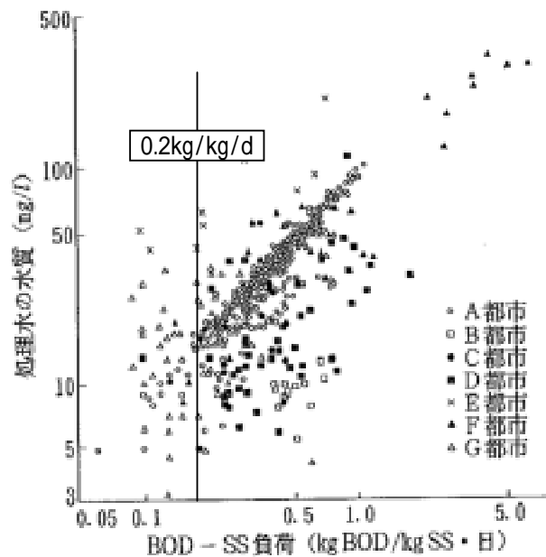
図3-3 BOD SS負荷と処理水質 出展：下水道施設計画・設計指針解説(2001年版)
