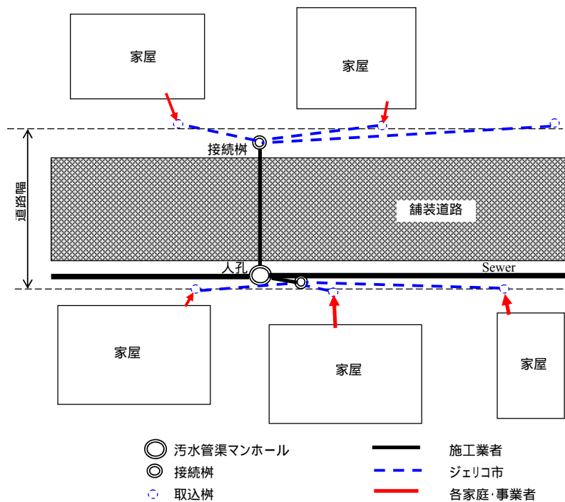
図 3-6 各家庭等からの汚水の接続方法
