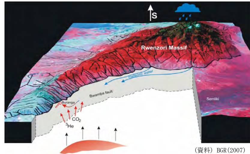
Buranga地域の三次元モデル
