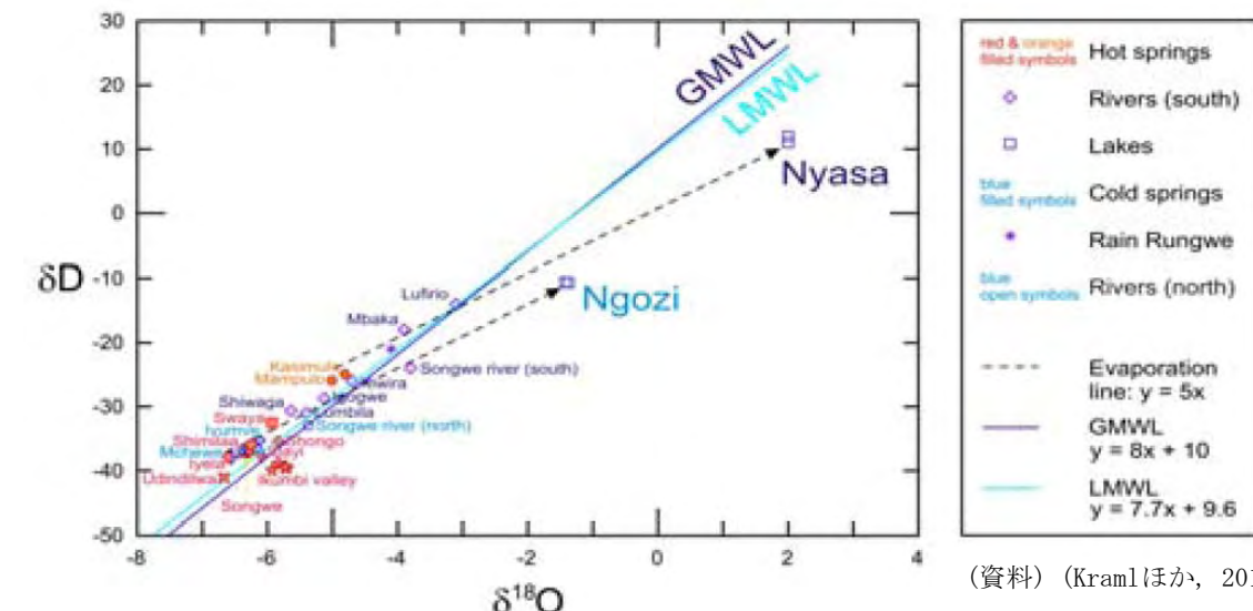
Mbeya地域の温泉水の水の水素・酸素同位体比関係図
