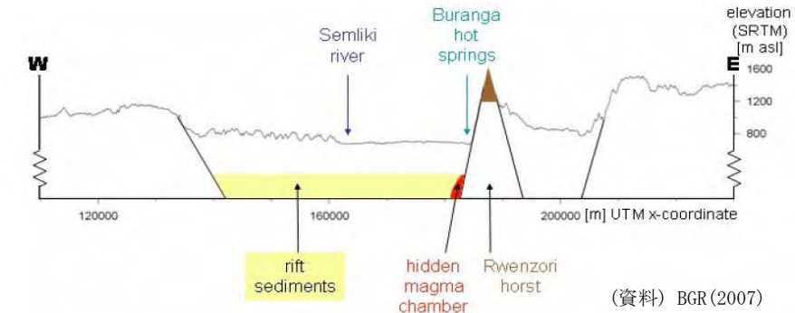
Buranga地域の地熱系概念モデル断面図
