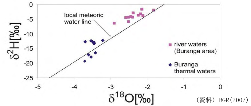
Buranga地域の温泉水・河川水の水素・酸素同位体比関係図
