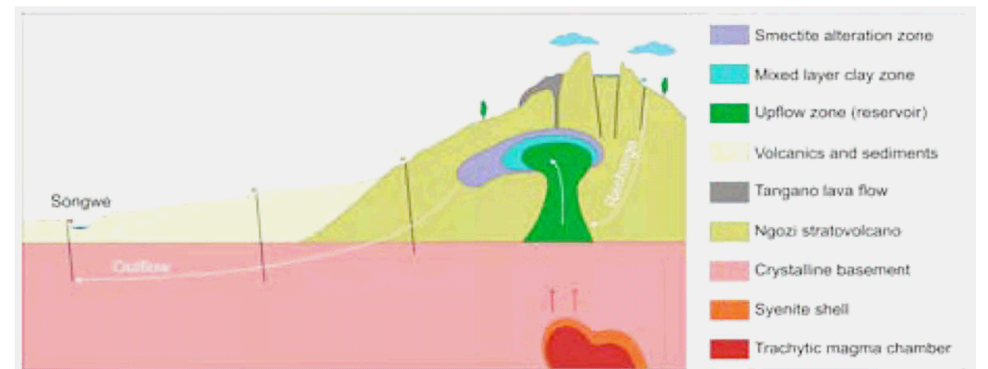
Mbeya地域の地熱系概念モデル（断面）
