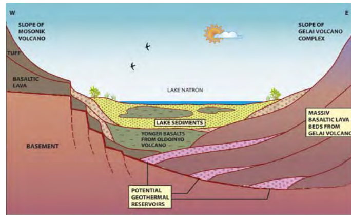
図-7. 4-9 Natron湖地域の地質構造概念モデル
