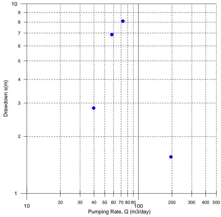
TM2_Diawara1 essai palier-3
