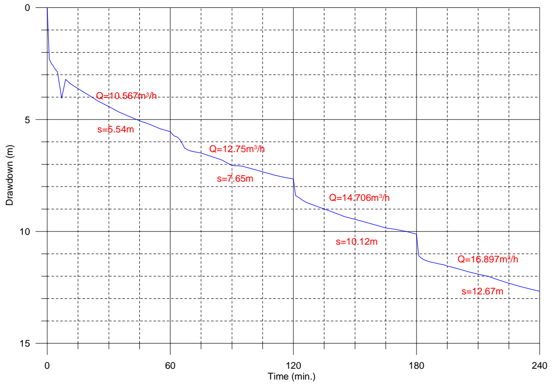
TM5_Ganguel Maka essai palier-1
