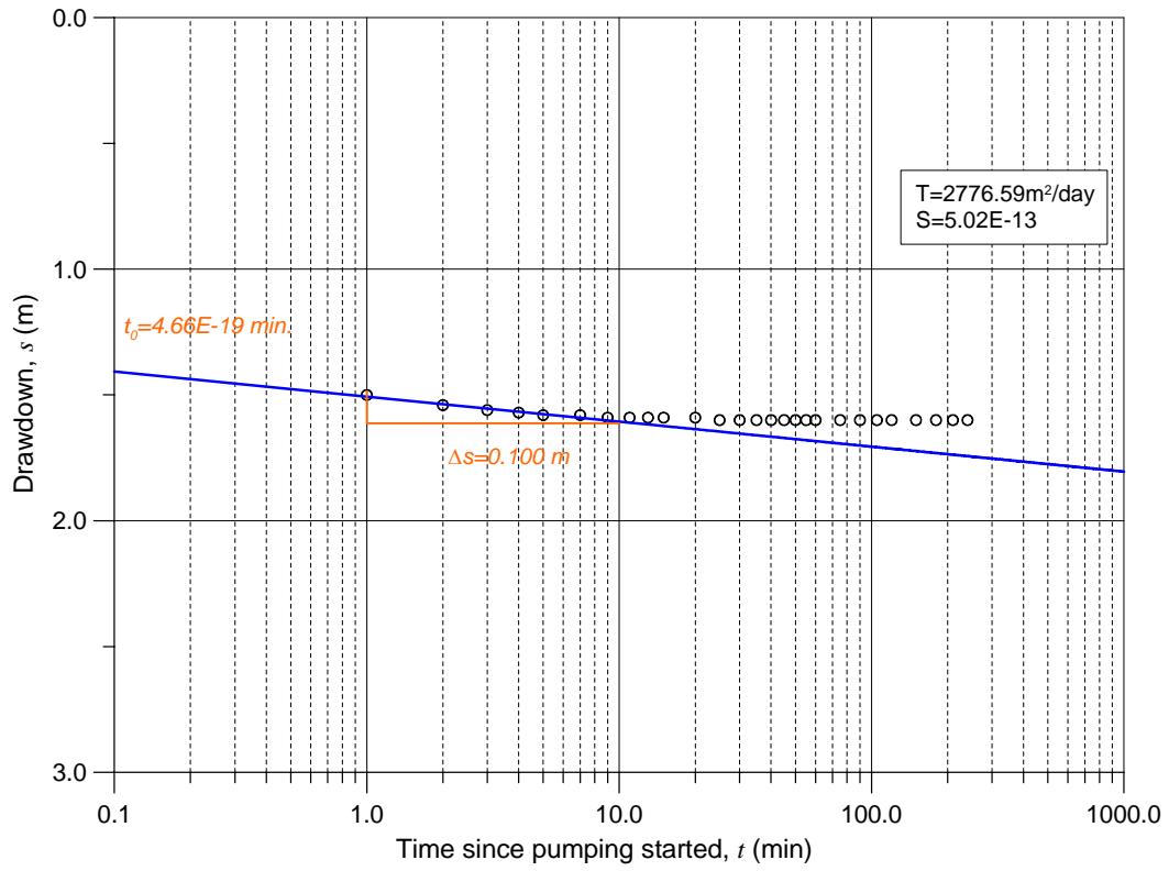
TM13_Dindoudi Doaka Cooper-Jacobmethode
