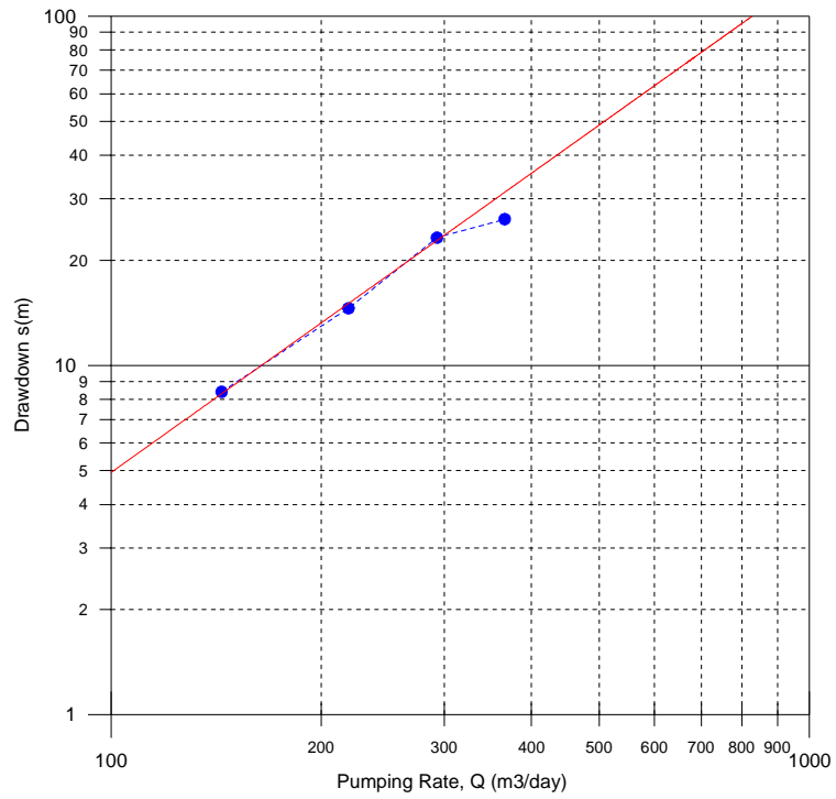
TM10_Diaria essai palier-3
