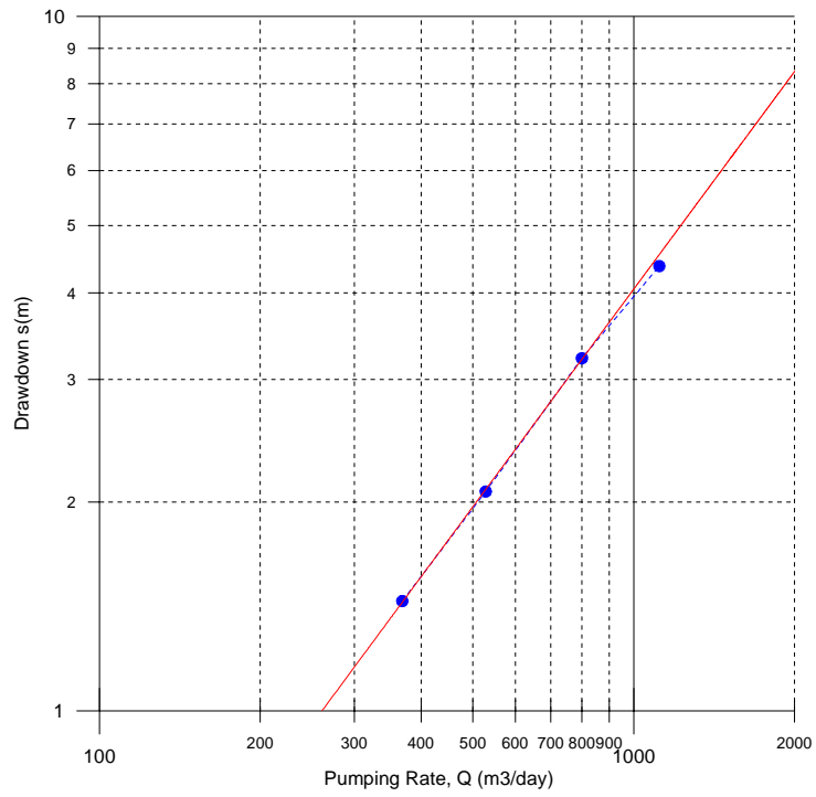
TM1_Ainou Mahdy essai palier-3
