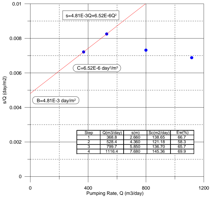
TM12_Soutouta essai palier-2
