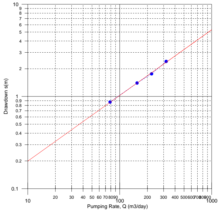
TM7_Takoura essai palier-3
