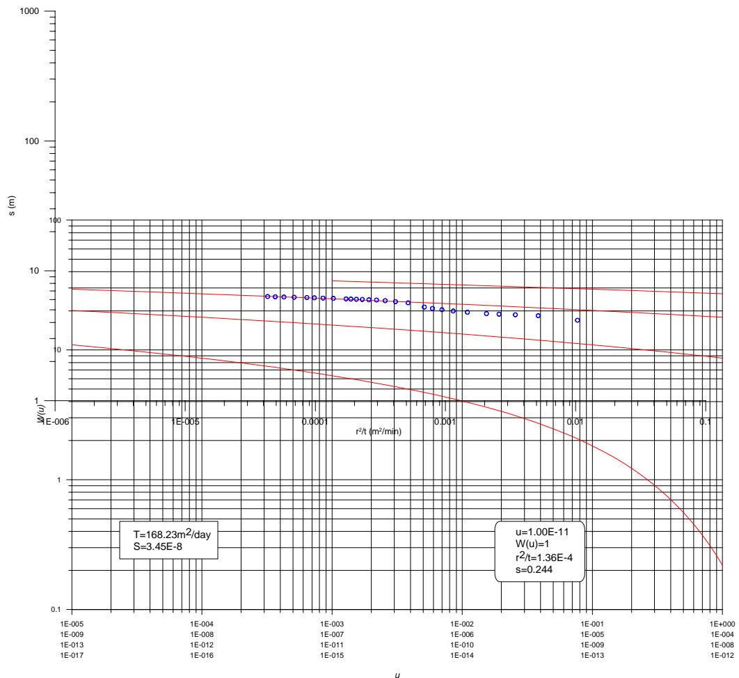
TM4_Diawara2 Theismethode
