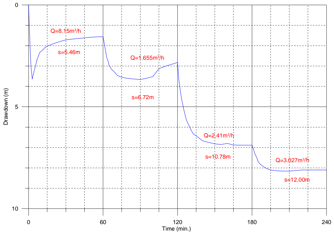
TM2_Diawara1 essai palier-1
