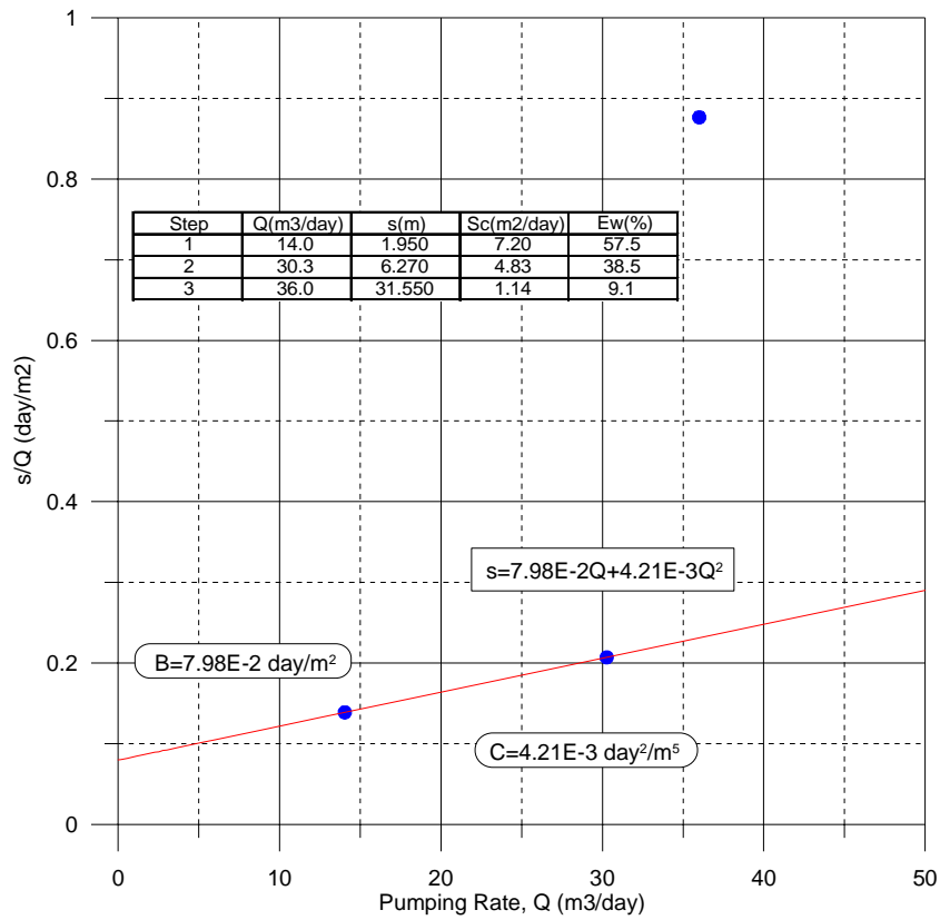
TM6_Yerimale essai palier-2
