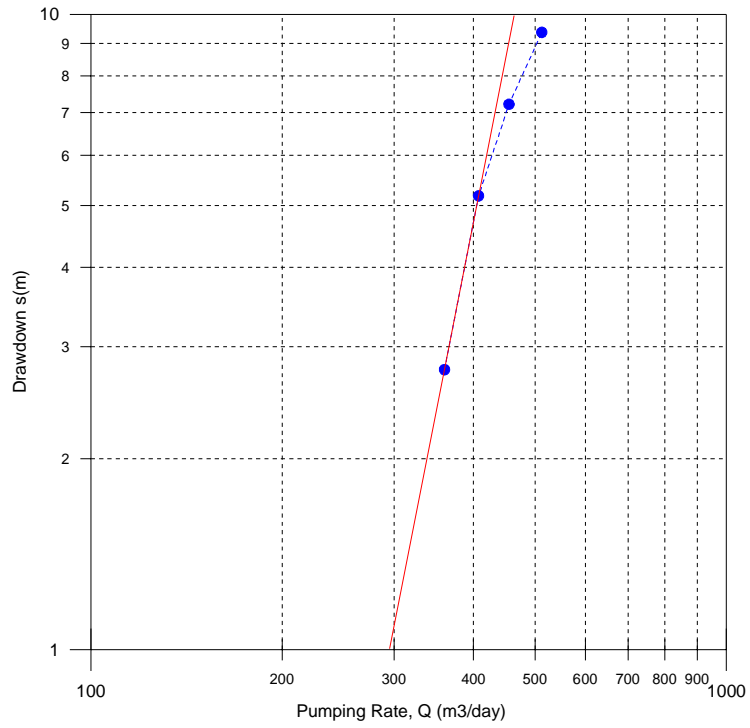
TM9_Medina Diakha essai palier-3
