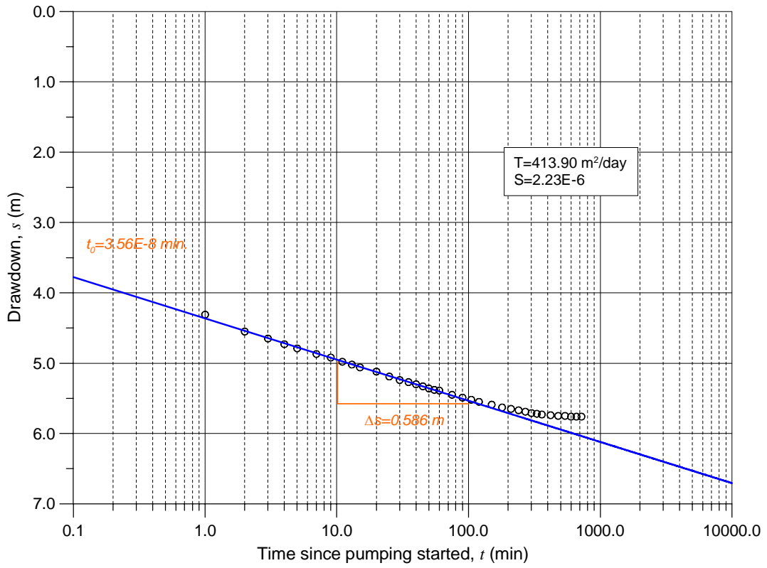
TM11_Thiengolele Cooper-Jacobmethode
