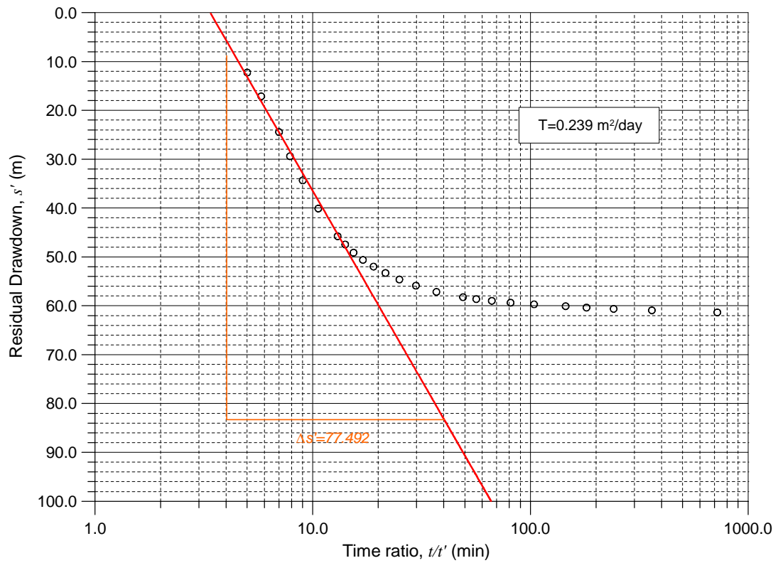
TM7_Khossanto par methode etablisement
