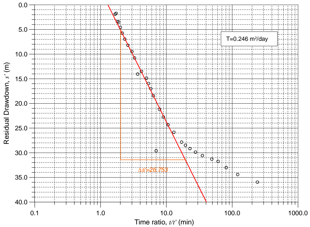
TM6_Yerimale par methode etablisement
