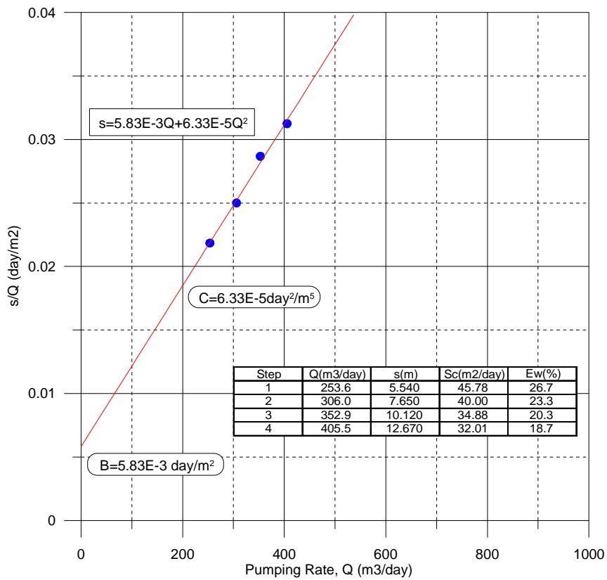
TM5_Ganguel Maka essai palier-2
