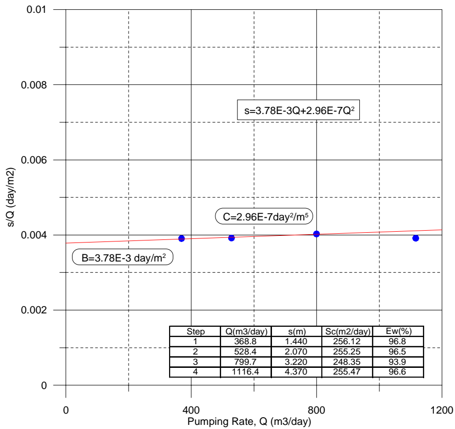
TM1_Ainou Mahdyessai palier-2
