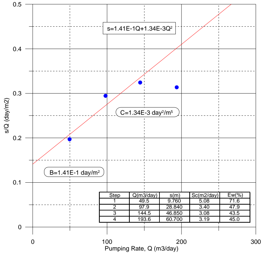
TM7_Khossanto essai palier-2
