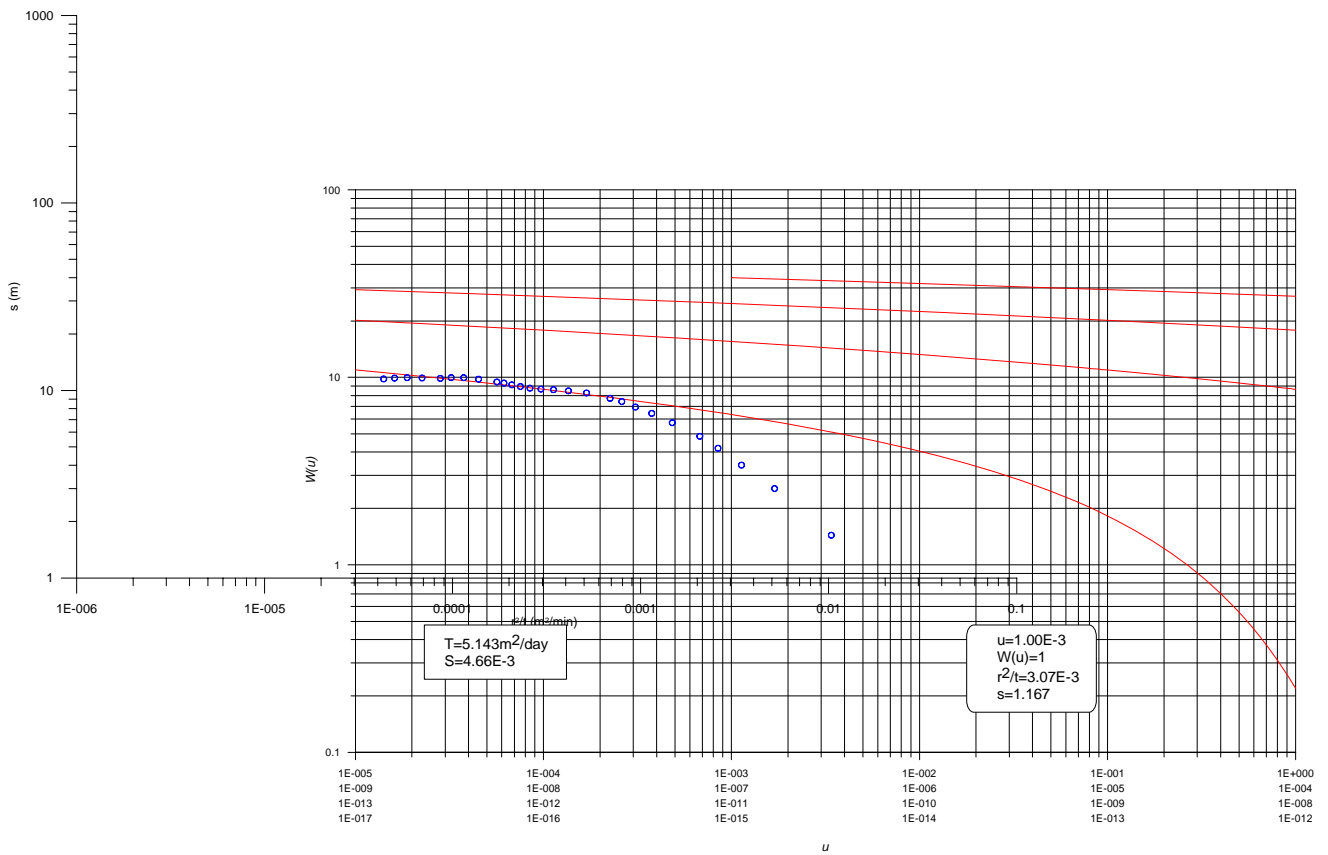
TM2_Diawara1 Theismethode
