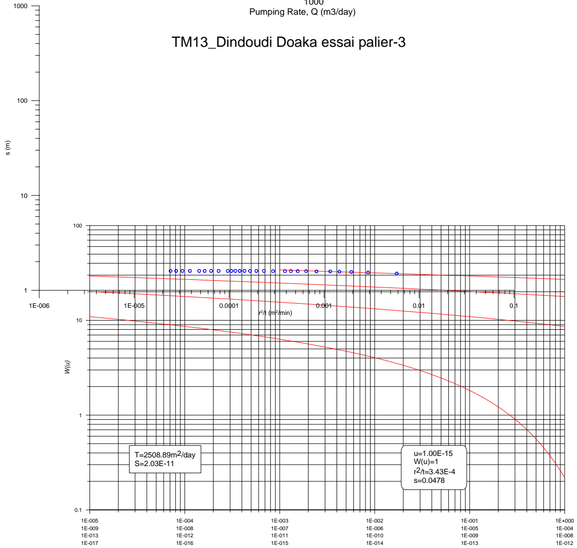
TM13_Dindoudi Doaka Theismethode
