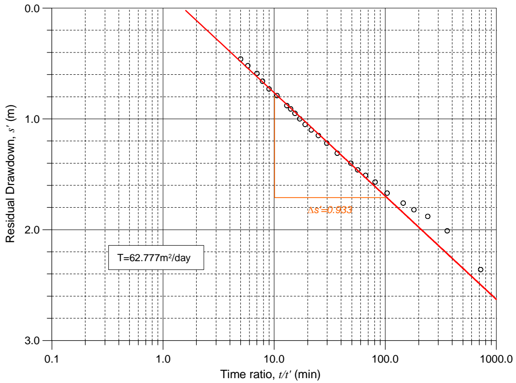
TM7_Takoura par methode etablisement
