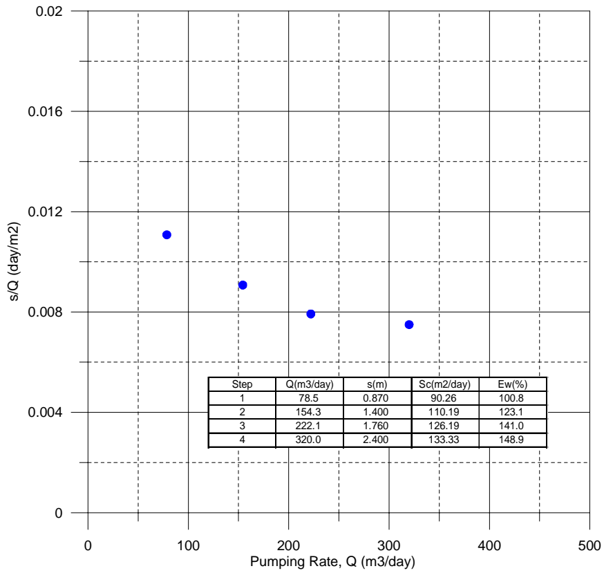
TM7_Takoura essai palier-2
