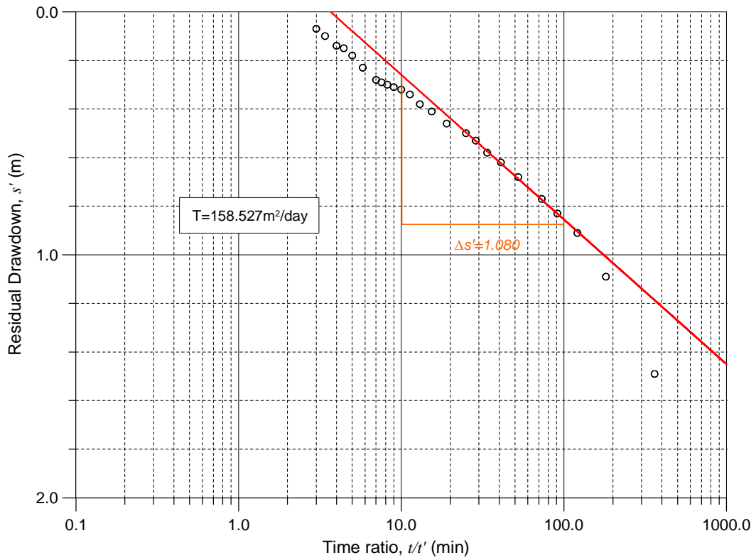
TM4_Diawara2 par methode etablisement
