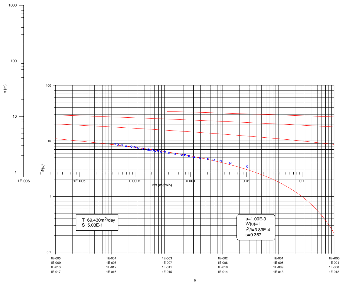
TM7_Takoura Theismethode
