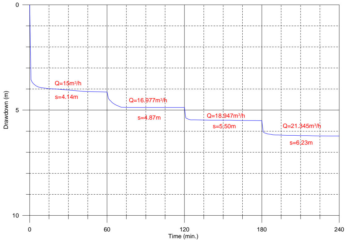
TM4_Diawara2 essai palier-1
