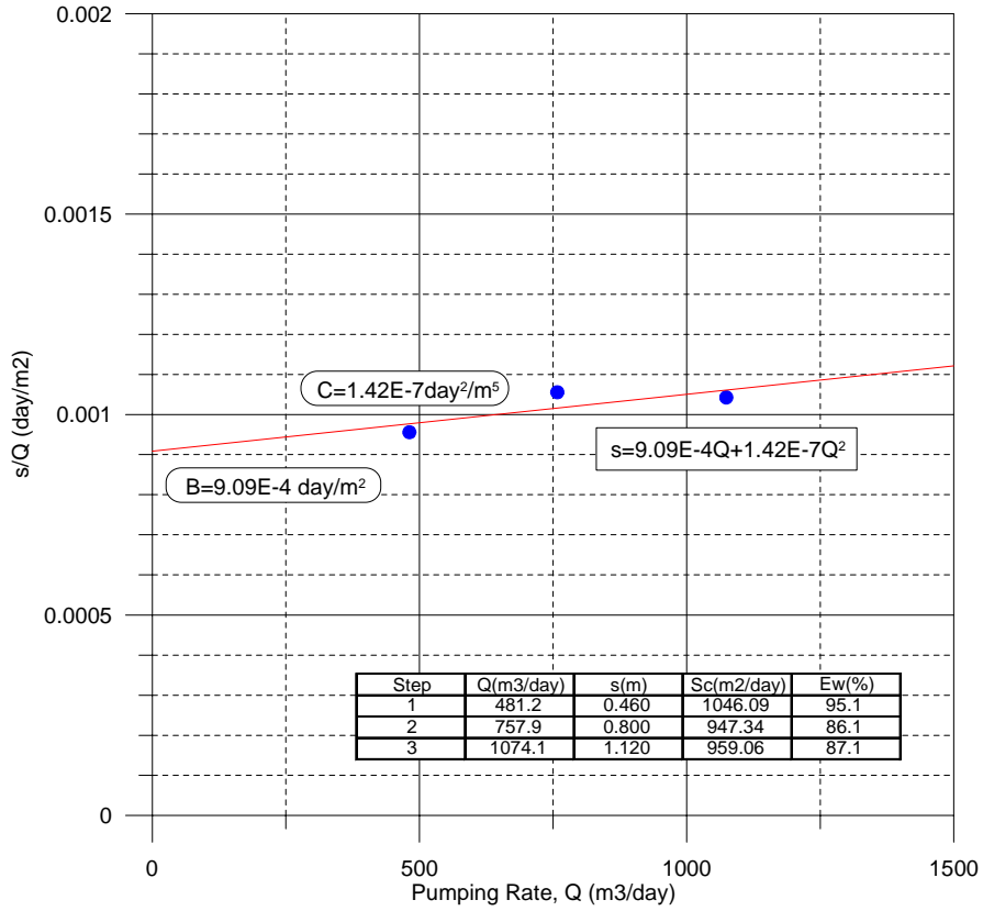
TM13_Dindoudi Doaka essai palier-2
