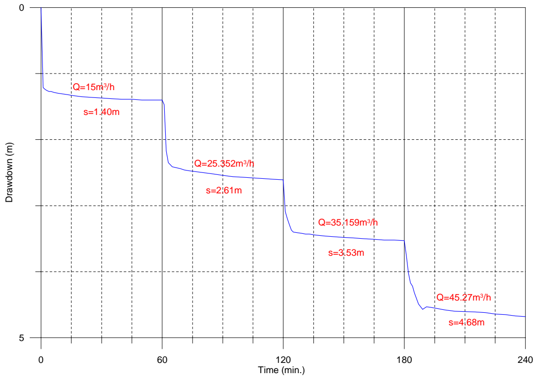
TM11_Thiengolele essai palier-1
