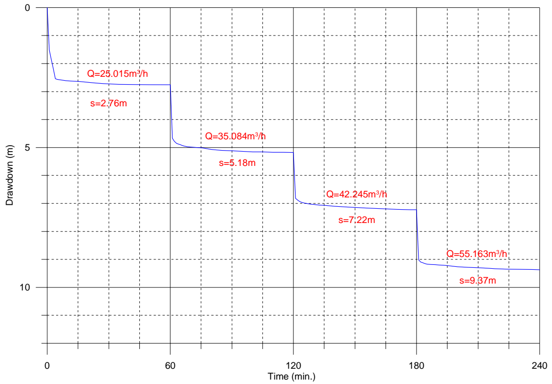
TM9_Medina Diakha essai palier-1
