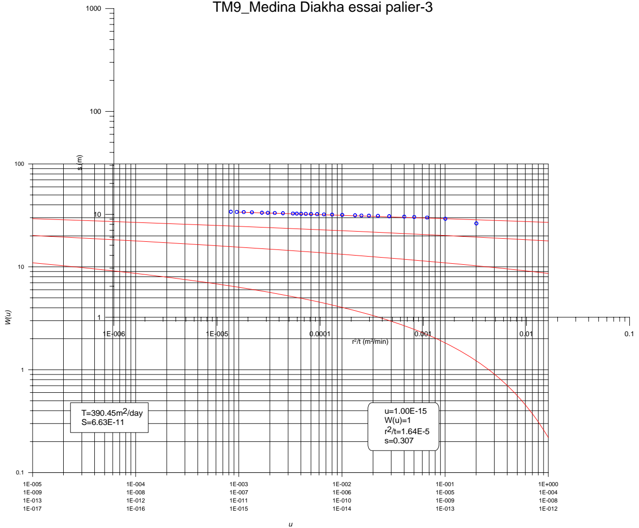
TM9_Medina Diakha Theismethode
