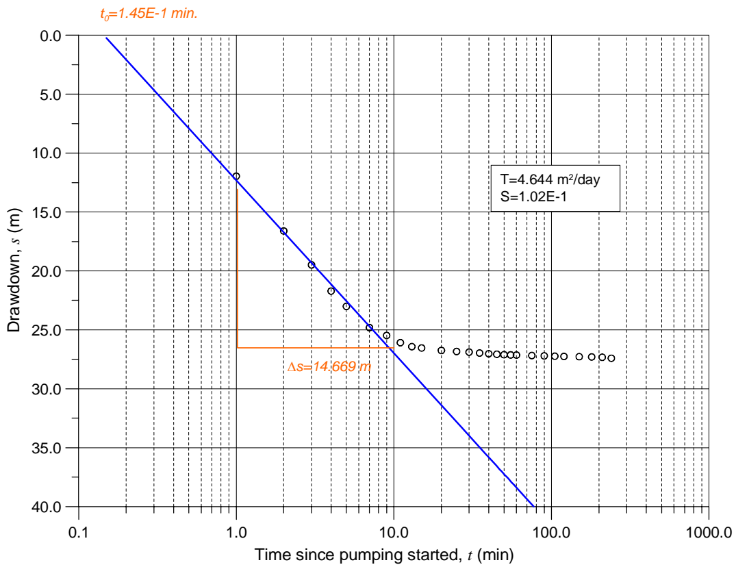
TM10_Diaria Cooper-Jacobmethode
