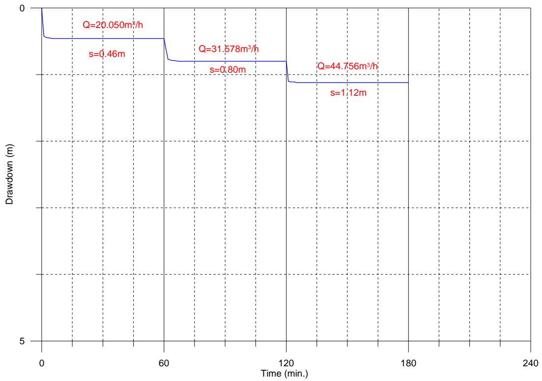
TM13_Dindoudi Doaka essai palier-1
