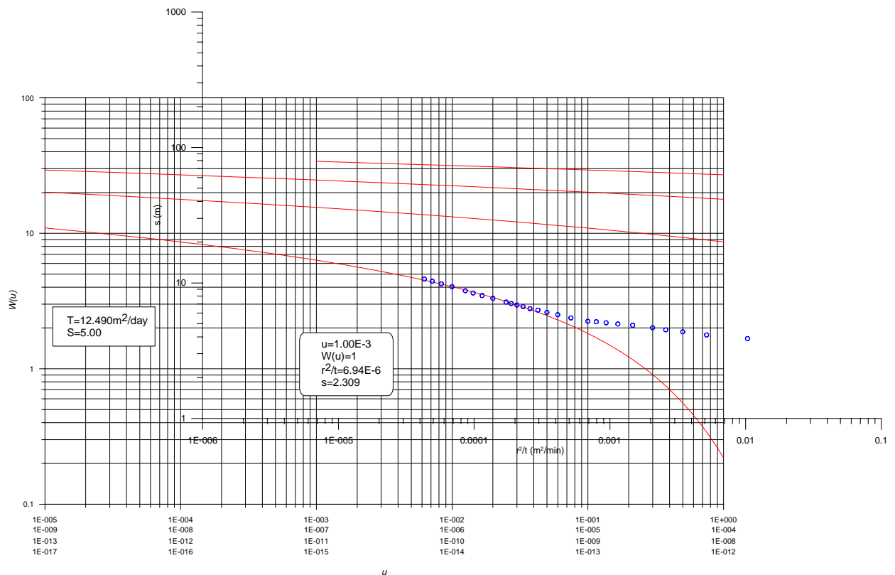
TM5_Ganguel Maka Theismethode
