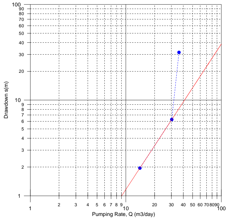
TM6_Yerimale essai palier-3
