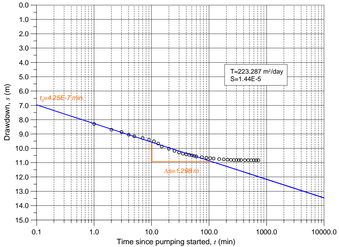
TM12_Soutouta Cooper-Jacobmethode
