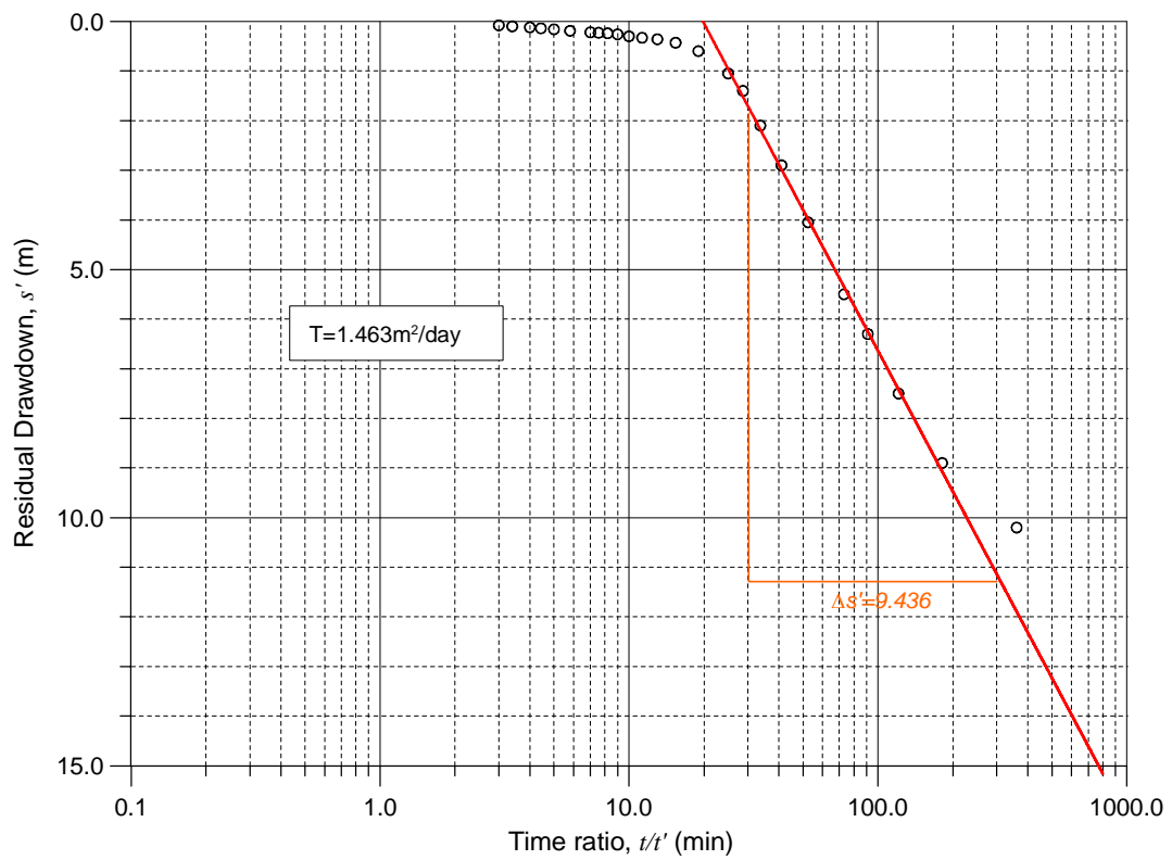
TM2_Diawara1 par methode etablisement
