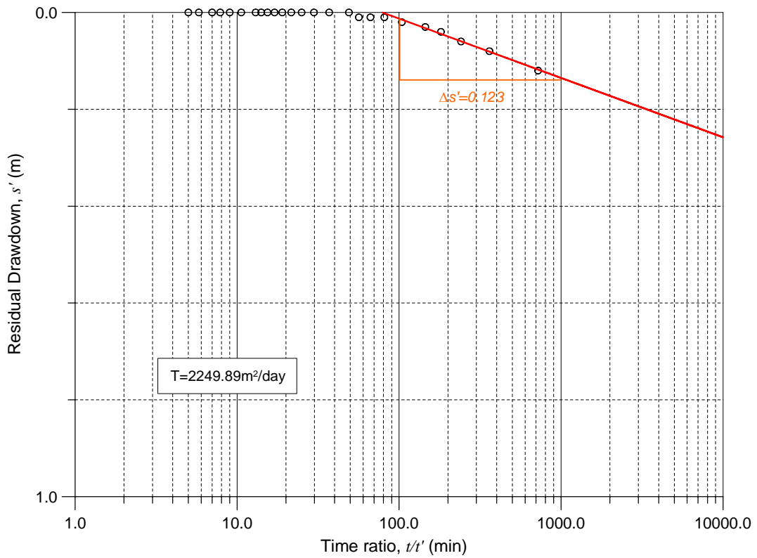
TM13_Dindoudi Doaka par methode etablisement
