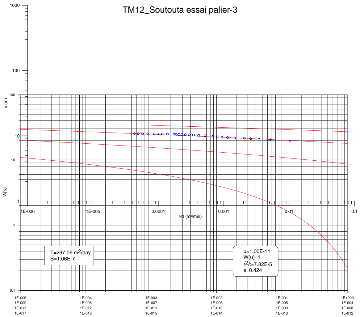
TM12_Soutouta Theismethode
