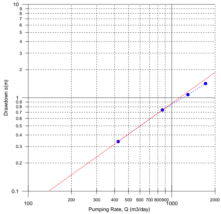
TM3_Gande essai palier-3
