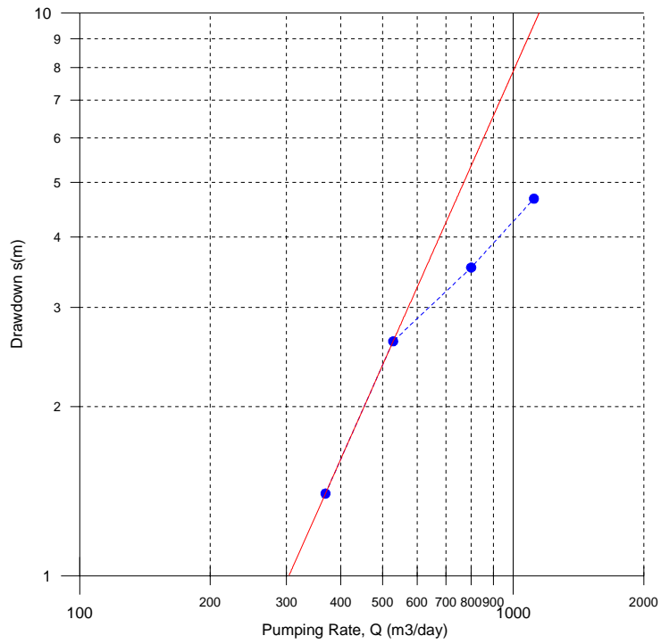
TM11_Thiengolele essai palier-3
