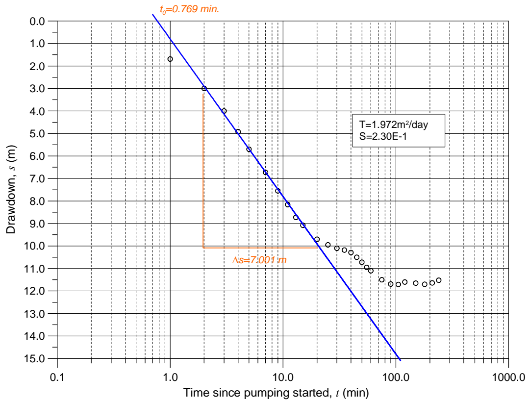
TM2_Diawara1 Cooper-Jacobmethode
