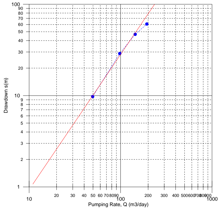
TM7_Khossanto essai palier-3
