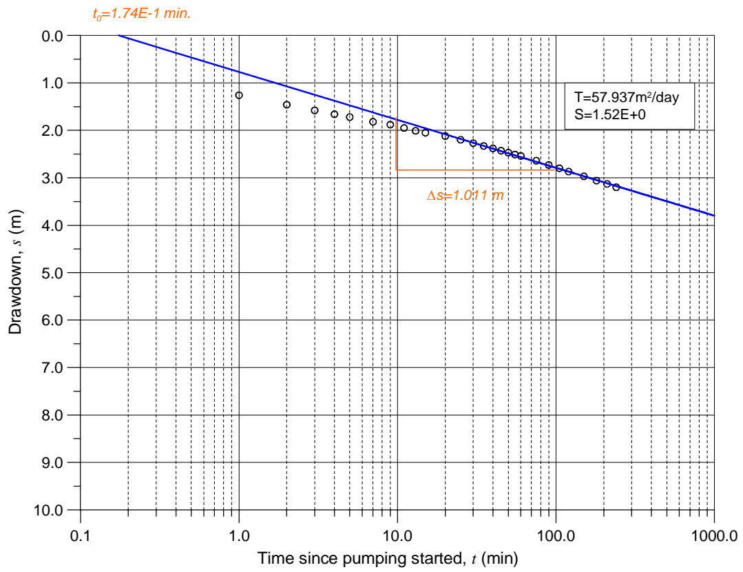
TM7_Takoura Cooper-Jacobmethode
