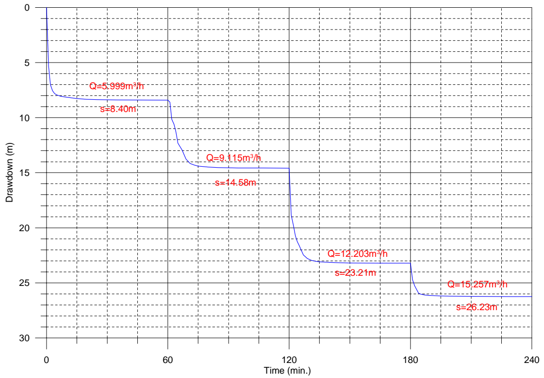
TM10_Diaria essai palier-1
