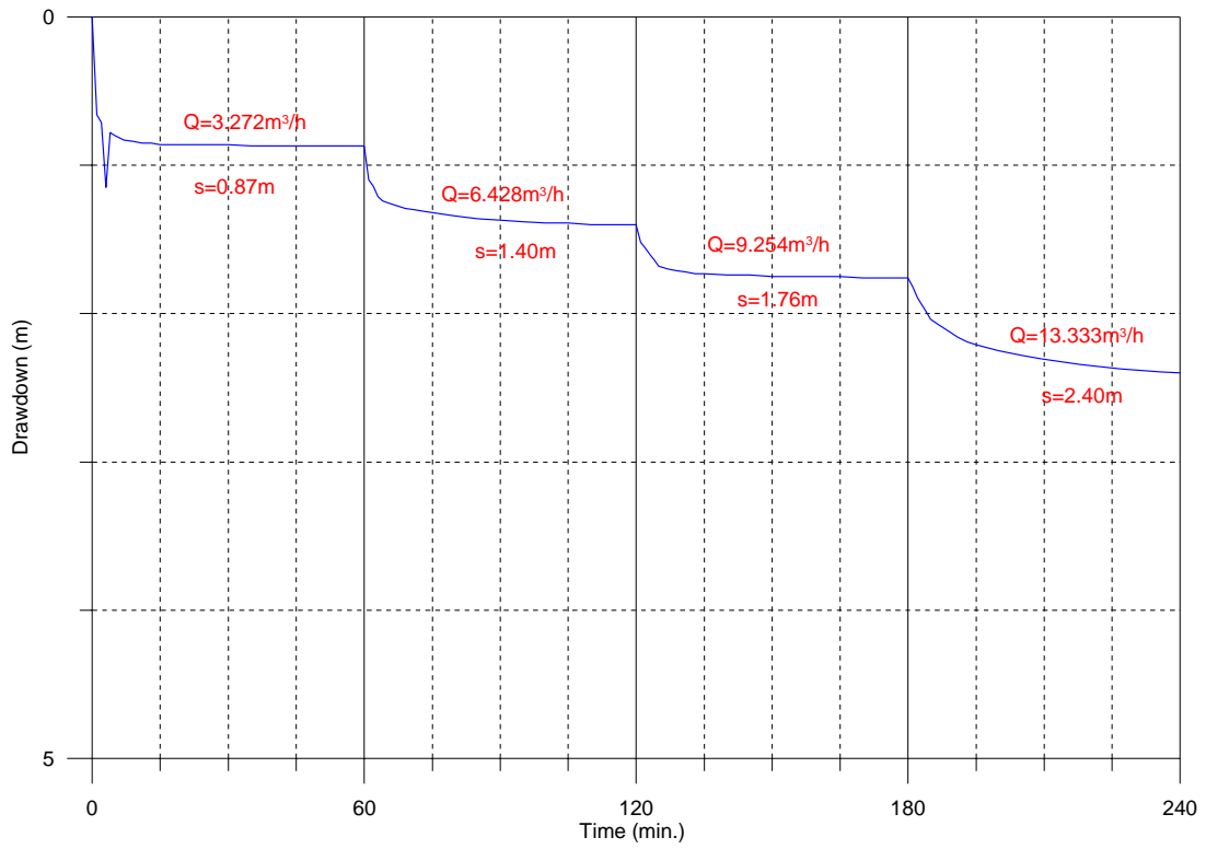
TM7_Takoura essai palier-1
