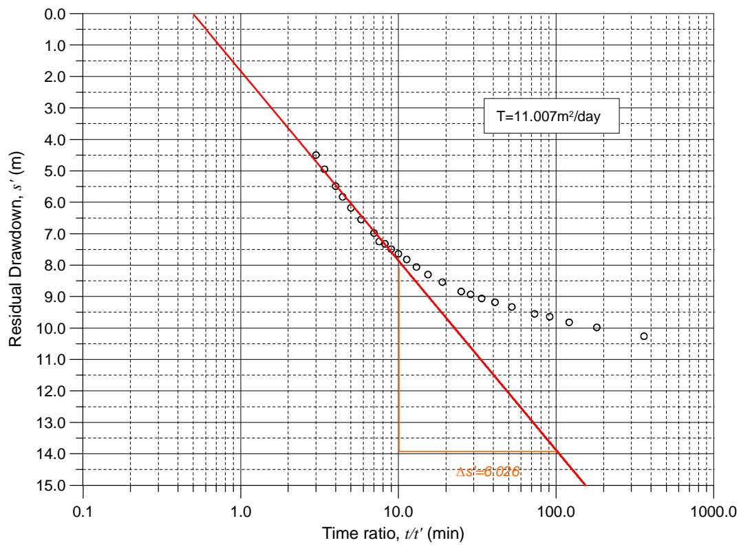
TM5_Ganguel Maka par methode etablissement
