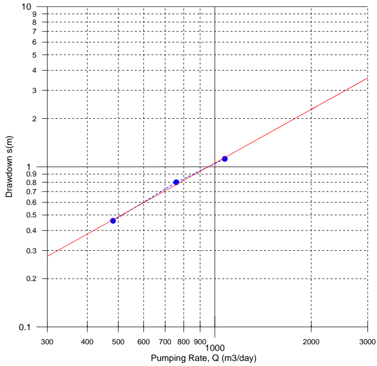
TM13_Dindoudi Doaka essai palier-3
