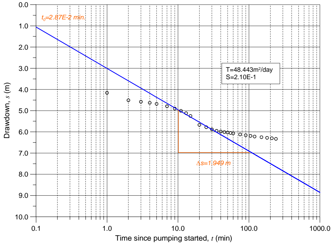
TM4_Diawara2 Cooper-Jacobmethode
