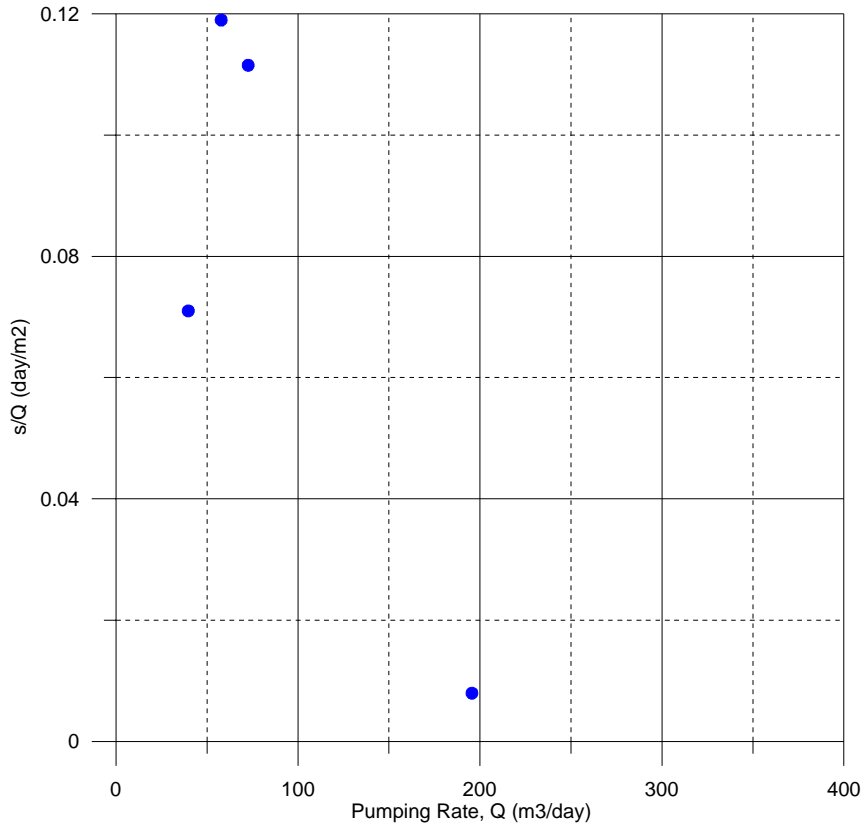
TM2_Diawara1 essai palier-2
