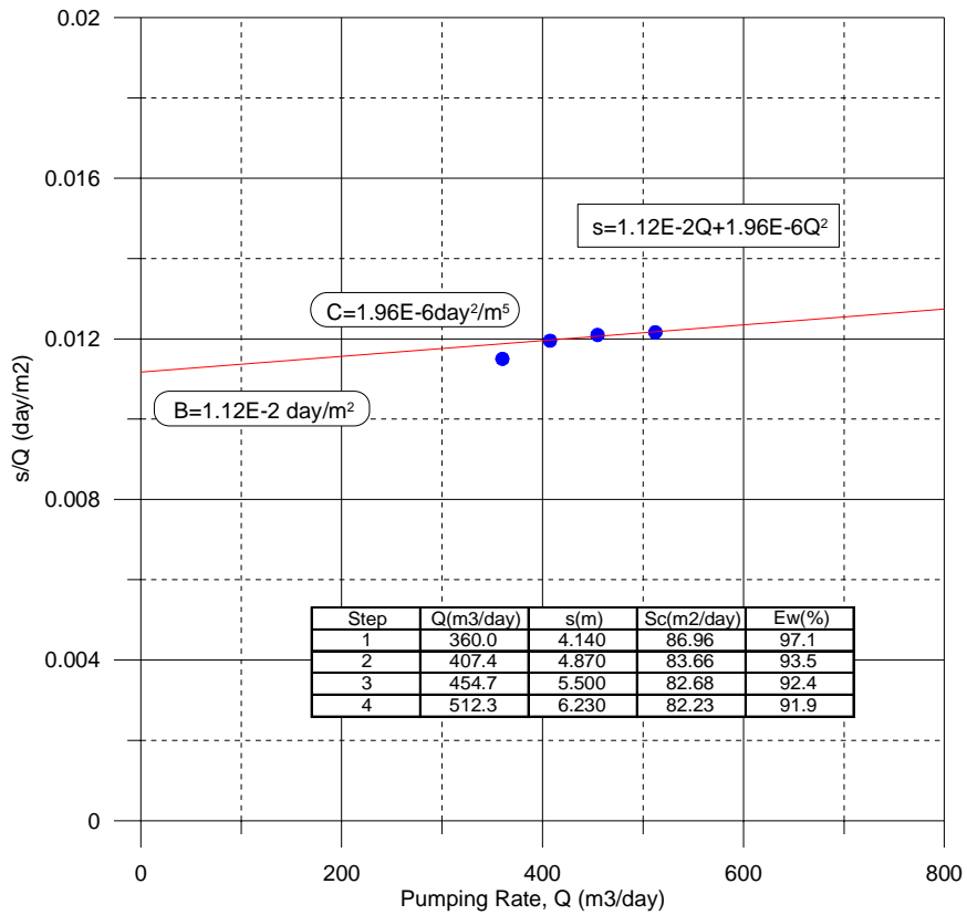
TM4_Diawara2 essai palier-2
