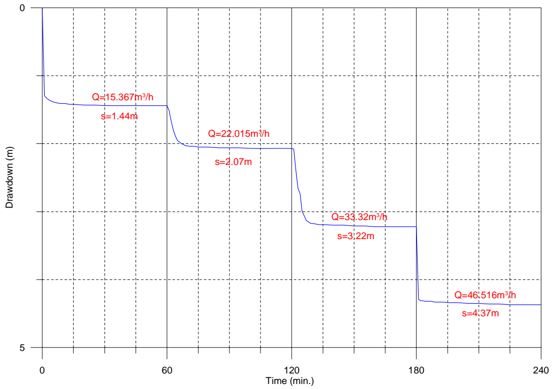
TM1_Ainou Mahdyessai palier-1
