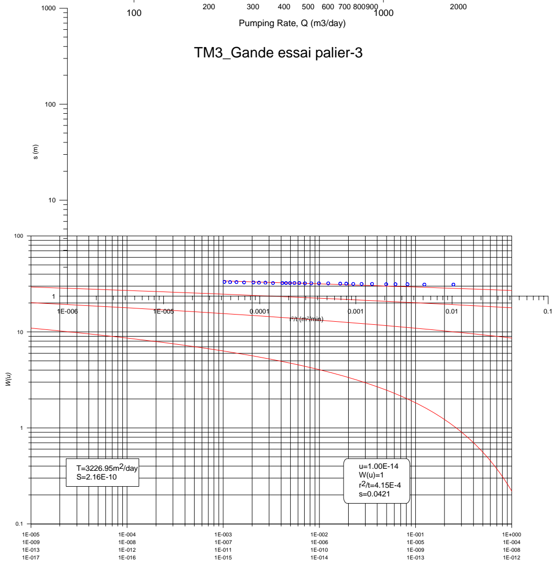
TM3_Gande Theismethode
