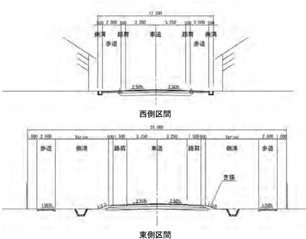
図 3-2-7 ベンベラ道路の標準横断面図
