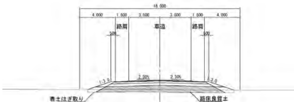
図 3-2-2 LS-MFEZ アクセス道路（高圧電力線沿線～LS-MFEZ ゲート区間）の標準横断面図（側溝無し）
