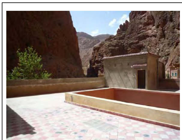
洪水警報設置予定地点（Toudgha 渓谷）
