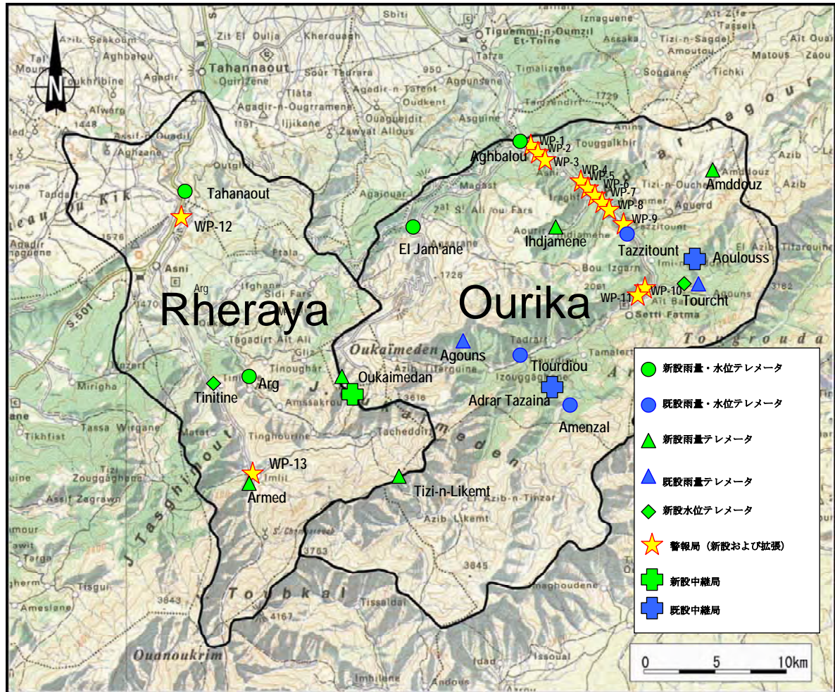
図 3-2 テレメータ水文観測所・警報局および中継局の配置計画図
