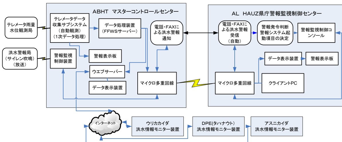
図 3-3 ウリカ川・レラヤ川流域洪水予警報システム情報フロー図
