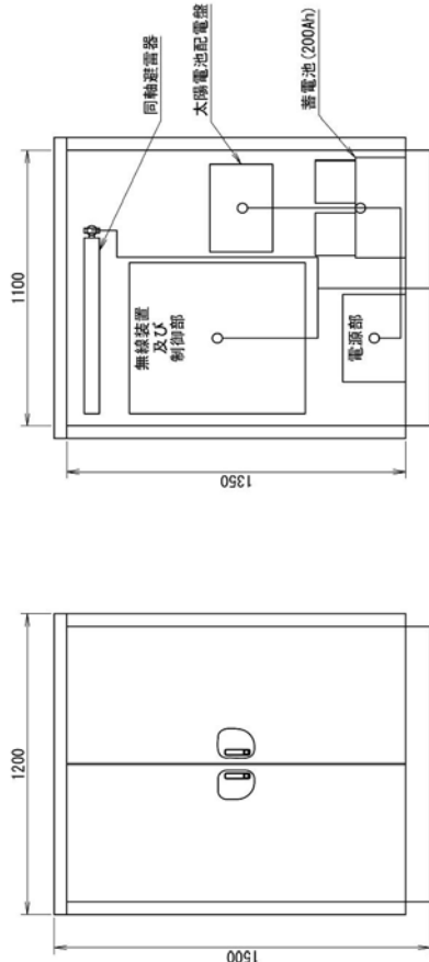
機器据付図 (S=1/20)
