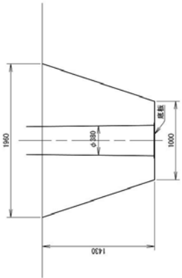
ハンガマスト埋設図 (R48) (S=1/40)
