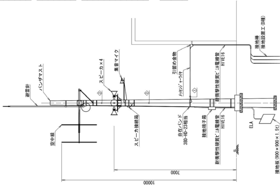
立面図 (S=1/80)
