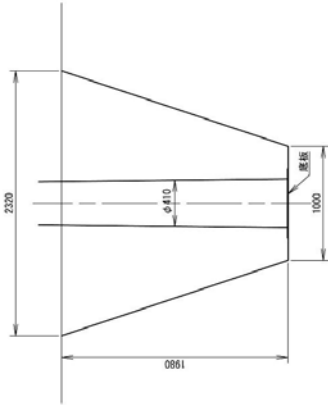
ハンガマスト埋設図 (R39) (S=1/40)
