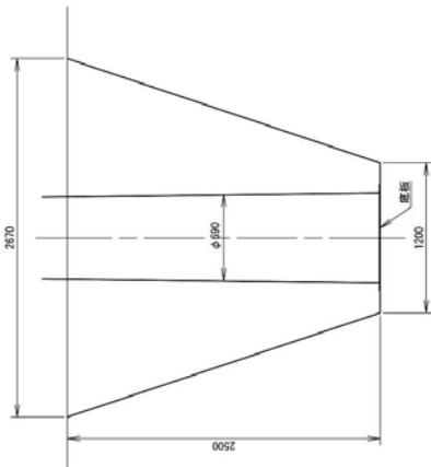
ハンガマスト埋設図 (R317) (S=1/40)
