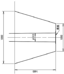
ハンガマスト埋設図 (R26) (S=1/40)
