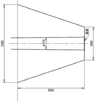
ハンガマスト埋設図 (R28) (S=1/40)
