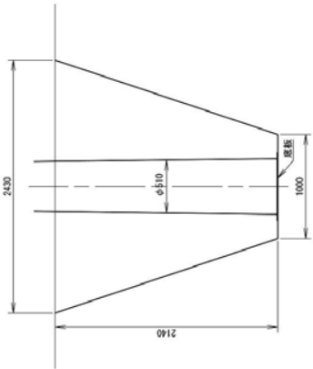
ハンガマスト埋設図 (R512) (S=1/40)
