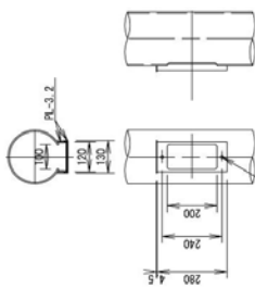
開口部詳細図 (S=1/20)
