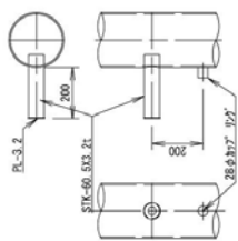
温度計取付部詳細図 (S=1/20)
