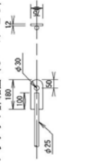
プレート詳細図 (S=1/20)
