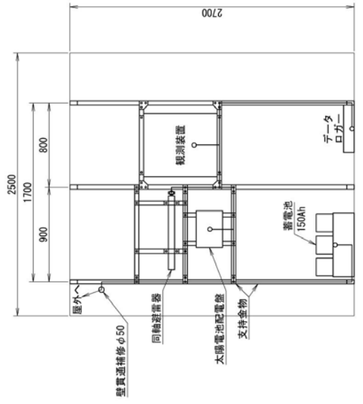
局舎内立面図 (S=1/30)
