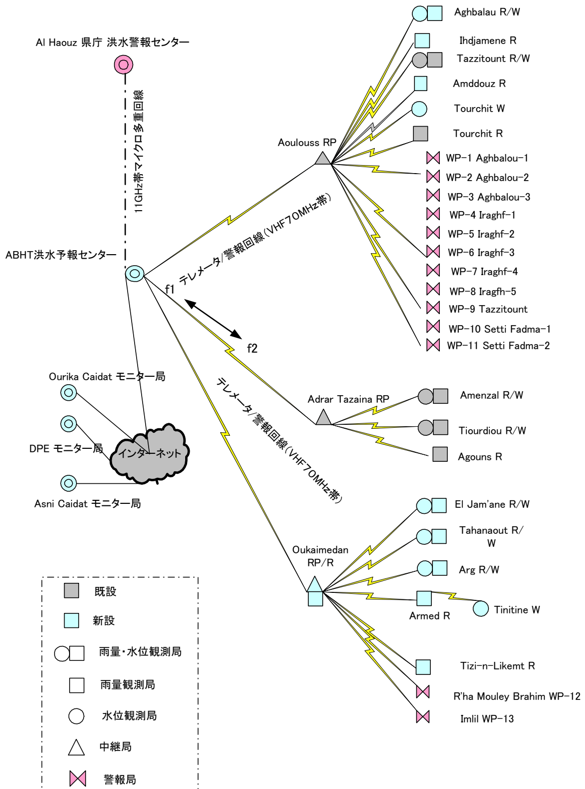
図 3-4 ウリカ川・レラヤ川流域洪水予警報システムネットワーク概念図
