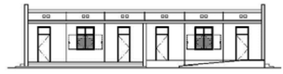
正面 立面図 Front Facade Elevation
