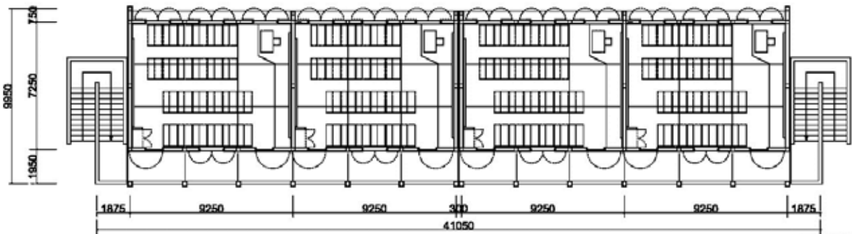
2階 平面図 2nd Floor Plan
