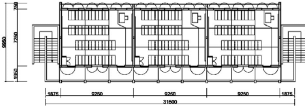
2階 平面図 2nd Floor Plan
