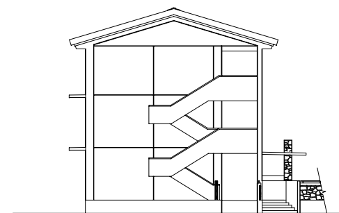
妻側立面図
