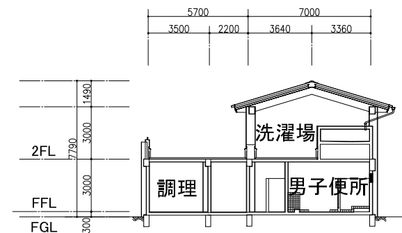
断面図
