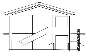
妻側立面図
