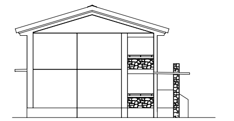
妻側立面図 (タイプ2-6A#2)
