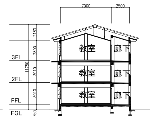
断面図
