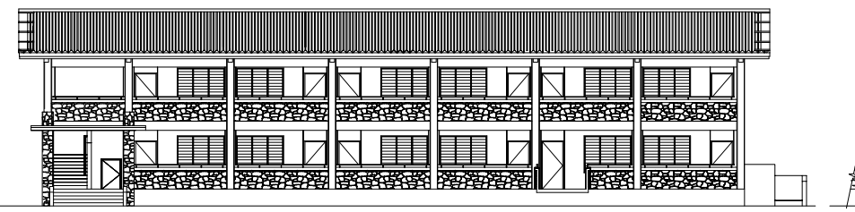
廊下側立面図(タイプ2-6A#2)
