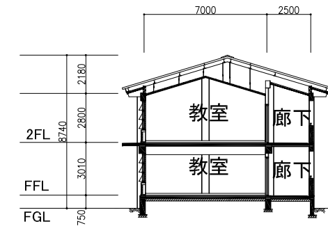
断面図(タイプ2-6A#1)
