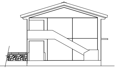
妻側立面図 (タイプ2-6A#1)
