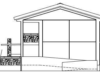
妻側立面図 (タイプ2-6A#2)
