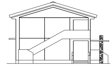
妻側立面図(タイプ2-4A)
