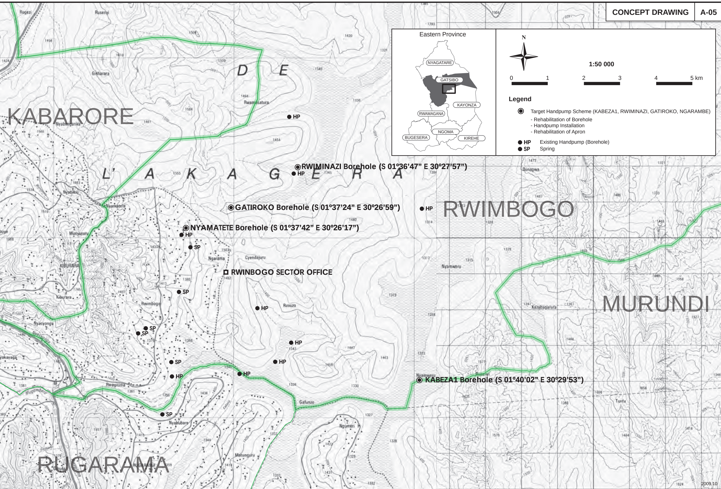
図3-13 優先プロジェクト計画概略図：PP05 RWIMBOGO
