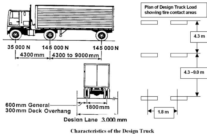
図 2-1-2 活荷重（HS20）
