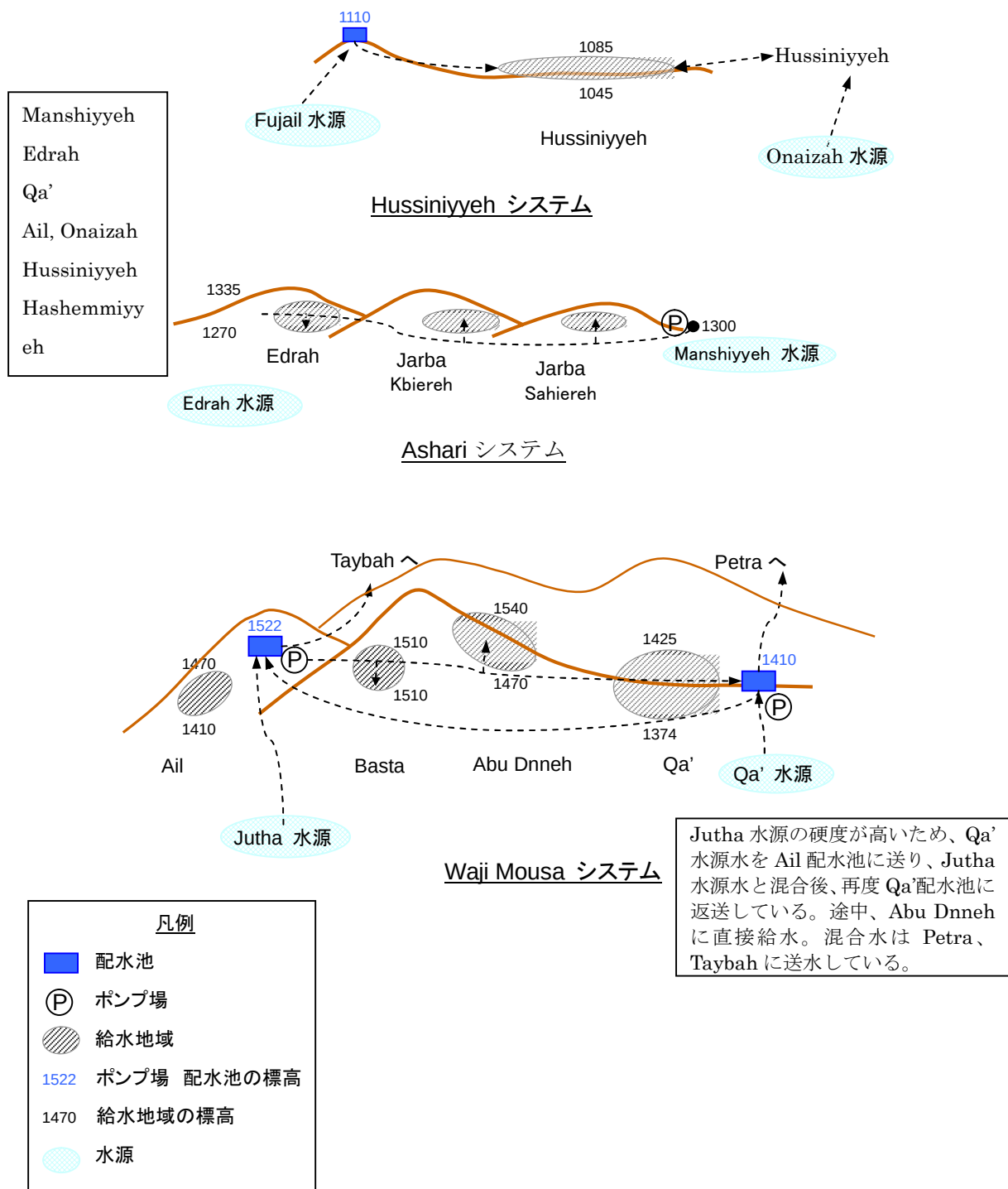
図ー2 対象地区の水道システムの模式図
