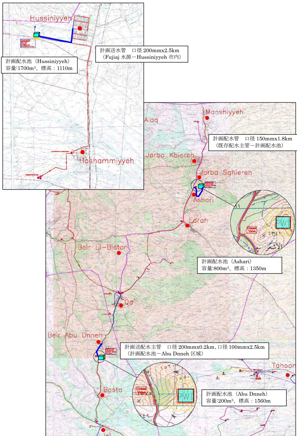
図－3 計画配水池及び送配水主管
