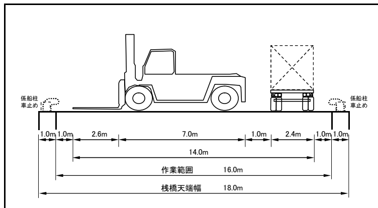
図 3.2.2-6(c) 栈橋上でのコンテナ荷役の状況
