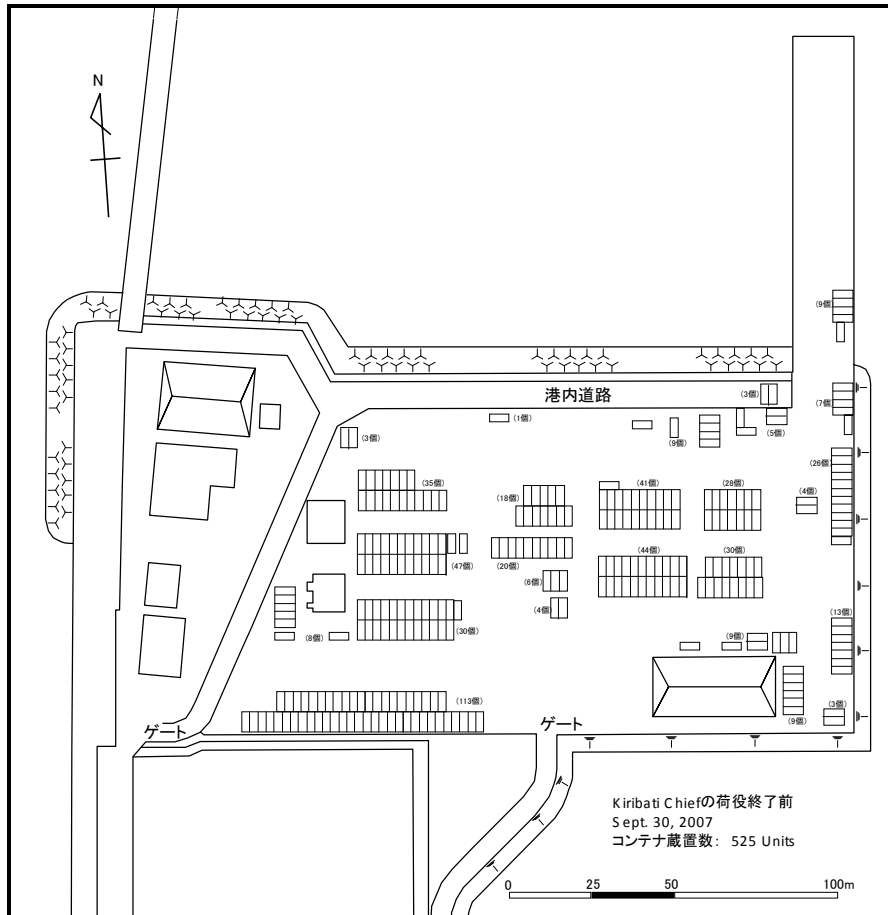
図 2.2.3-6 コンテナの蔵置状況(2007/09)
