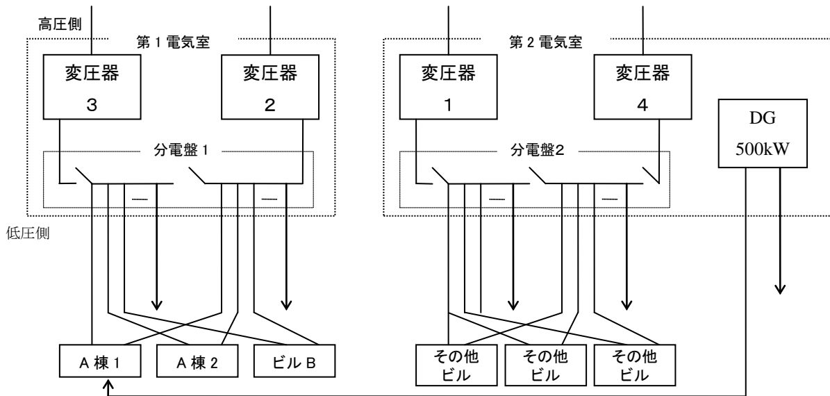
図 2-1-4-2 受電システム概念図
