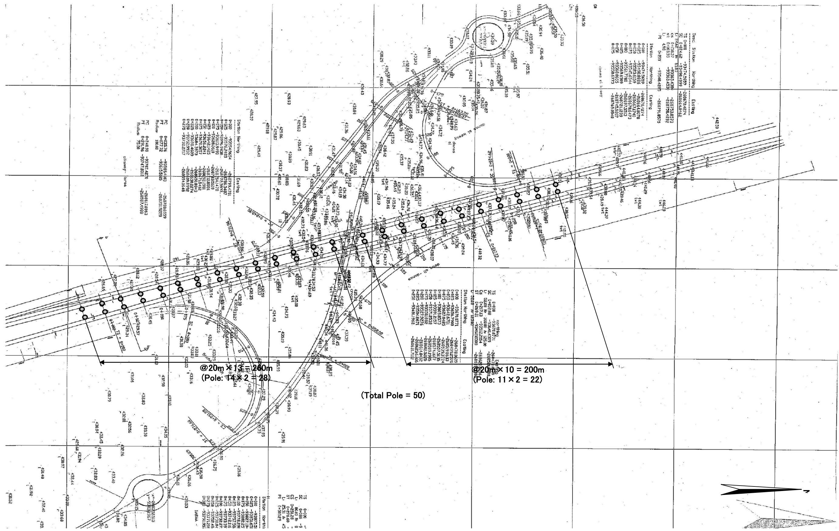
図3-6 Dear Ali インターチェンジ街灯配置図
