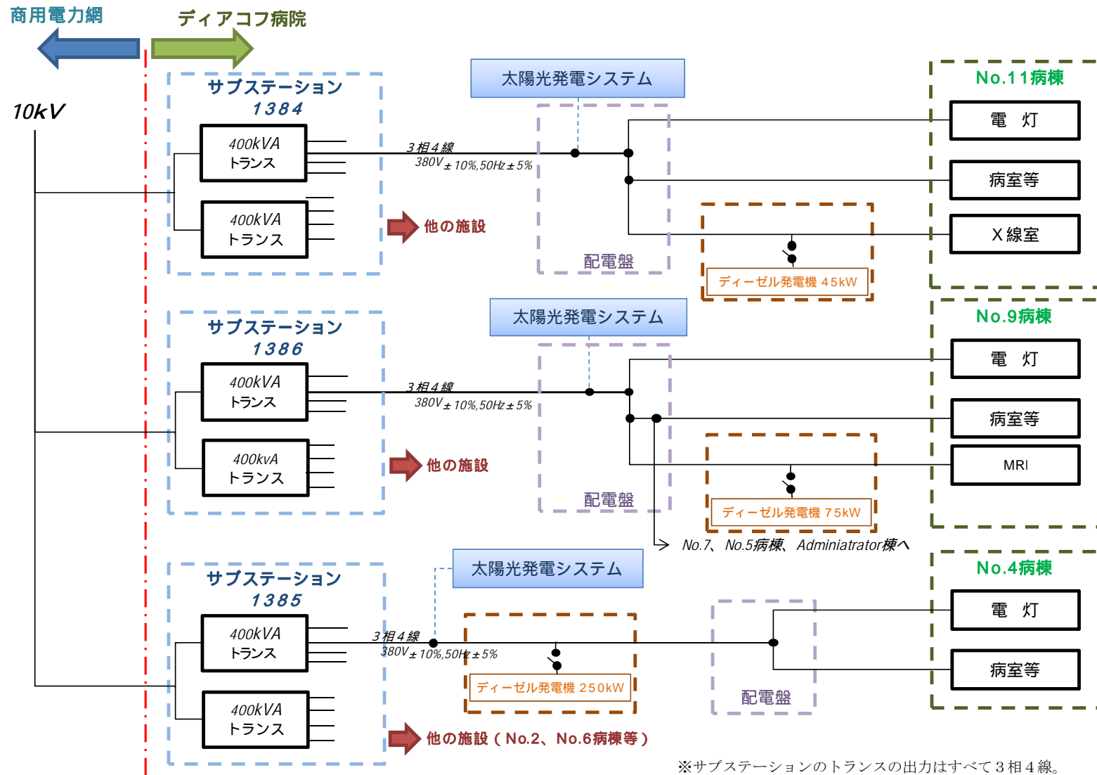
図 3-2 ディアコフ病院配電概要図
