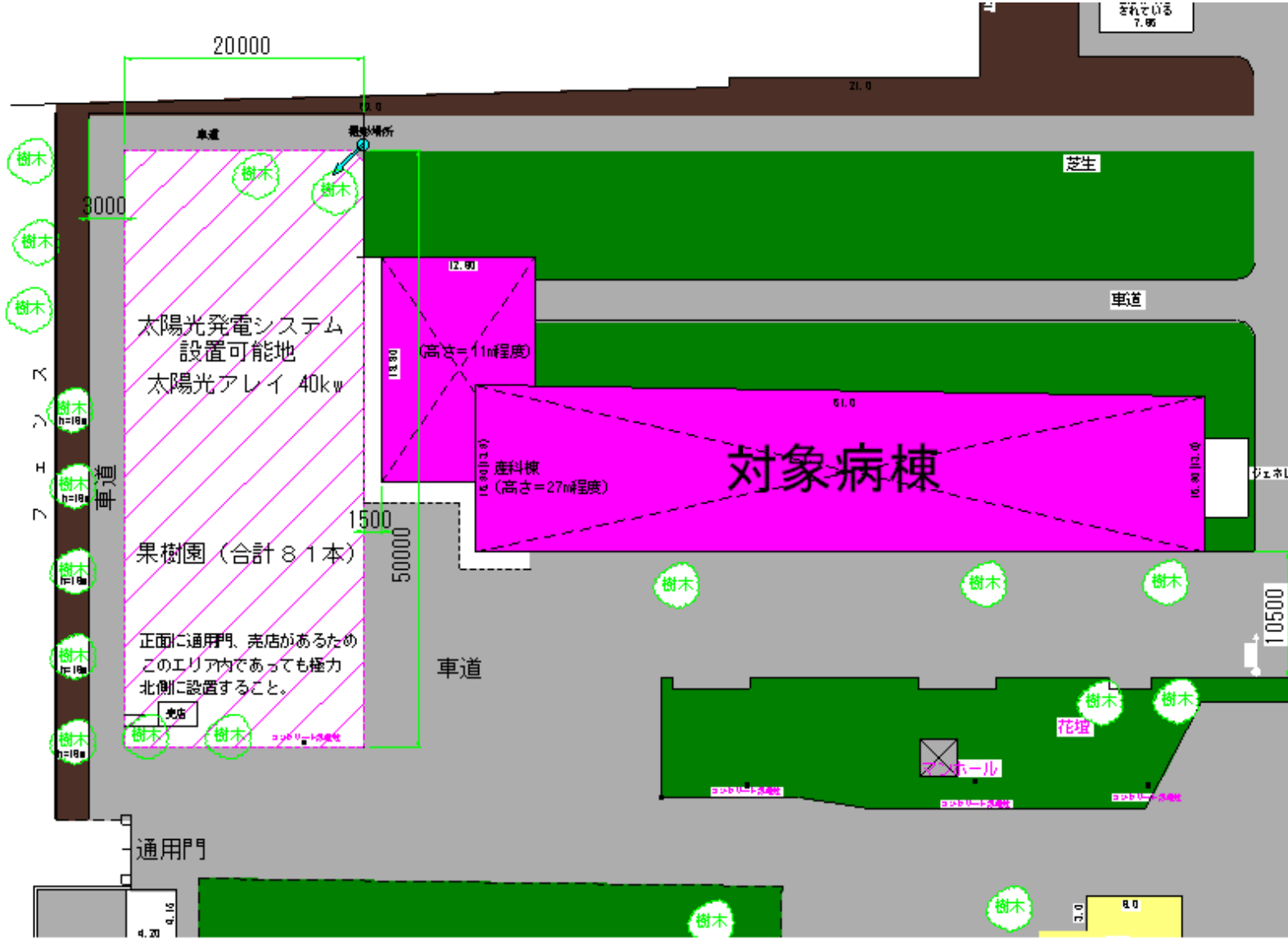
(2) 産科婦人科研究所 太陽電池アレイ配置図
