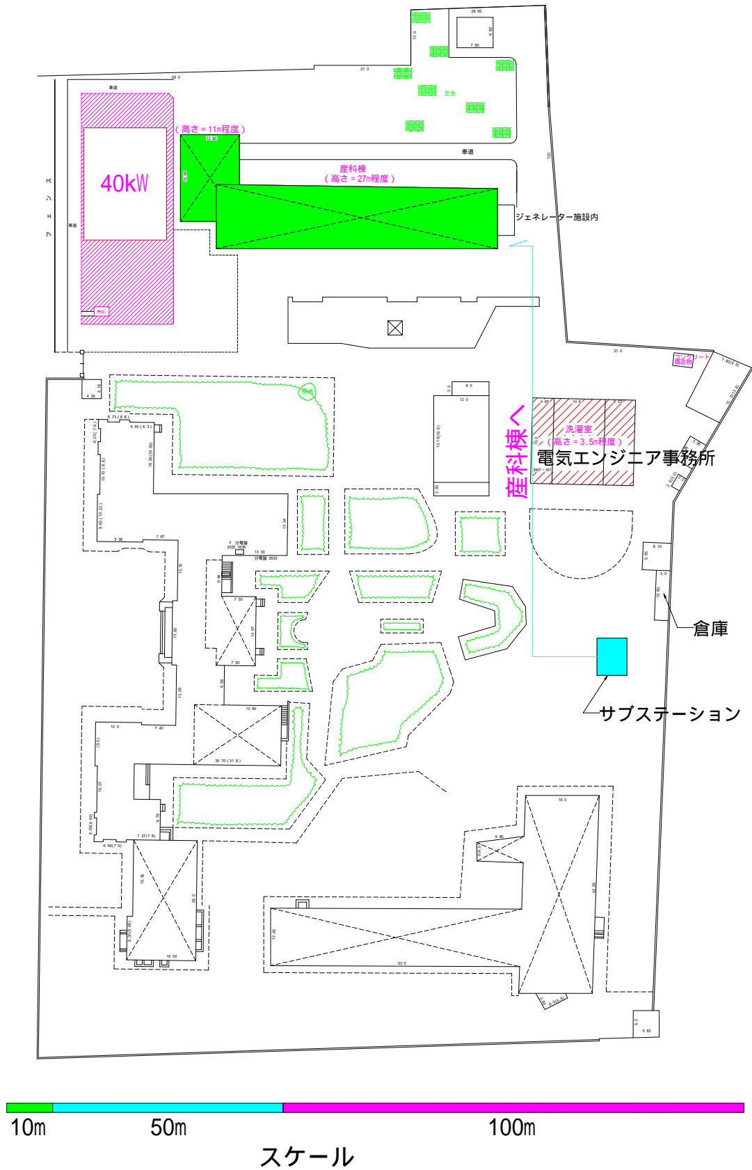
図 3-5 産科婦人科研究所配電図
