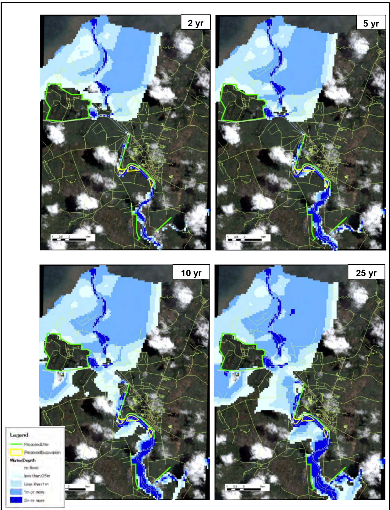
図 7.6 洪水氾濫計算結果 (With Alt-I2)
