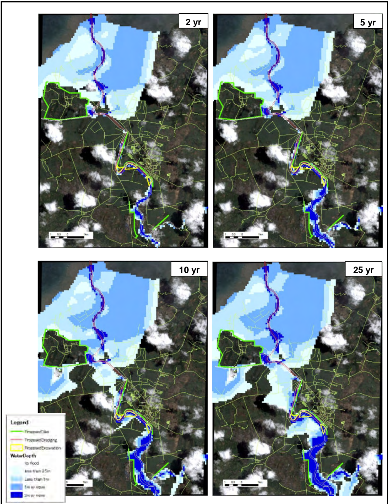
図 7.7 洪水氾濫計算結果 (With Alt-I3)
