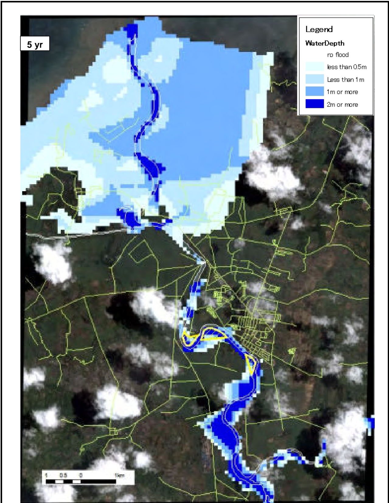
図 7.5 (2/6) 洪水氾濫計算結果 (Without Project)
