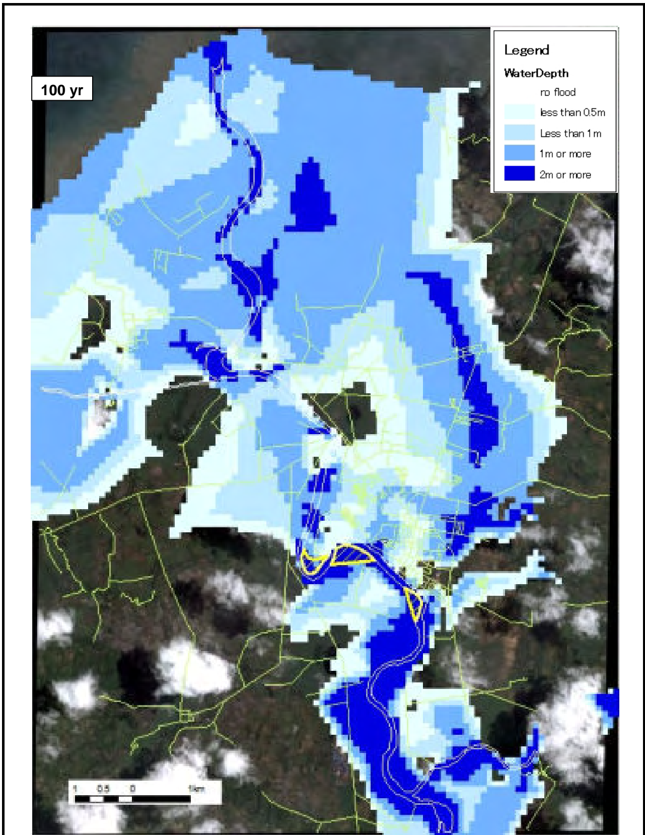
図 7.5 (6/6) 洪水氾濫計算結果 (Without Project)
