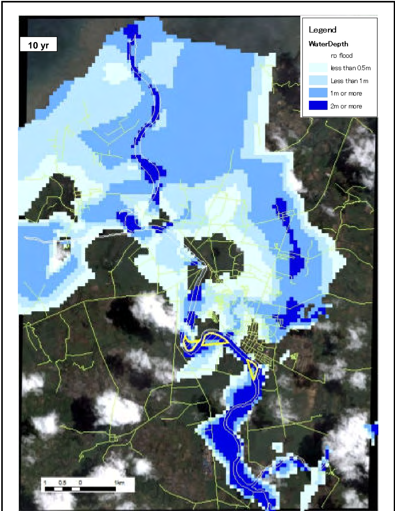
図 7.5 (3/6) 洪水氾濫計算結果 (Without Project)
