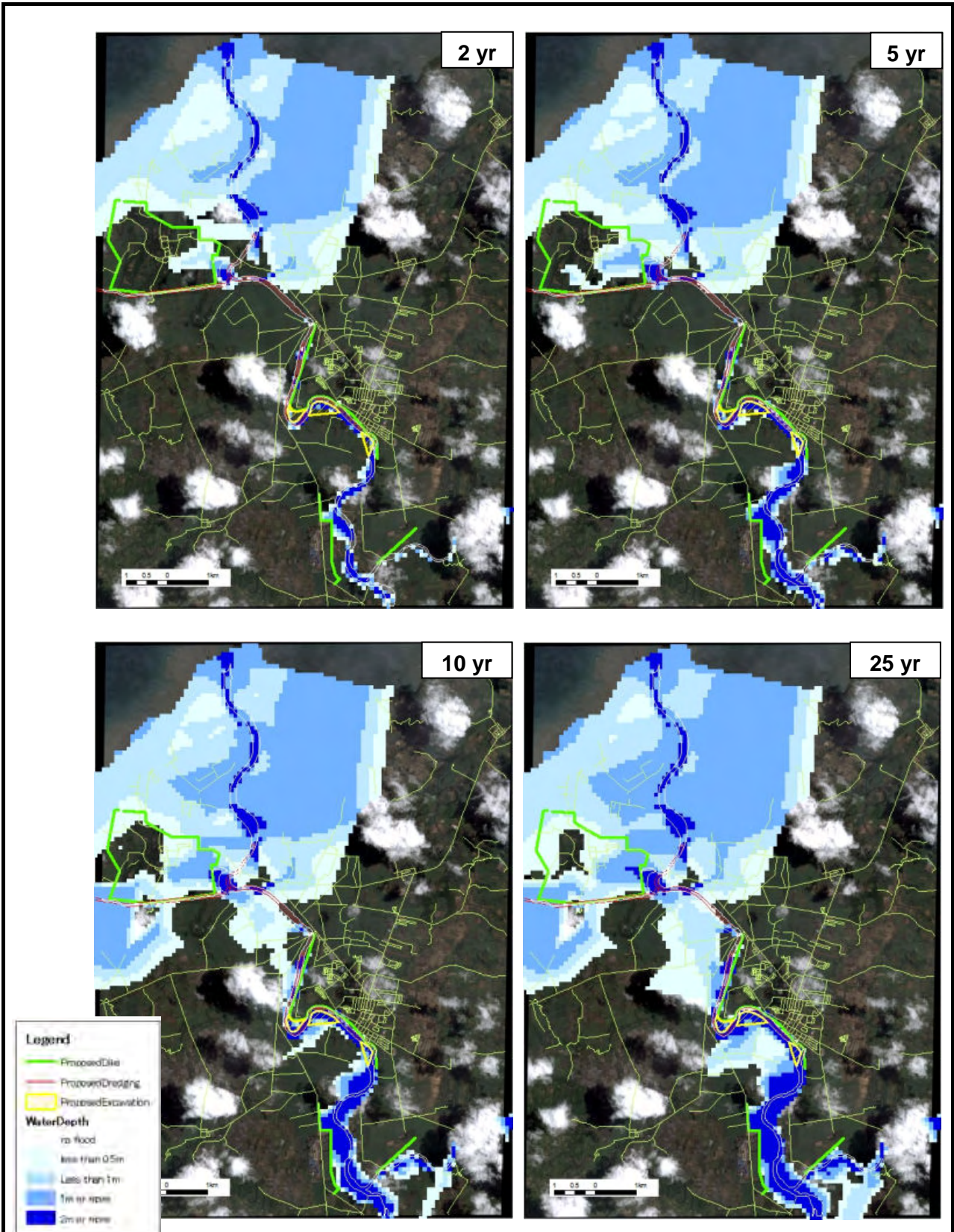
図 7.8 洪水氾濫計算結果 (With Alt-I4)
