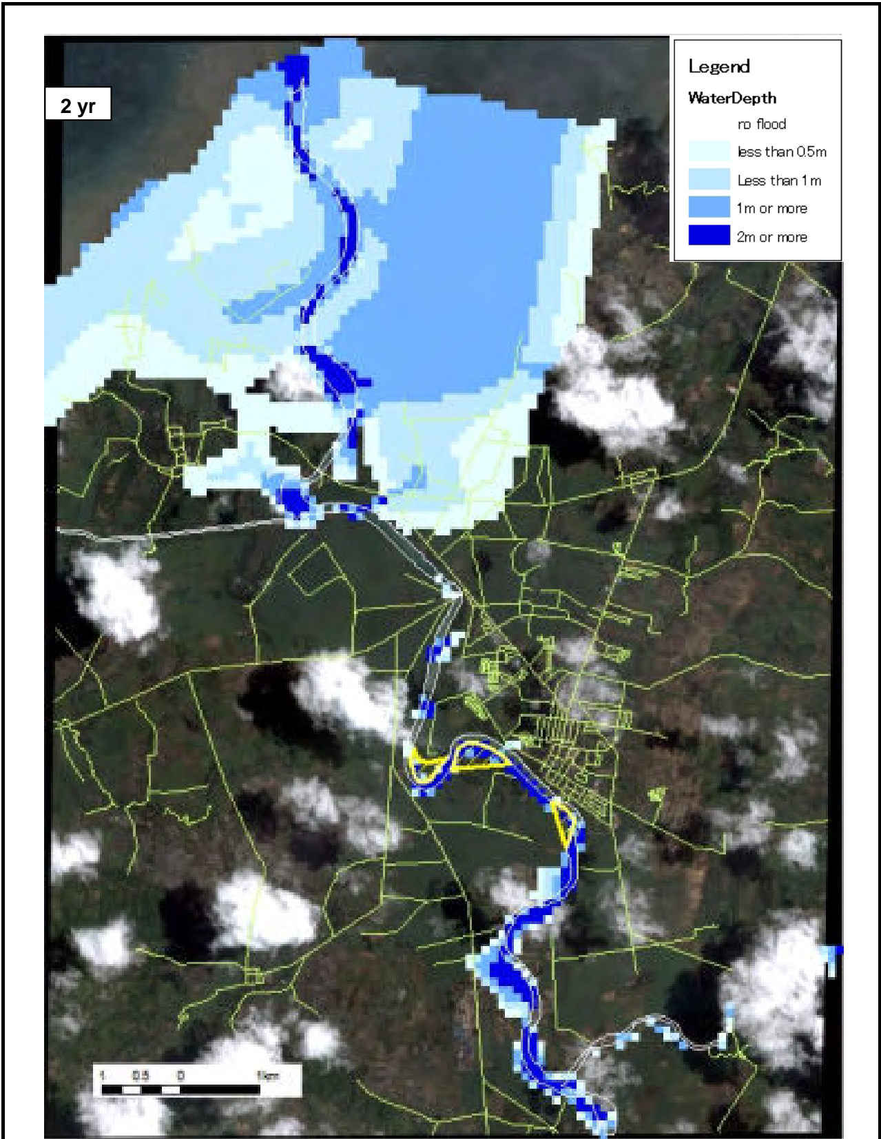
図 7.5 (1/6) 洪水氾濫計算結果 (Without Project)
