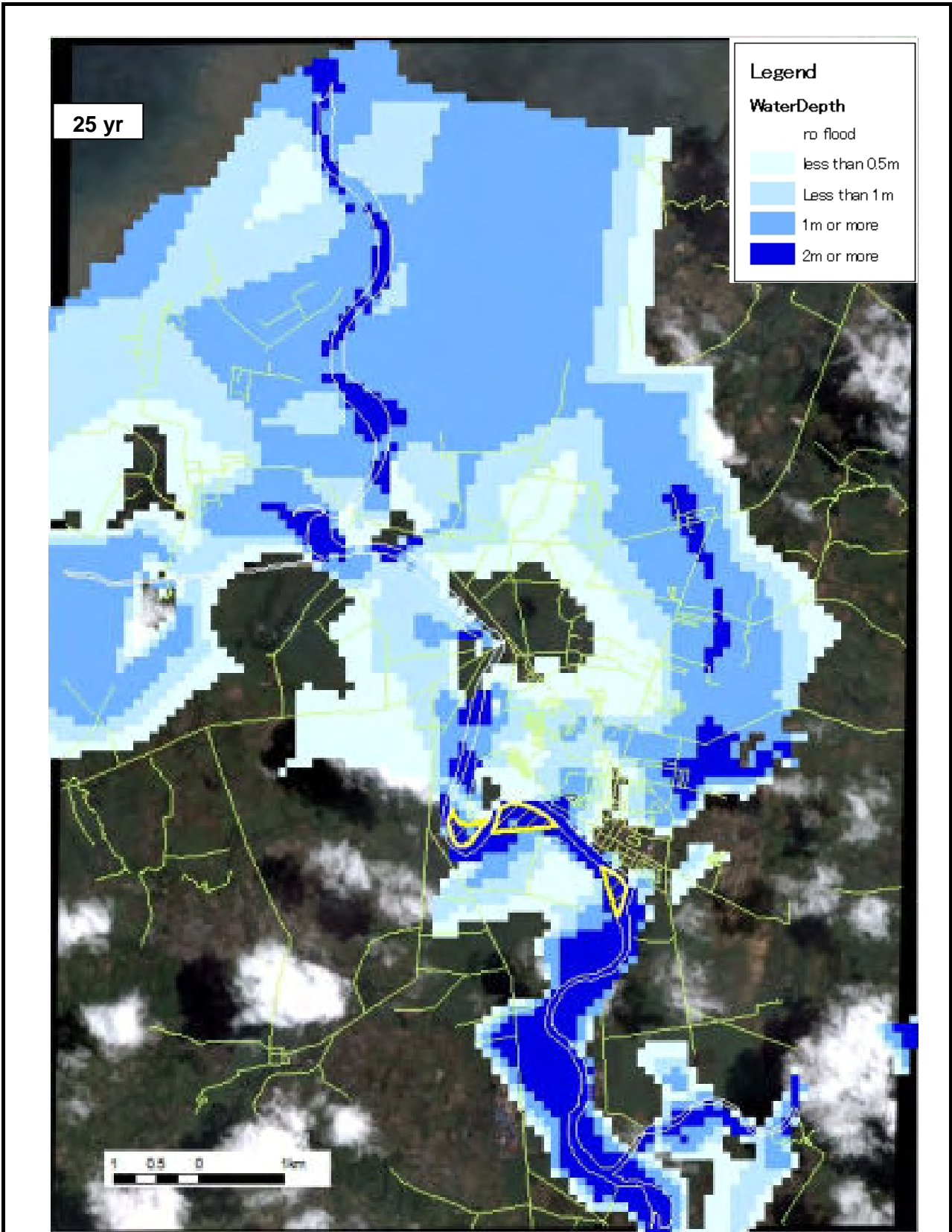
図 7.5 (4/6) 洪水氾濫計算結果 (Without Project)
