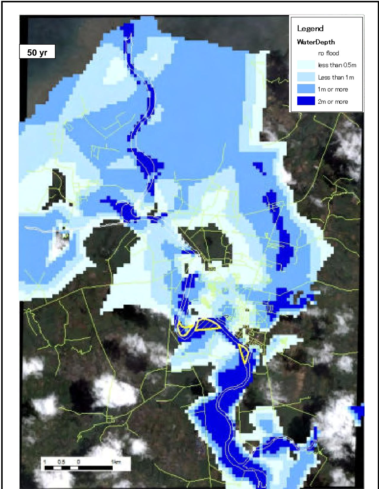
図 7.5 (5/6) 洪水氾濫計算結果 (Without Project)
