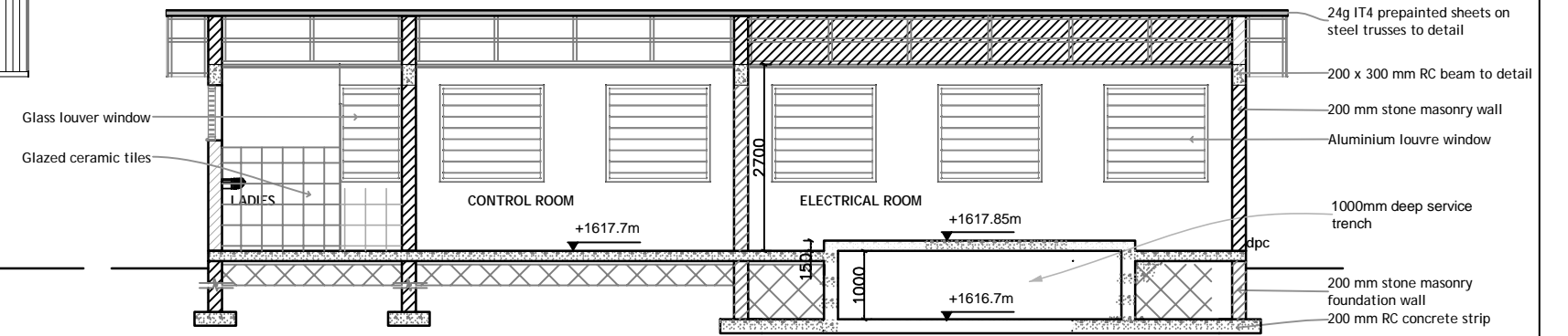
SECTION A-A
