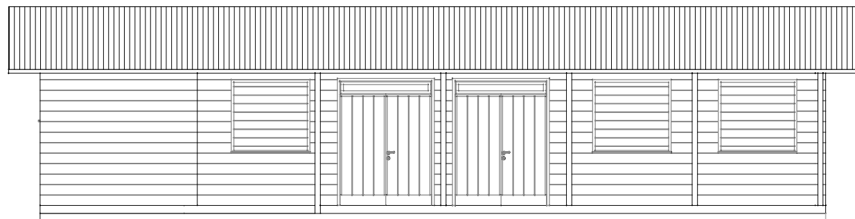
ELEVATION 01
