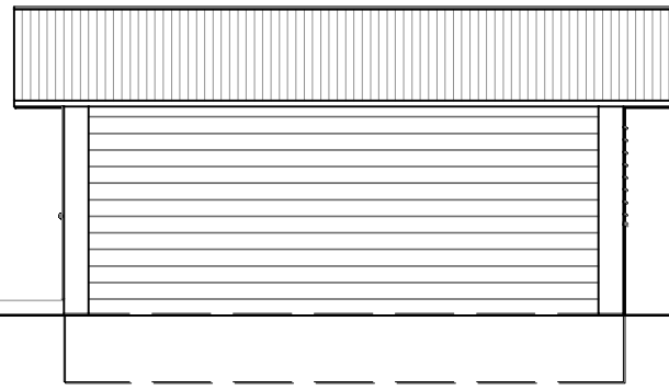
ELEVATION 01
