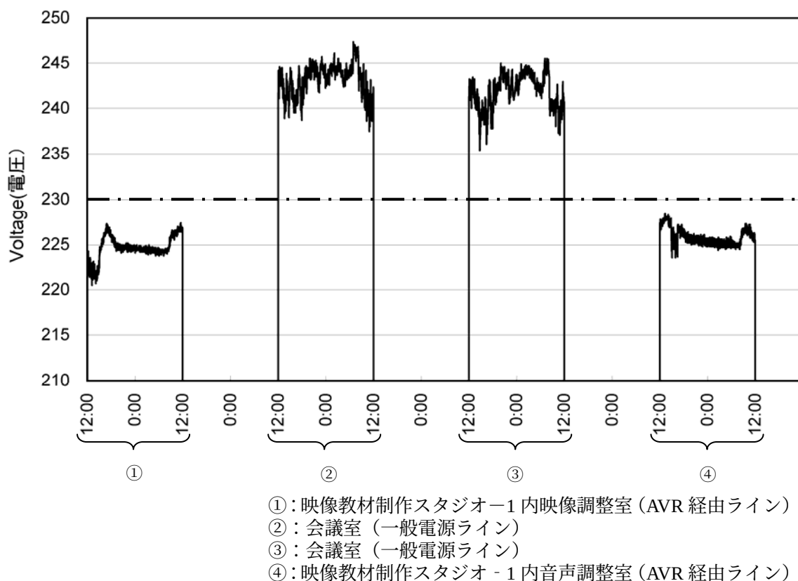
図 3-7 電圧変動グラフ
