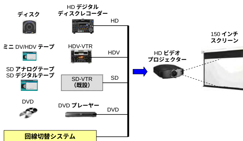
映像教材評価 プロセスチャート
