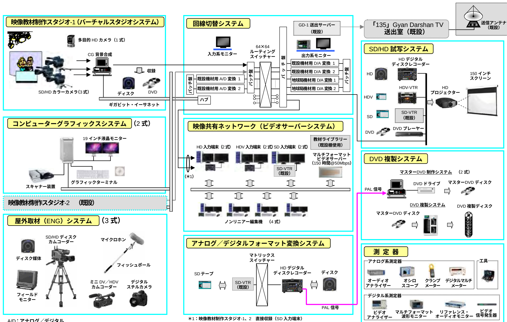
図 3-1 協力対象事業のシステム全体概要図
