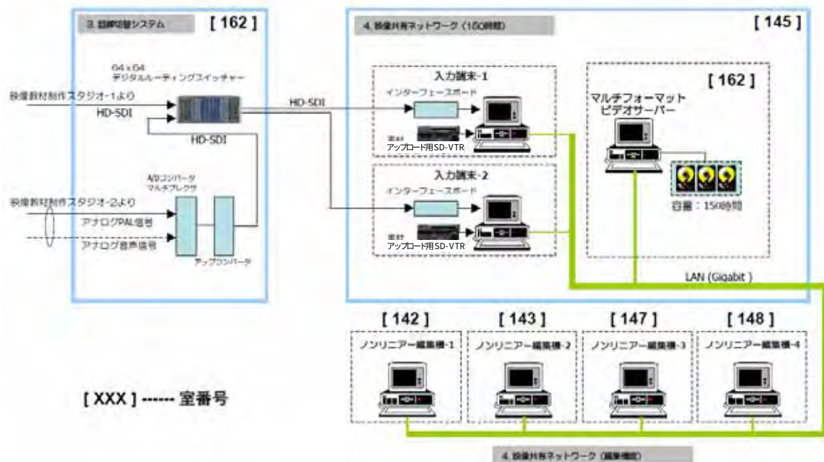
図 3-5 リアルタイム収録の概念図
