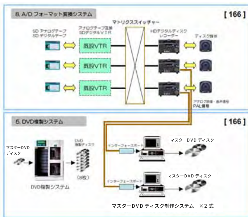
図 3-6 マスターDVD ディスク制作システム
