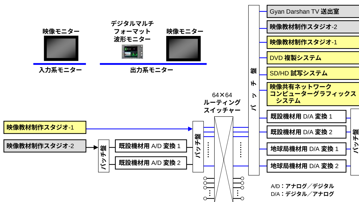
室間接続切替 プロセスチャート
