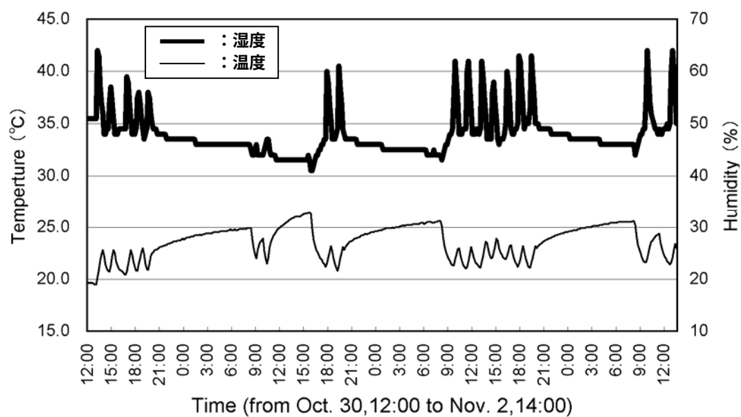
図 3-9 温度・湿度グラフ [音声教材制作スタジオ-1 内音声調整室 室番「108」]
