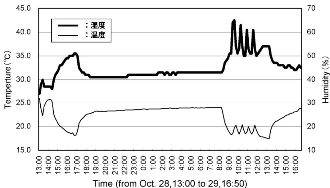
図 3-8 温度・湿度グラフ [映像機材制作スタジオ1 内音声調整室 室番「124」]
