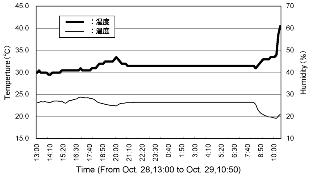
図 3-11 温度・湿度グラフ [シングルステップ編集室-1 室番「139」]
