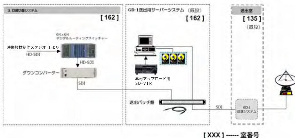
図 3-4 GD-1 への送出概念図
