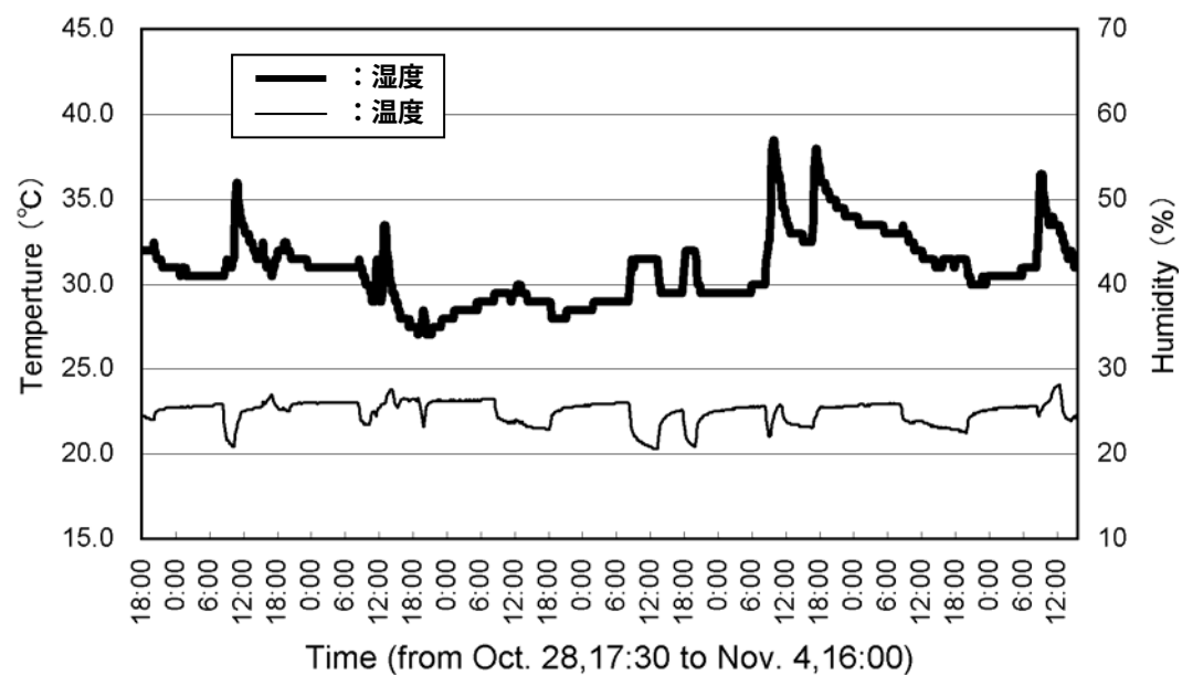
図 3-10 温度・湿度グラフ [複製室 室番「166」]
