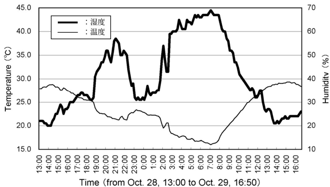
図 3-13 温度・湿度グラフ [外気温・湿度(中庭)]
