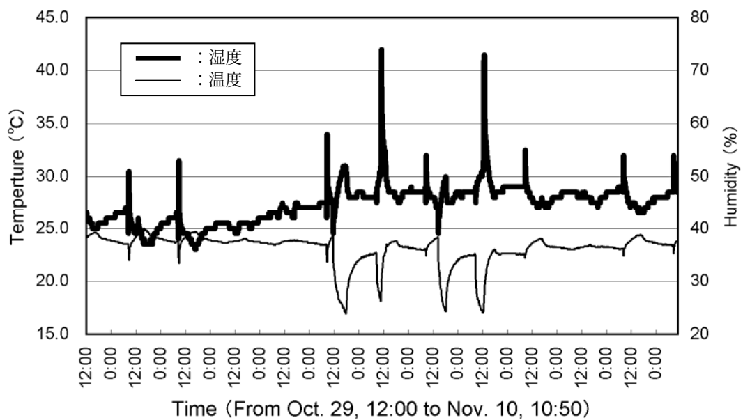
図 3-12 温度・湿度グラフ [サーバー入力／閲覧 CG 室-2 室番「146」]
