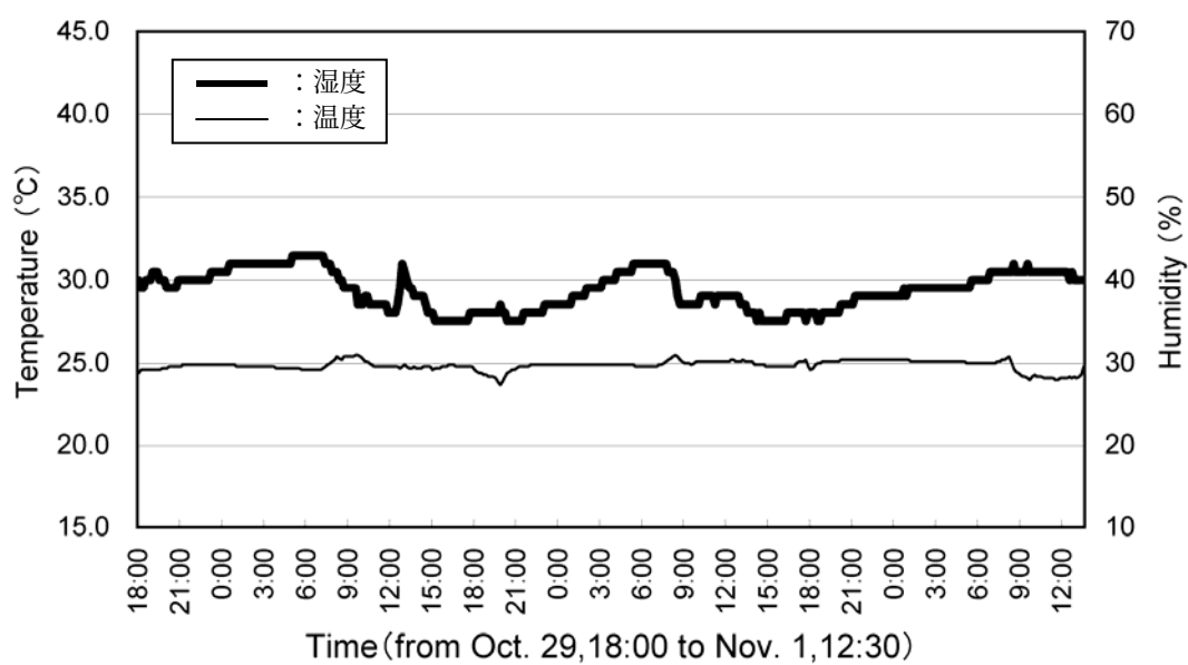
図 3-14 温度・湿度グラフ [会議室 室番「234」]
