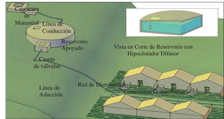
Gráfico N° 4.8.2-3: Sistema de Abastecimiento por Gravedad sin Tratamiento
