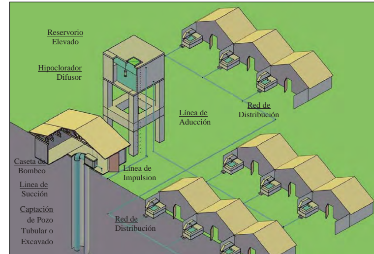
Gráfico N° 4.8.2-4: Sistema de Abastecimiento por Bombeo sin Tratamiento
