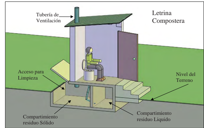
Gráfico N° 4.8.2-10: Letrina Compostera
