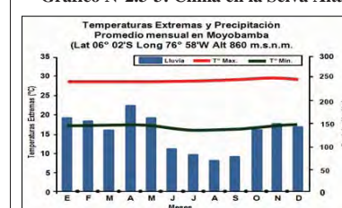
Gráfico N°2.3-3: Clima en la Selva Alta
