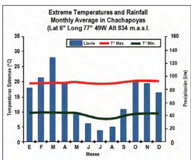
Gráfico N°2.3-4: Clima en la Ceja de Selva
