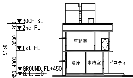
A-A' 断面図 S=1:400
