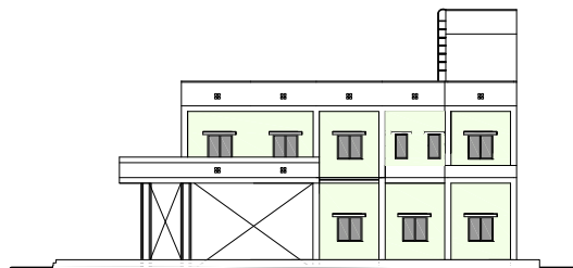
南側立面図 S=1:400
