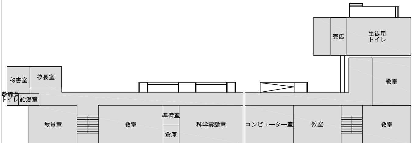
1階平面図 S=1:400
