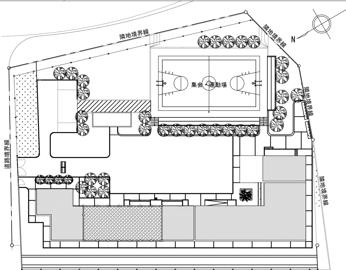
配置図 S=1:600
