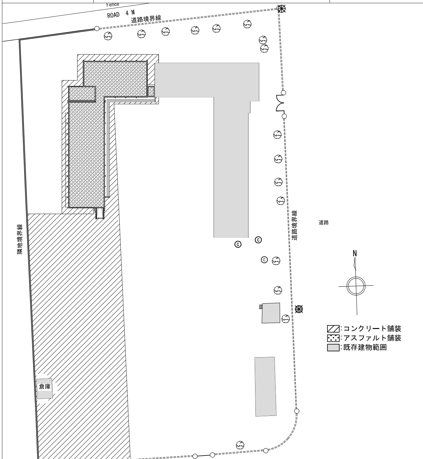
配置図 S=1:600
