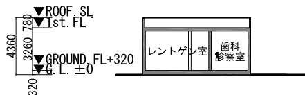
A-A' 断面図 S=1:400
