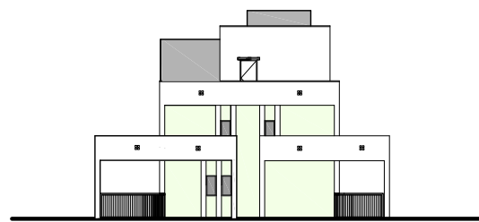
北側立面図 S=1:400
