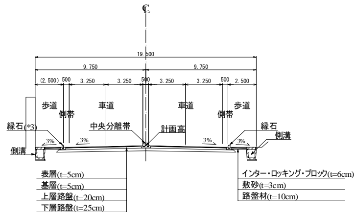
区間-4 標準横断図 (ヤナキス RA~スタンダードバンク IC)
