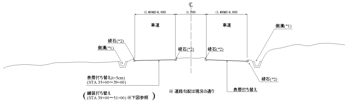
区間-3 標準横断図 (その1) (チチリ RA~マセレマ RA)
