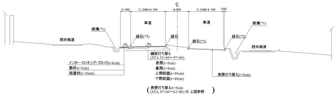
区間-3 標準横断図 (その2) (マセレマ RA~ヤナキス RA)
