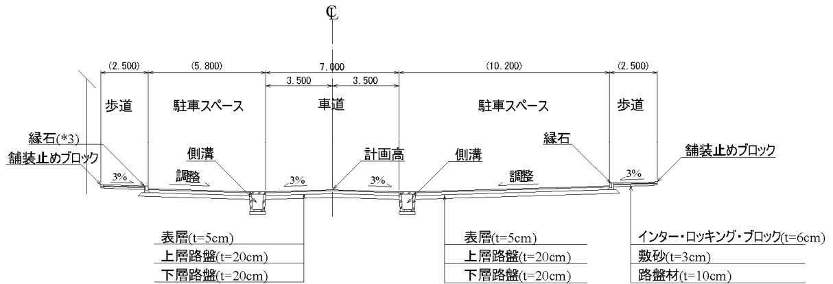
区間-5 標準横断面図 (スタンダードバンク IC~イロボ RA)
