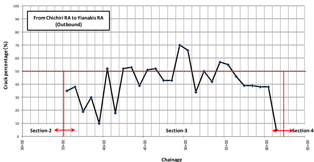
図 3-2(1) 区間-3 ひび割れ調査結果 (下り線側/チチリ⇒ヤナキス)
