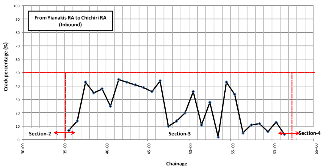
図 3-2(2) 区間-3 ひび割れ調査結果 (上り線側/ヤナキス⇒チチリ)
