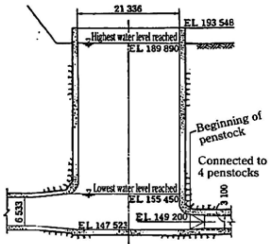
Fig. 47-1 1. Simple Type
