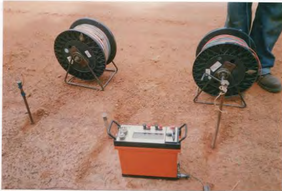
Trabajo de campo de Sondeos Eléctricos verticales
