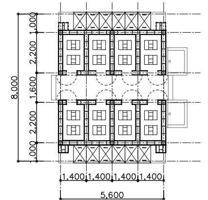
1階平面図
