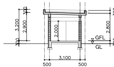
断面図 (短辺方向)
