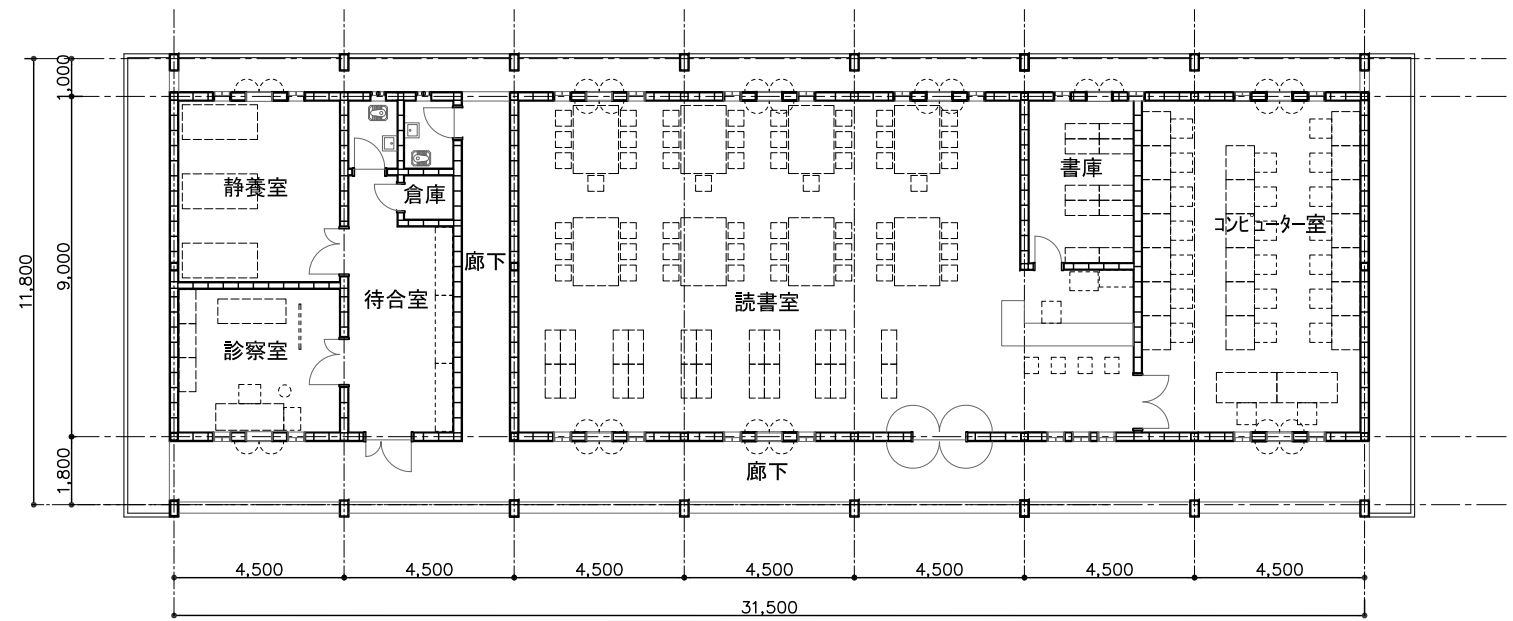
1階平面図
