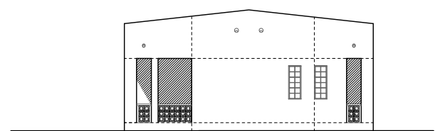
側面立面図 (南東面)
