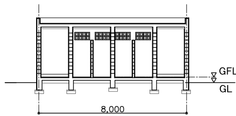
断面図 (長辺方向)
