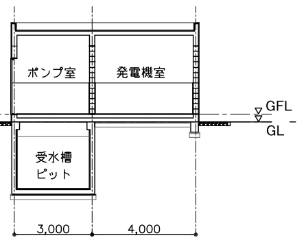
断面図 (長辺方向)
