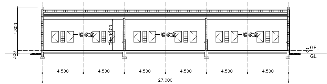
断面図 (長辺方向)
