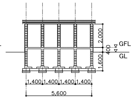
断面図 (短辺方向)
