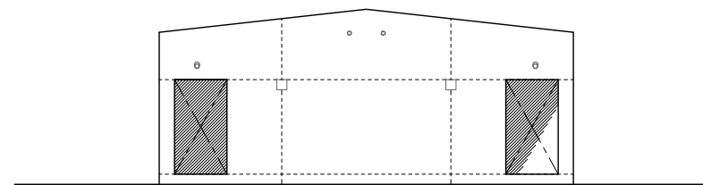
側面立面図 (北西面)
