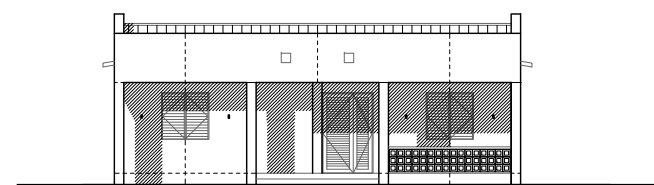
立面図 (南西面)
