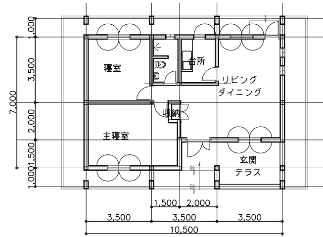
1階平面図
