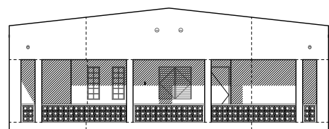
側面立面図 (南東面)
