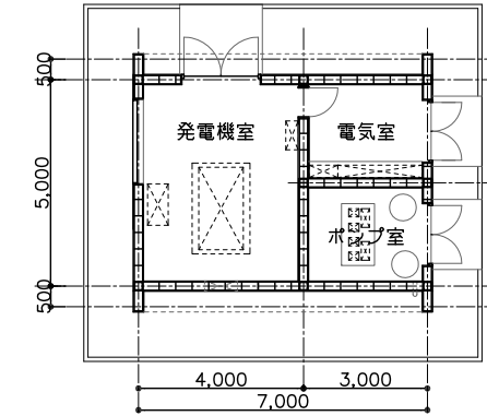
1階平面図
