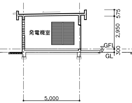
断面図 (短辺方向)
