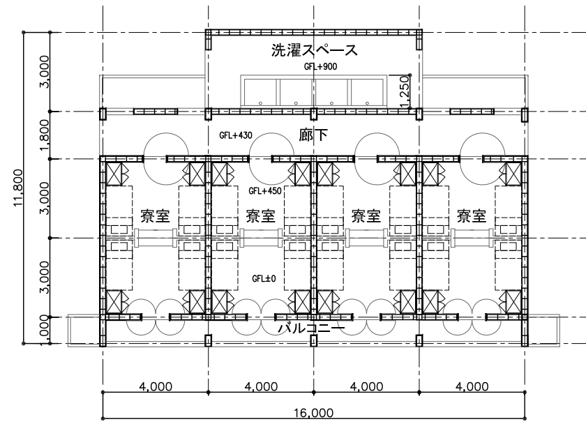
1階平面図
