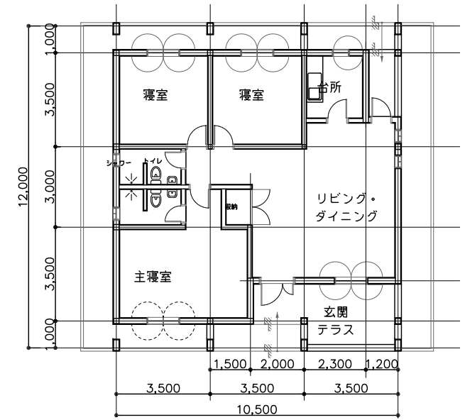
1階平面図
