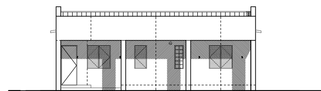
立面図 (北東面)
