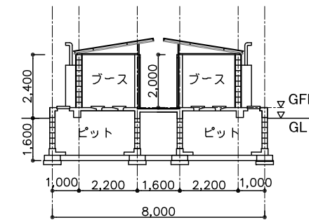
断面図 (長辺方向)
