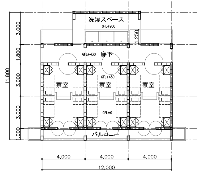
1階平面図
