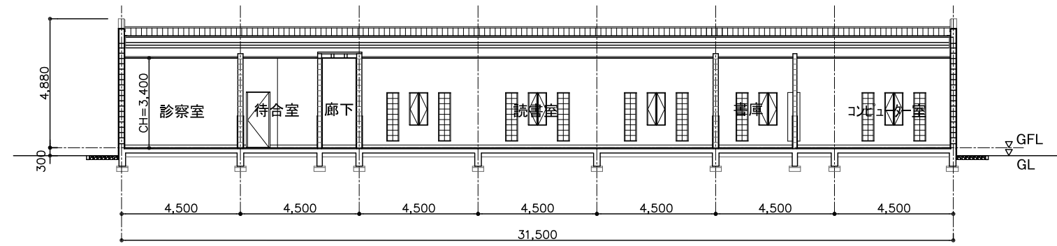
断面図(長辺方向)
