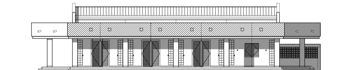
立面図 (北東面)
