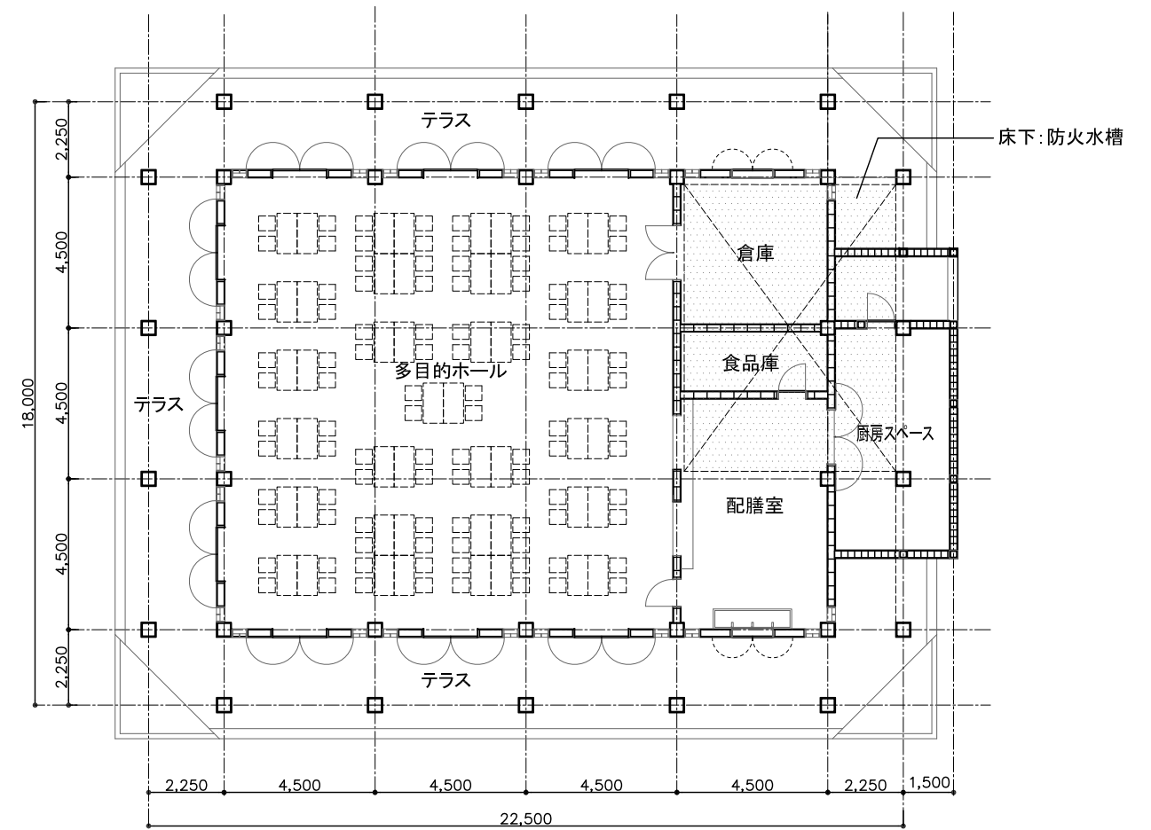
1階平面図
