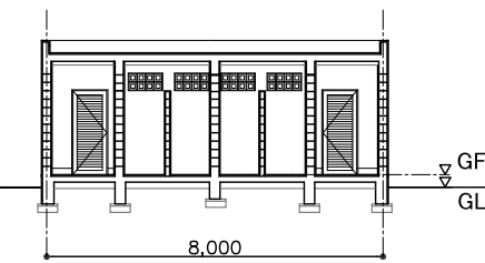
断面図 (長辺方向)
