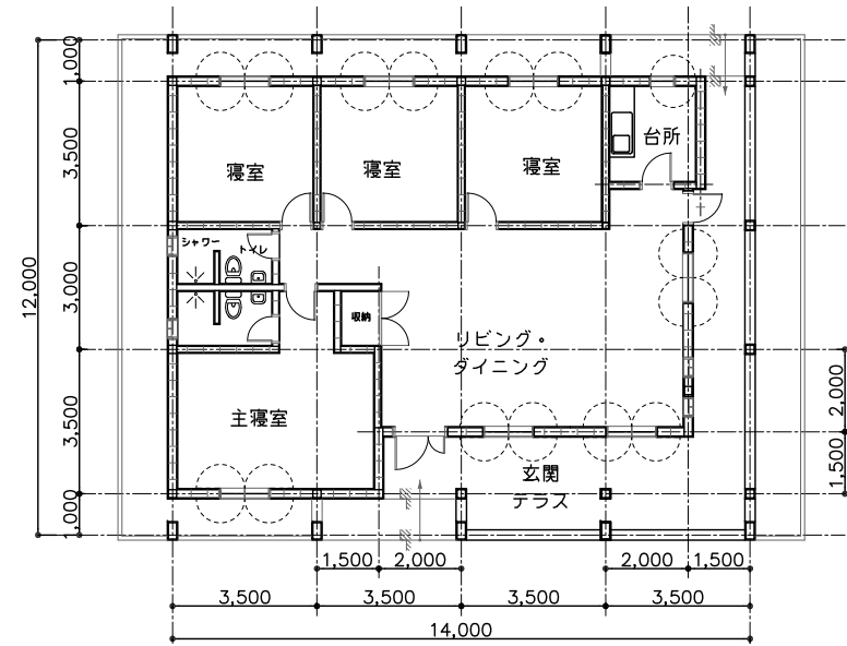
1階平面図
