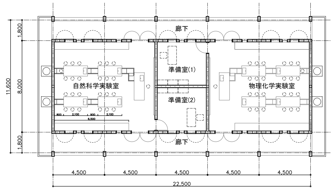
1階平面図
