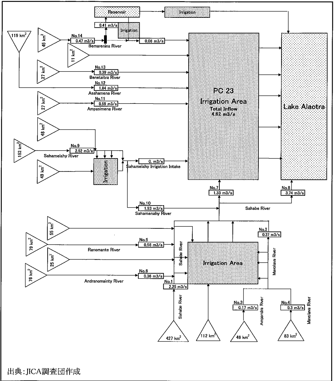
付図3.2 PC23流域の流量測定結果 (2003年10月8日より11日に測量)
