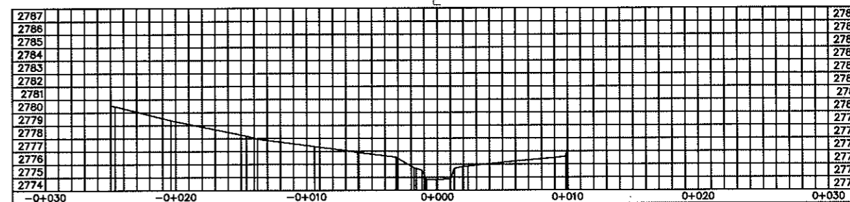
SECCION k0+005
