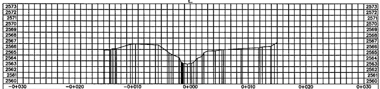
SECCION k0+110
