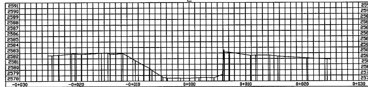
SECCION K0+030
