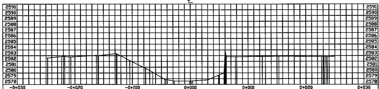
SECCION K0+040
