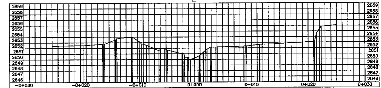
SECCION k0+035
