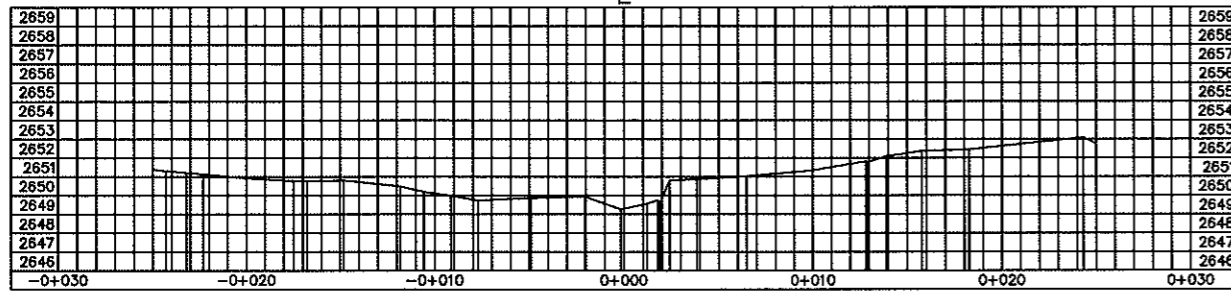
SECCION k0+000
