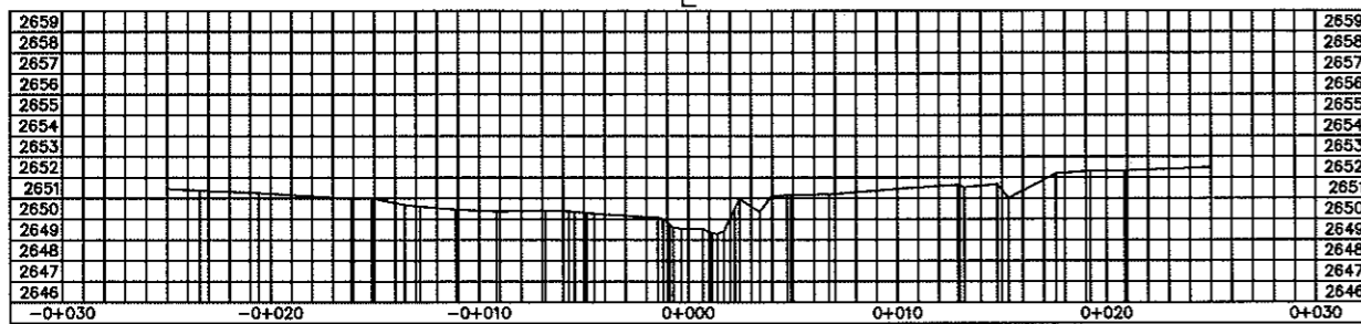
SECCION k0+010
