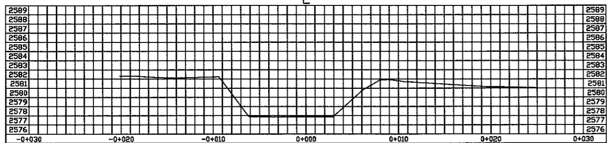
SECCION K0+000
