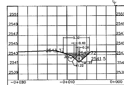
k3+481
