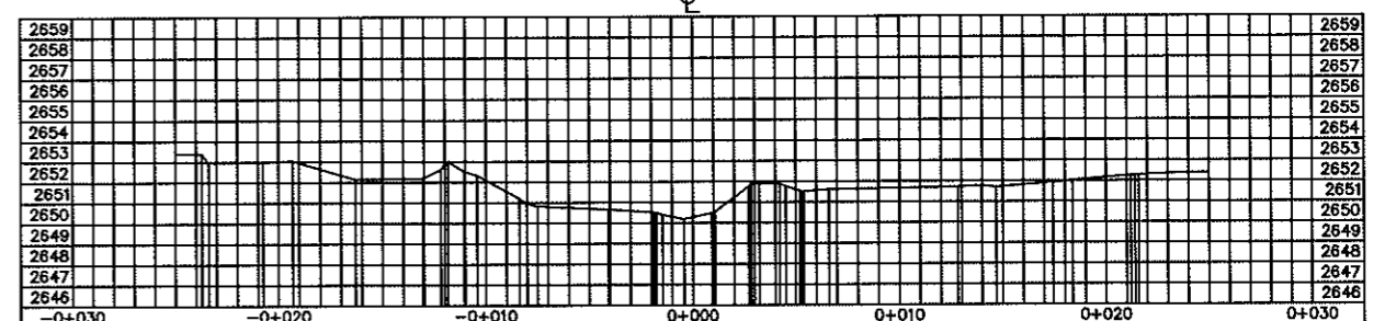
SECCION k0+025
