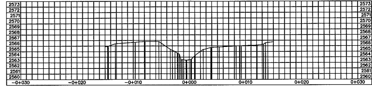
SECCION k0+100
