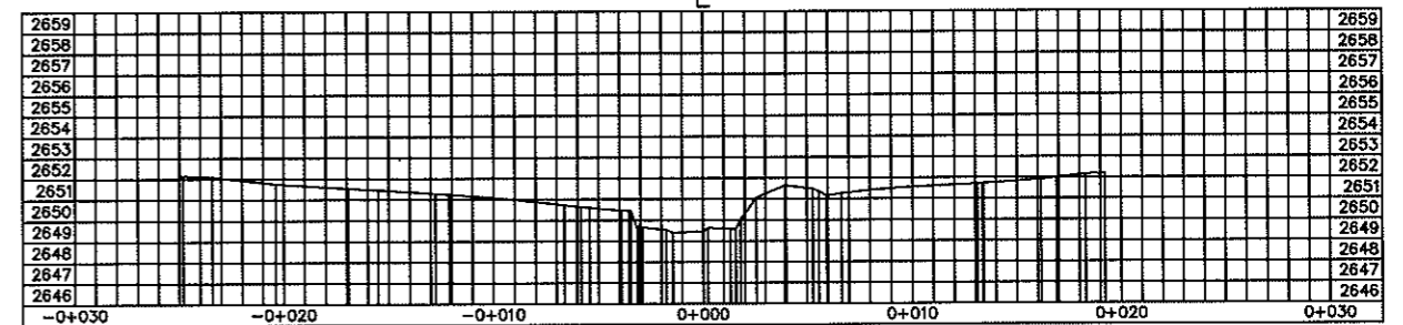
SECCION k0+015
