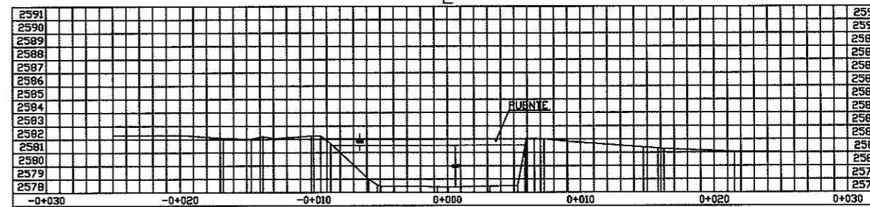
SECCION K0+010
