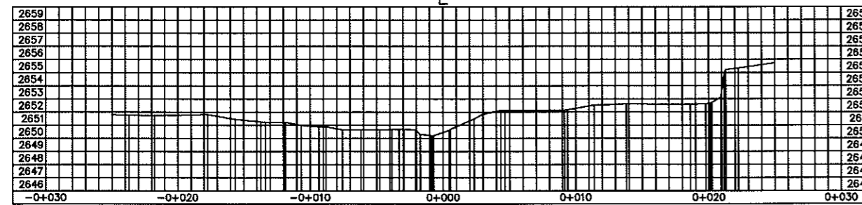
SECCION k0+030
