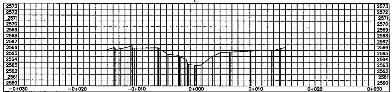
SECCION k0+090
