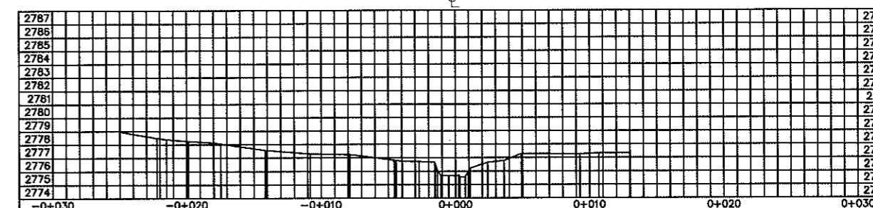
SECCION k0+025
