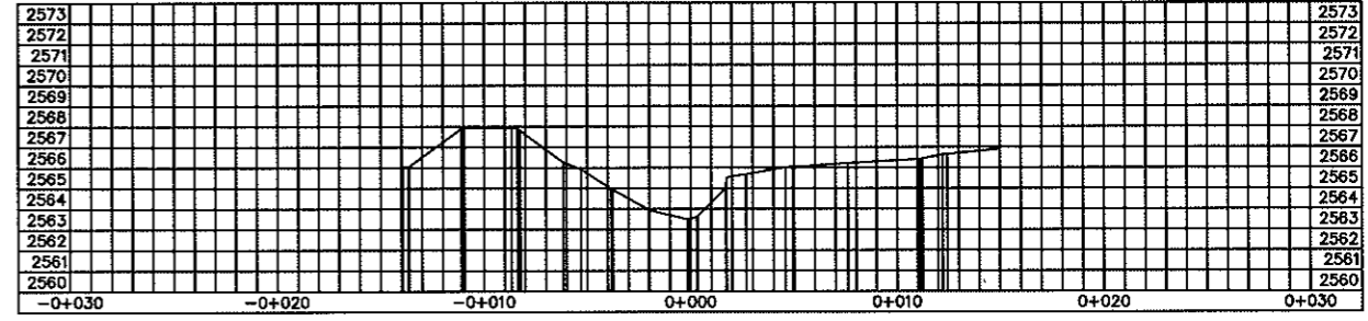
SECCION k0+120
