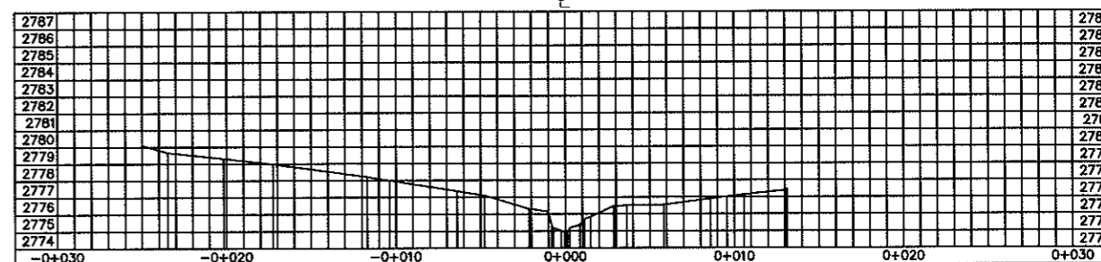
SECCION k0+015
