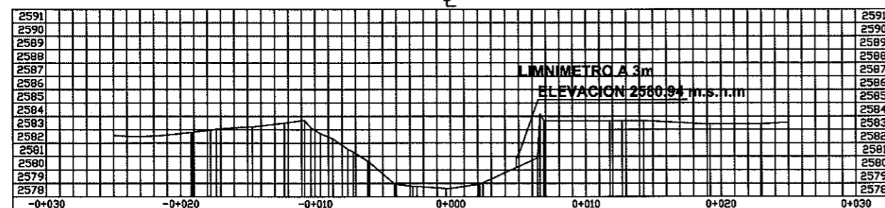
SECCION K0+061.41
