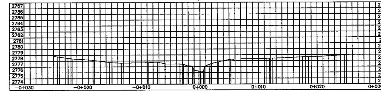
SECCION k0+035
