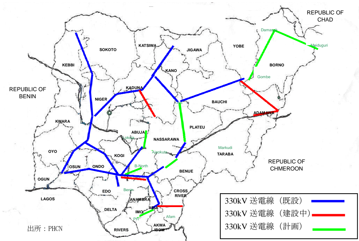
図 3-5 基幹送電線(330kV)の増強計画
