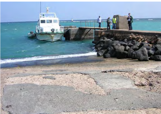
スリップウェイとドルフィン施設
