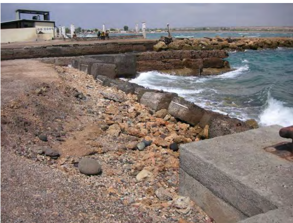
岸壁・護岸の洗堀崩壊状況
